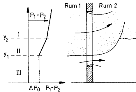
Figur 4.2 Tre olika tryck- och flödesmönster för strömning av brandgas från ett rum till ett annat /4/
