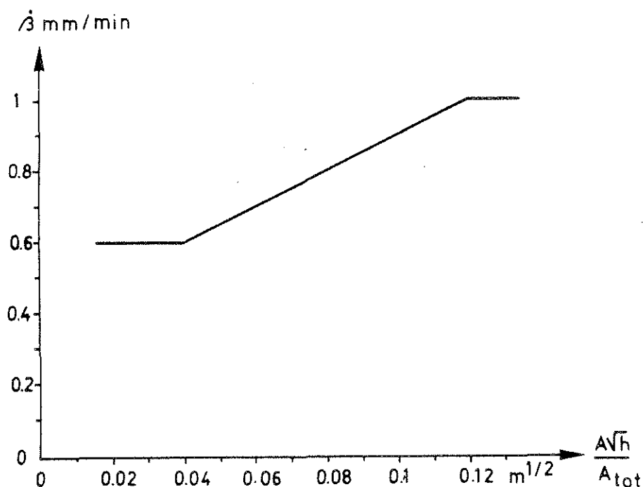
Figur 6.3 Efter enkla överväganden konstruerat närme samband mellan kolskiktets tillväxthastighet \beta för massiv eller laminerad träbalk av gran eller furu och brandcellens öppningsfaktor \frac{A\sqrt{h}}{A_{tot}} /6.1, 6.7, 6.13/
