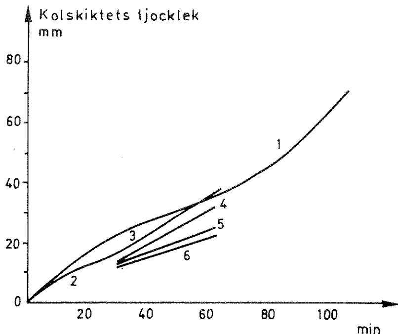
Figur 6.2 Experimentellt bestämt samband mellan kolskiktets tjocklek och varaktigheten för standardbrand. De olika kurvorna ger resultat från engelska, finska och svenska brandprovningar av massiva eller laminerade träbalkar i furu (kurvorna 1, 2 och 3), furu med brandskyddsfärg (kurva 4), ek (kurva 5) och teak (kurva 6) /6.4, 6.5, 6.6/
