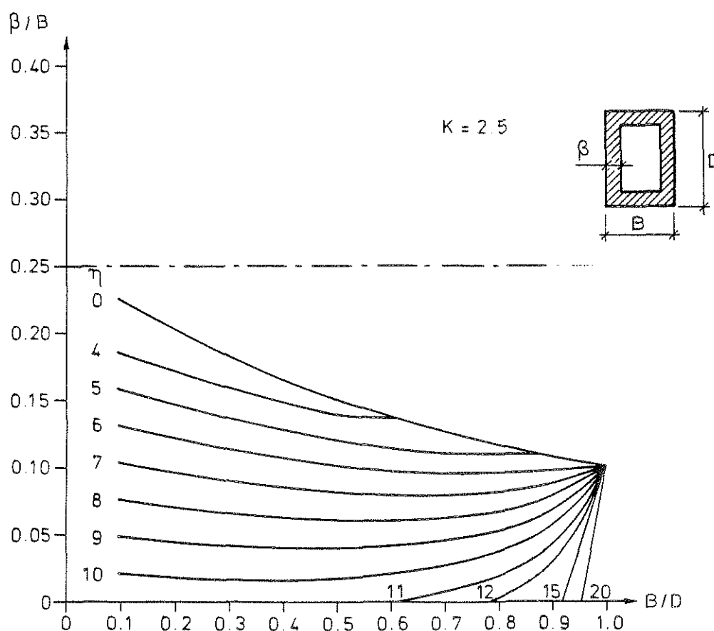
Figur 6.7 Kvoten \beta/B som funktion av breddhöjdförhållandet B/D för fyrsidigt brandangrepp och säkerhetsfaktorn K = 2.5 mot böjbrott före brand vid varierande värden på parametern n /6.12/
