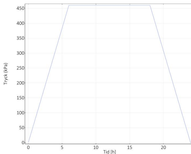
Figur 20 Trycktest av reaktor inneslutning.
