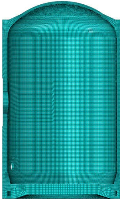
Figur 3 Inneslutningen vid vertikal genomskärning, i nivå med stora genomföringen och kontreforerna.
