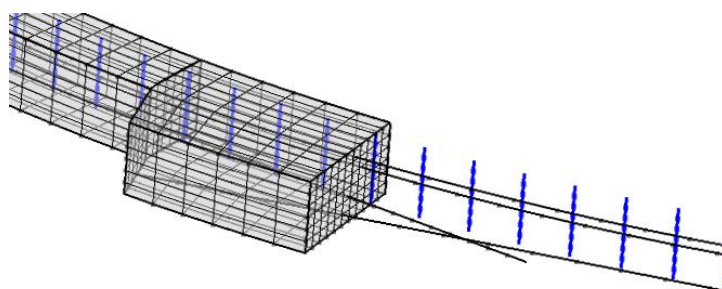
Figur 18 Detalj av elementindelning av spännkablar där de vertikala spännkablar är blåa med nodpunkter markerade och de horisontella spännkablar är svarta med markerade nodpunkter.
