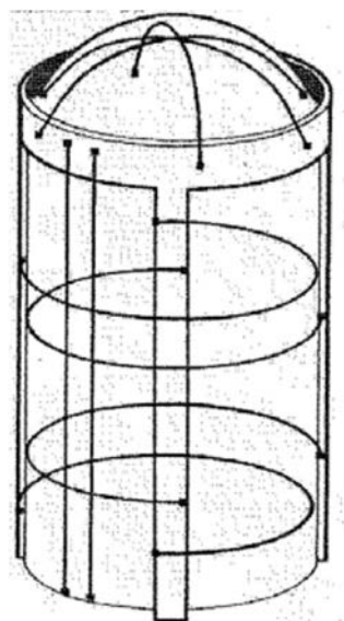
Figur 6 Illustration av anordning av spännkablar i inneslutningen.
