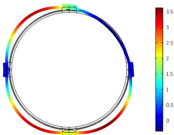
Figur 25 Radiella deformationer när en horisontell spännkabel helt saknar vidhäftning skalan är i millimeter.
