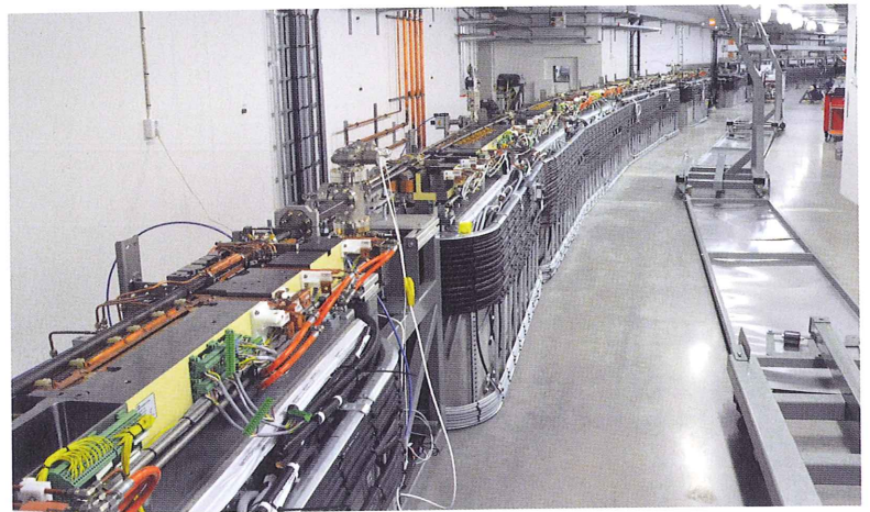
Några magnetsektioner i 3 GeV ringen i MAX IV. Överdelen av magneterna är avlyft och vakuumröret synligt. Foto: Annika Nyberg.
