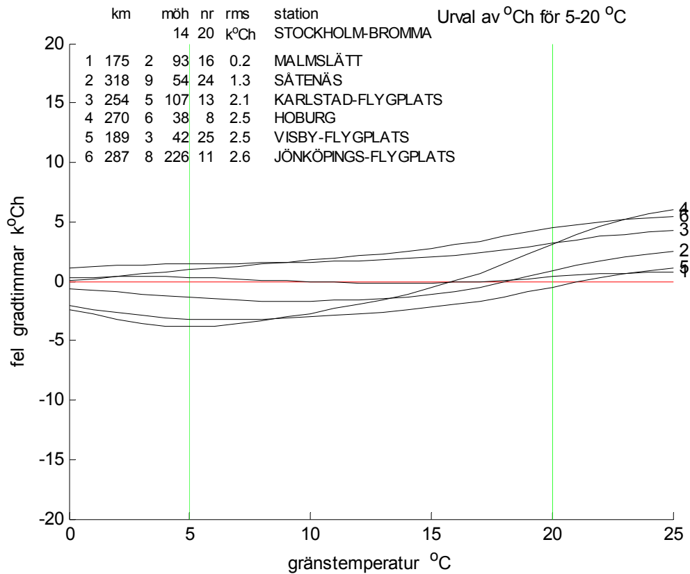
Figur 5.20 Fel i \text{k}^{\circ}\text{Ch} till sex orter som funktion av gränstemperaturen med urval 5-20 ^{\circ}\text{C} .
