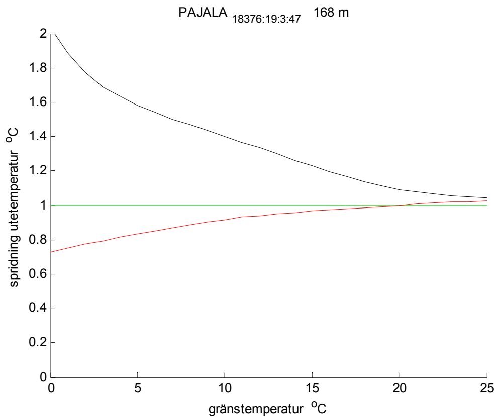
Figur 4.38 Spridning i utetemperatur beräknad med gradtimmar och drifttid eller 8760 h.
