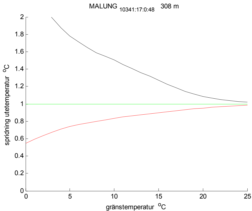
Figur 4.34 Spridning i utetemperatur beräknad med gradtimmar och drifttid eller 8760 h.
