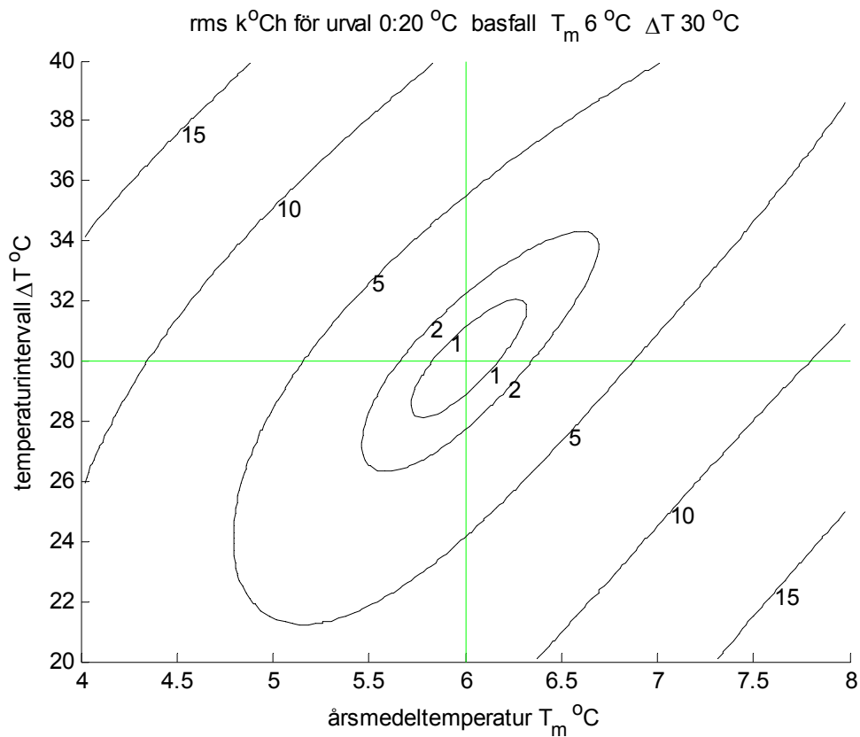
Figur 4.56 Felkänslighet k^{\circ}Ch för urval 0:20 °C för förenklad °Ch-funktion.
