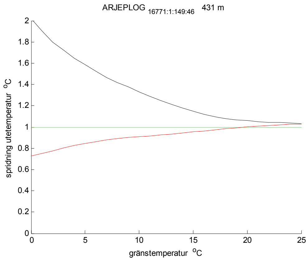
Figur 4.2 Spridning i utetemperatur beräknad med gradtimmar och drifttid eller 8760 h.
