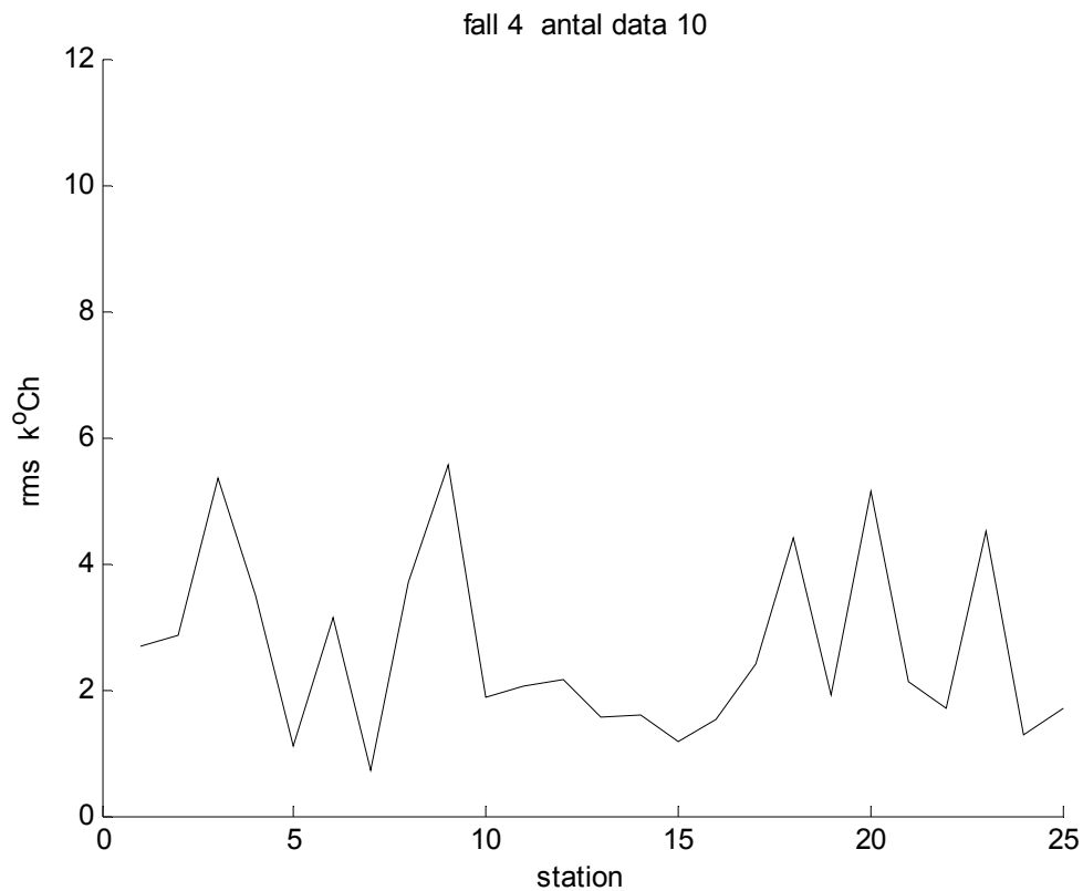
Figur 5.30 Rms k^{\circ}Ch för fall 4, antal data 10, urval 0-25 °C och olika stationer.
