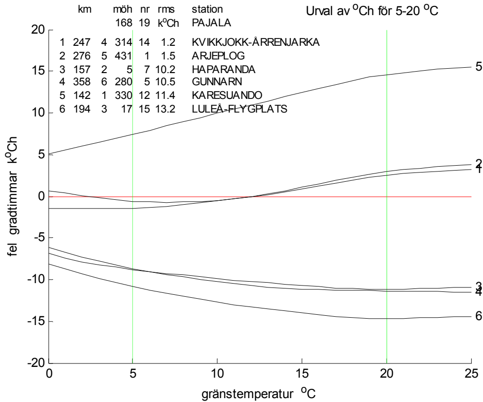
Figur 5.19 Fel i \text{k}^{\circ}\text{Ch} till sex orter som funktion av gränstemperaturen med urval 5-20 ^{\circ}\text{C} .
