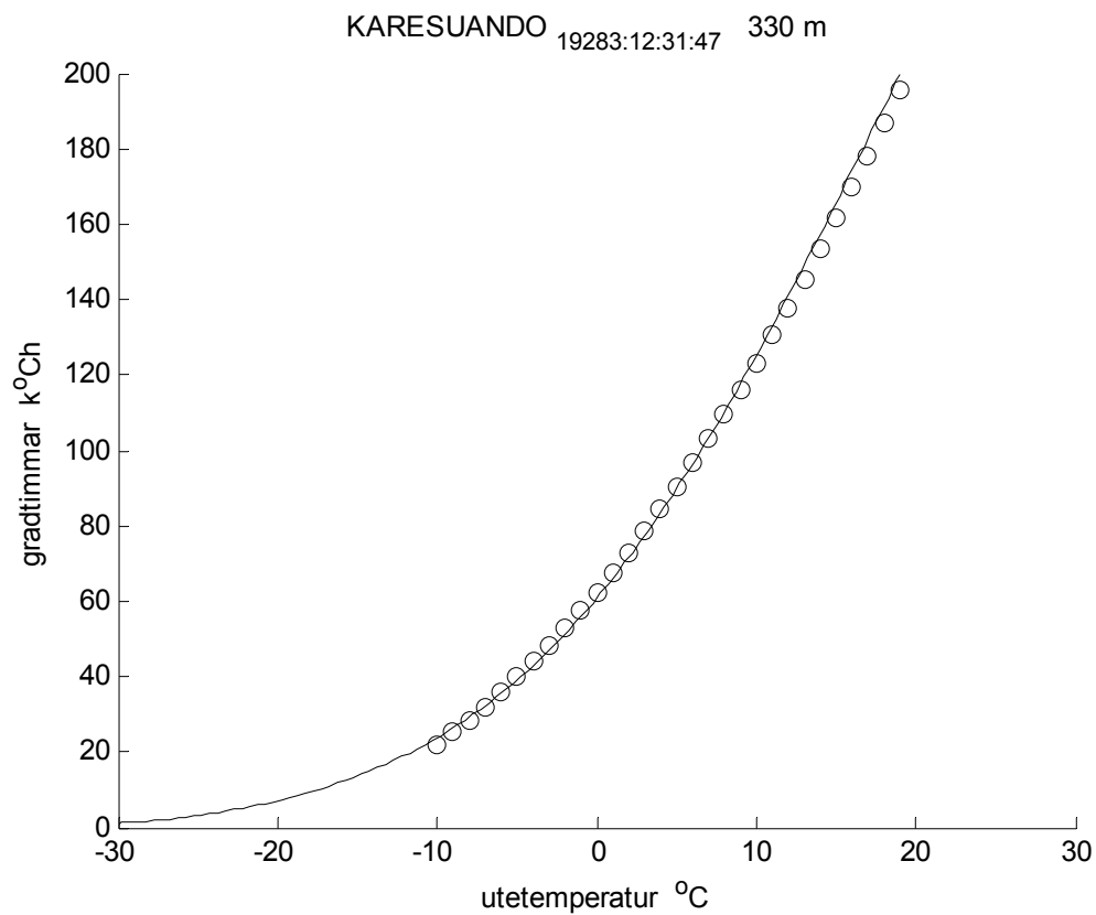
Figur 4.60 Uppmätt och förenklad °Ch-funktion för utetemperaturen för Karesuando.
