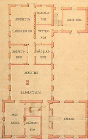
1 re VÅNINGEN
