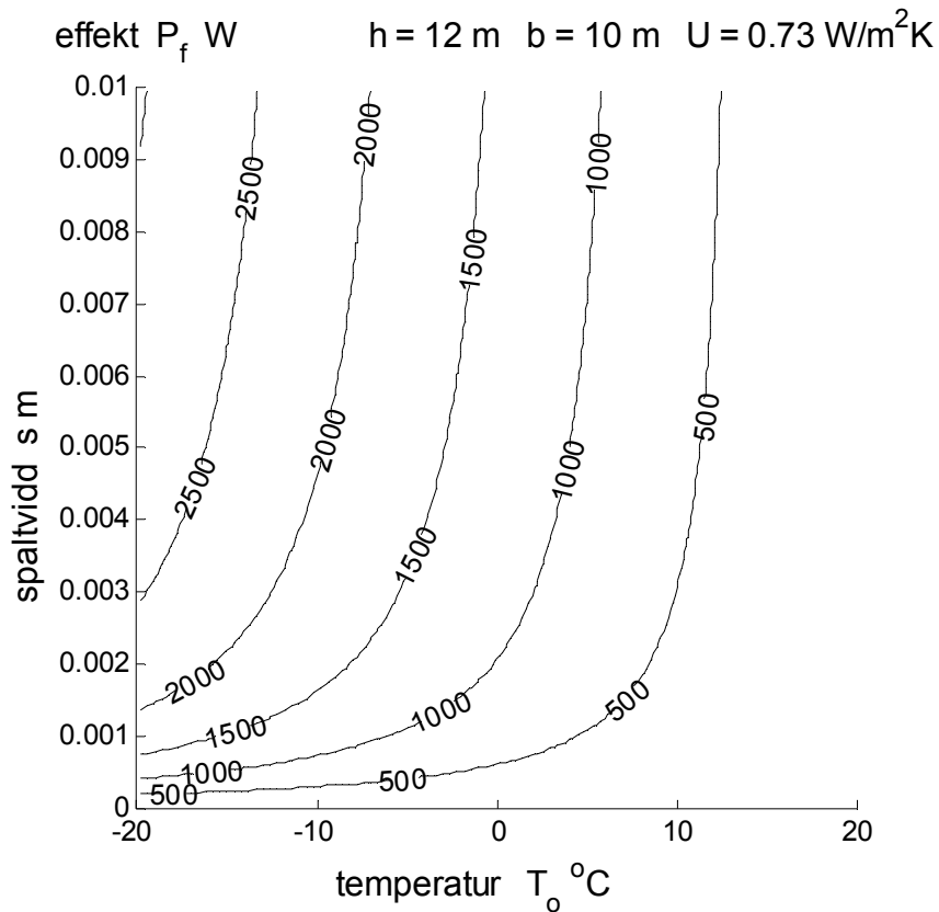
Figur 4.2 Isodiagram för värmeförlust P_f \text{ W} med axlarna utetemperatur och spaltvidd.
