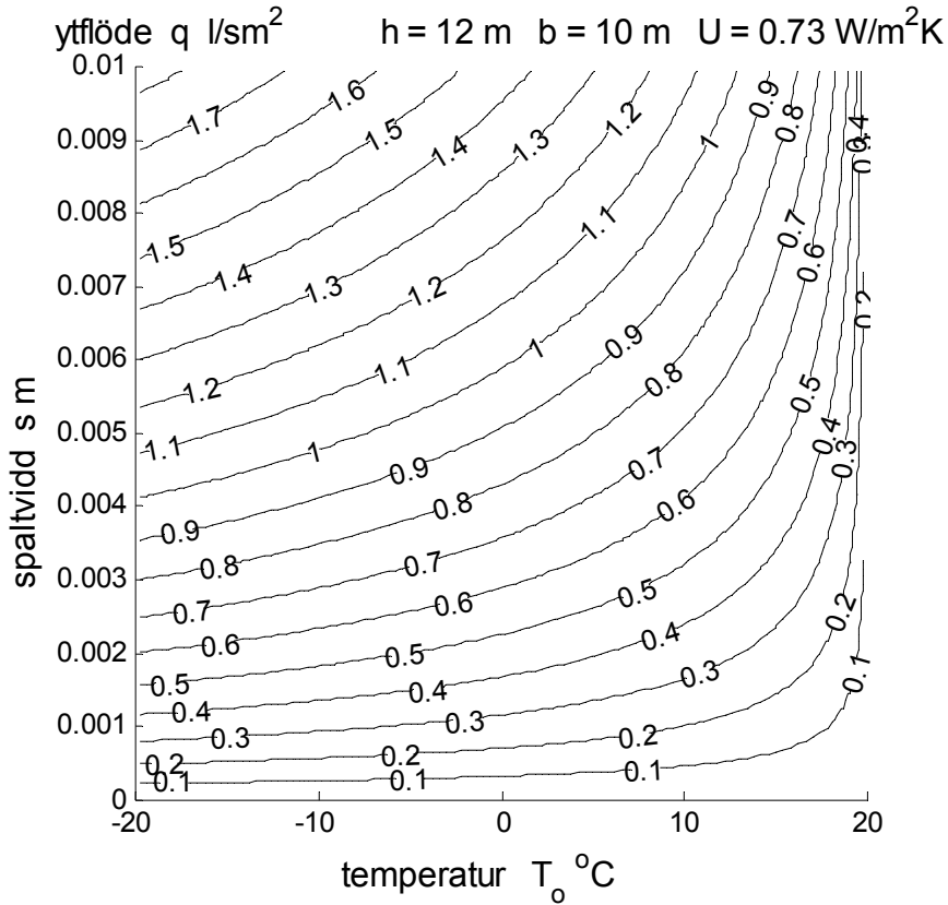
Figur 4.7 Isodiagram för ytlöde q l/sm 2 med axlarna utetemperatur och spaltvidd.
