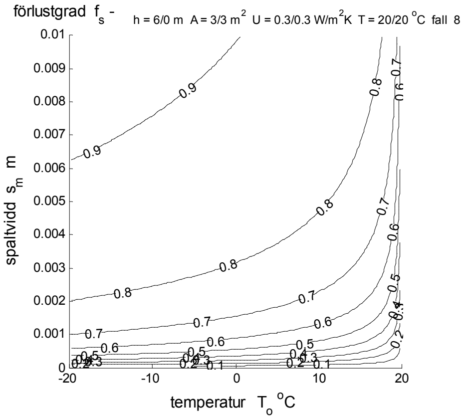
Figur 2.19 Isodiagram för förlustgrad f - med axlarna utetemperatur och spaltvidd för fall 8.
