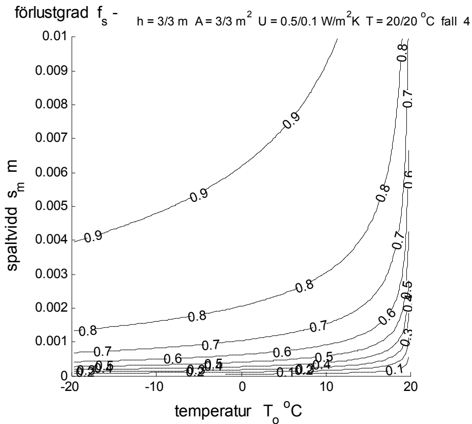
Figur 2.11 Isodiagram för förlustgrad f - med axlarna utetemperatur och spaltvidd för fall 4.
