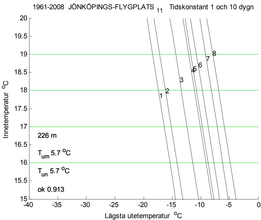
Figur 3.2 Innetemperatur för lägsta utetemperatur för given varaktighet och tidskonstant.
