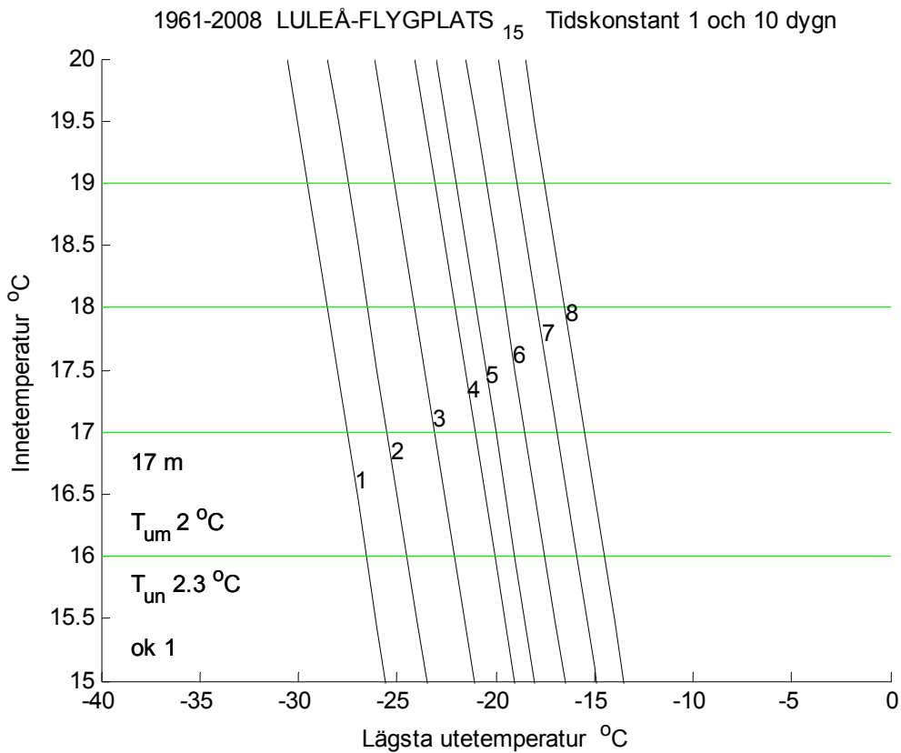
Figur 3.6 Innetemperatur för lägsta utetemperatur för given varaktighet och tidskonstant.
