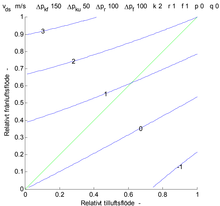
Figur 5.4 Lufthastighet i renblåsning mellan avluft och uteluft för \Delta p_k \Delta p_r 1.0.
