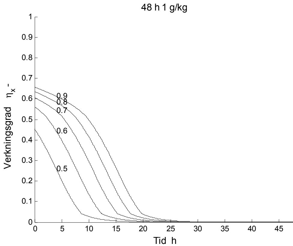
Figur 14.8 Fuktverkningsgrad \eta_x -för som funktion av tiden 0-48 h för fall 4.
