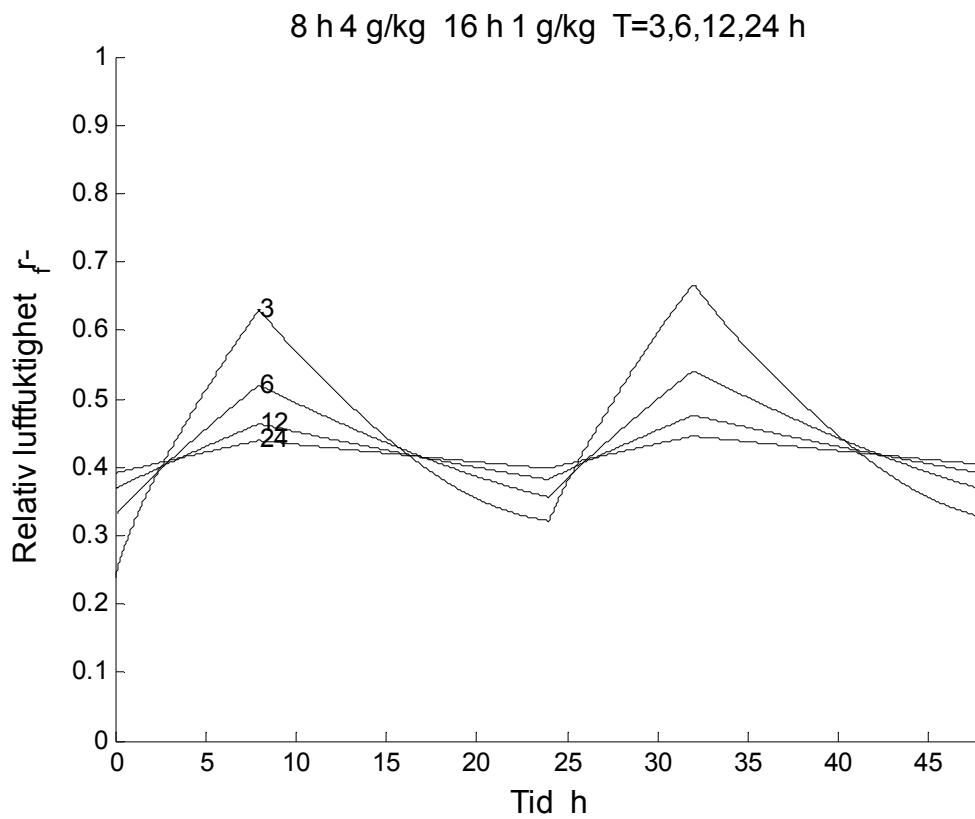
Figur 14.13 Relativ luftfuktighet r_f - som funktion av tiden 0-48 h för fall 7.
