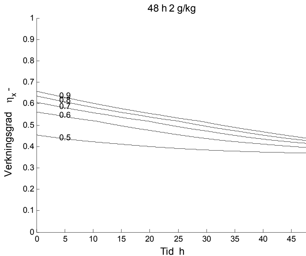
Figur 14.10 Fuktverkningsgrad \eta_x -för som funktion av tiden 0-48 h för fall 5.
