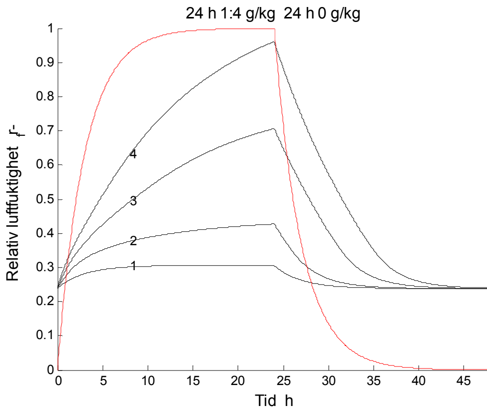
Figur 14.1 Relativ luftfuktighet r_f - som funktion av tiden 0-48 h för fall 1.
