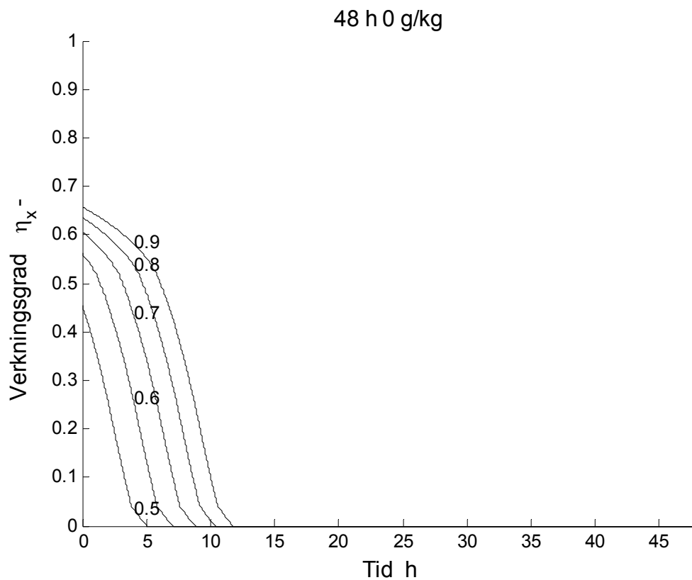
Figur 14.6 Fuktverkningsgrad \eta_x -för som funktion av tiden 0-48 h för fall 3.
