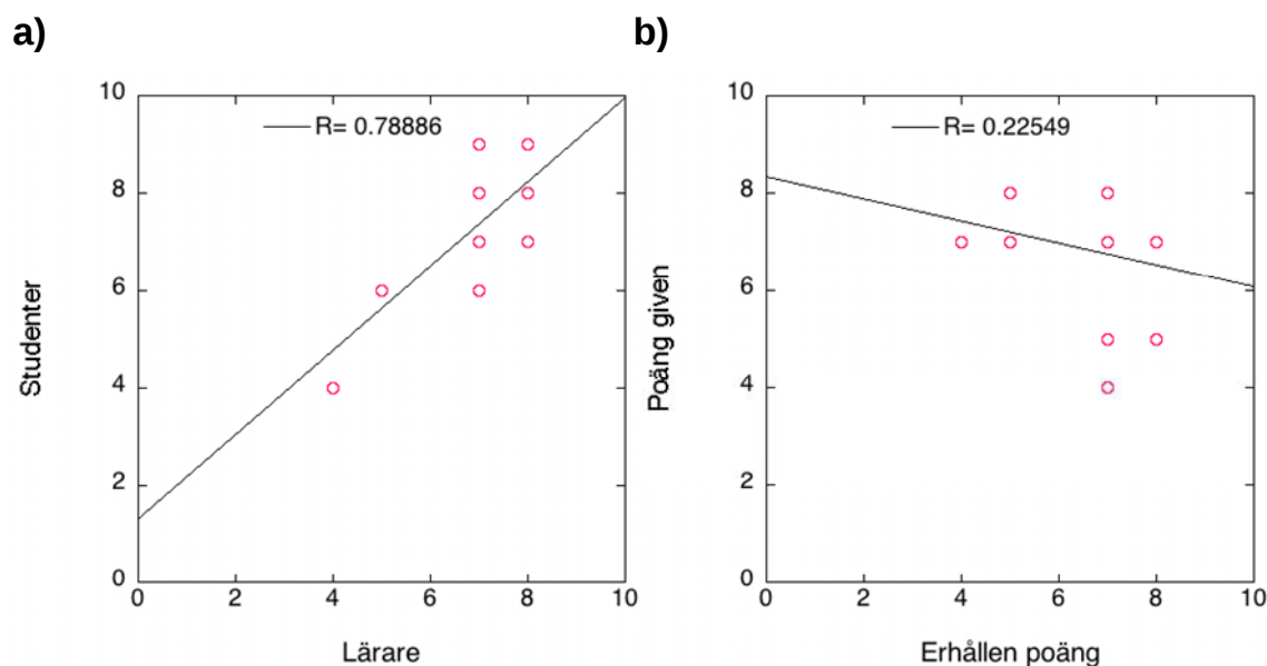
Figur 3. a) Korrelation mellan lärargrups och studentgrupps totalpoäng. b) Avsaknad av korrelation mellan totalpoäng som studentgrupp erhöll och den totalpoäng de gav som opponenter.
