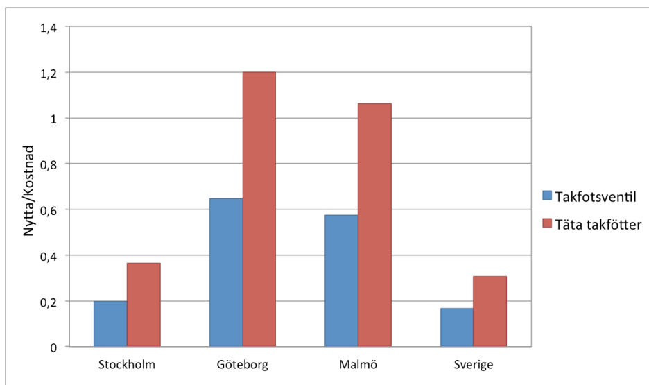
Figur 11: Skydd av takfot för referensfall 2.
