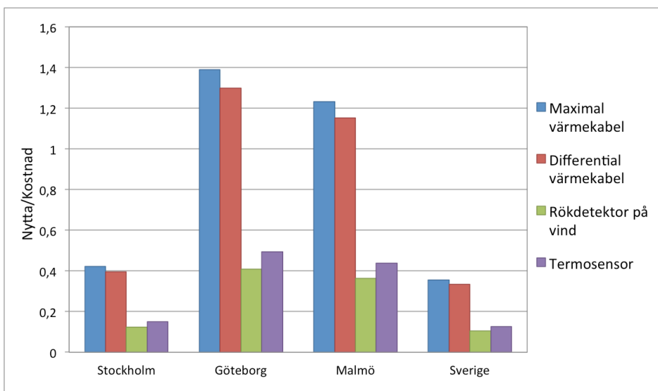
Figur 14: Utvändiga detektionssystem i referensfall 2 med 15 års livslängd.
