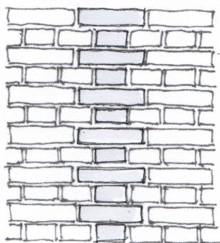
Blockförband, renässansförband
