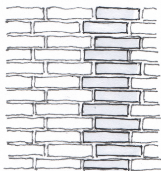
Löpförband med 1/4 stens växlande förskjutning
