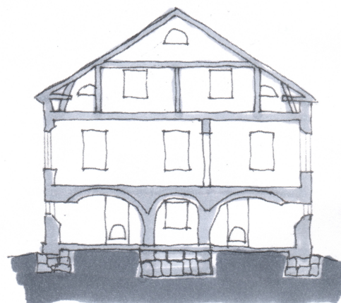
Sektion, tvärsnitt
