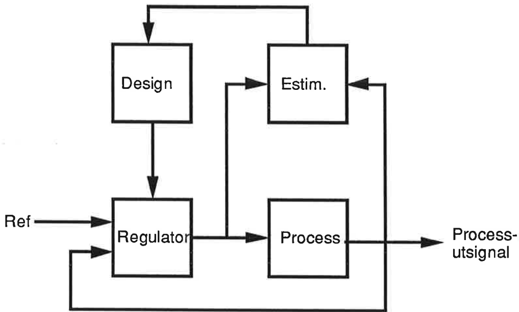
Fig 1 Principskiss, STR
