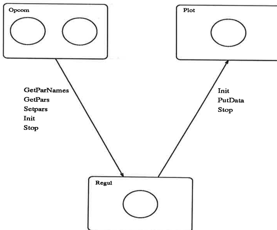
Figur 2: Ingående moduler
