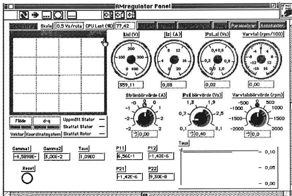
Figur 4: Vår frontpanel.
