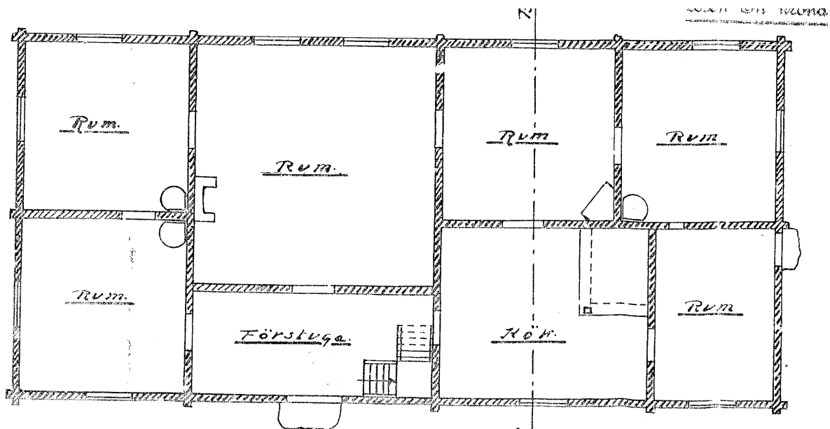
Fig. 21. Planlösning över Västra Vrams prästgård i skala 1:100, Kulturhistoriska museet i
