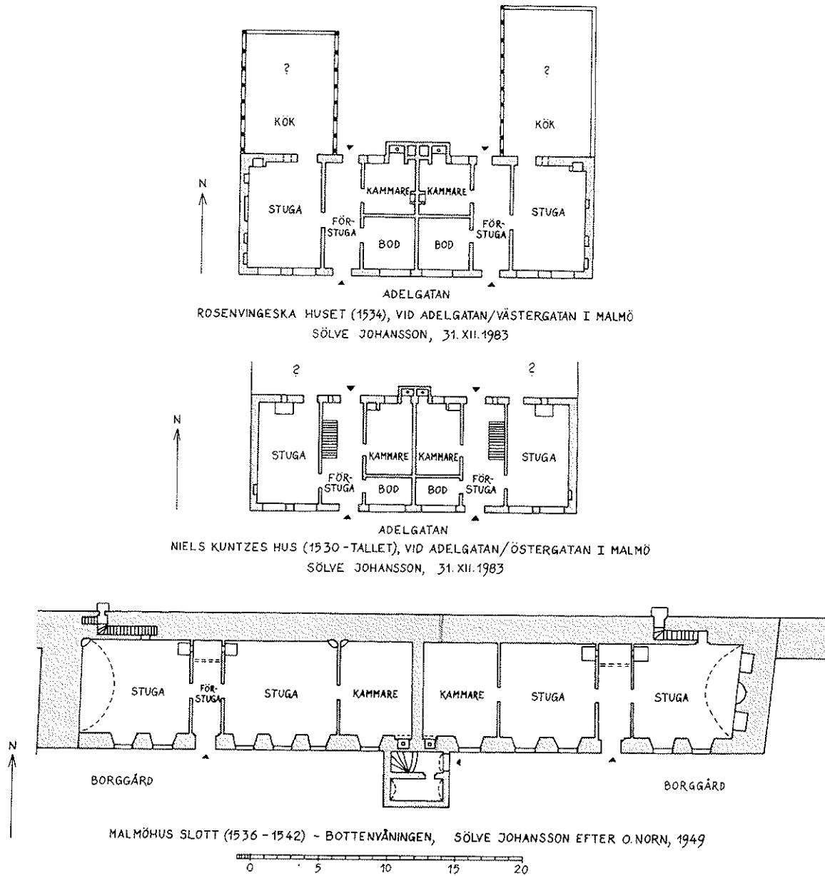
Fig. 19. 3 Planlösningar över Liljefeldska, Malmöhus och Kuntzes hus (Johansson 1987:58)
