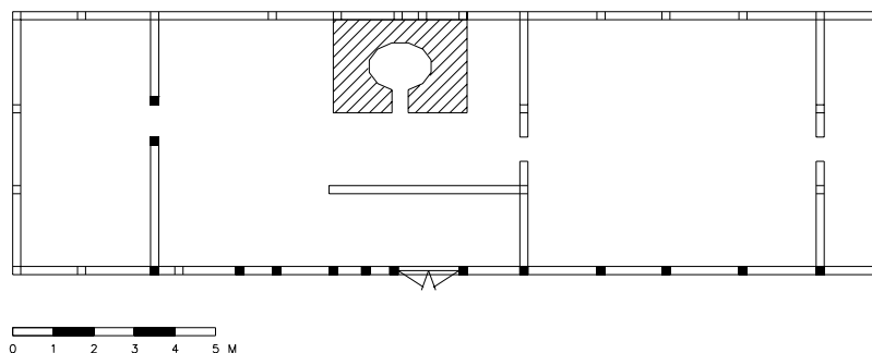
Fig. 8. Rekonstruktion på Wowragårdens planlösning i skala 1:200, efter underlag ifrån Eriksdotters byggnadsarkeologiska undersökning.
