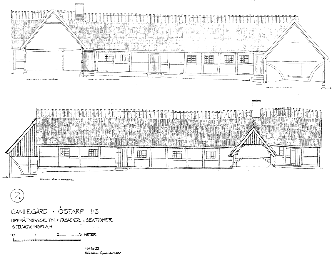
Fig. 10. Fasadritningar av bostadshuset på Östarps Gamlegård, av Rebecka Gunnarsson.
