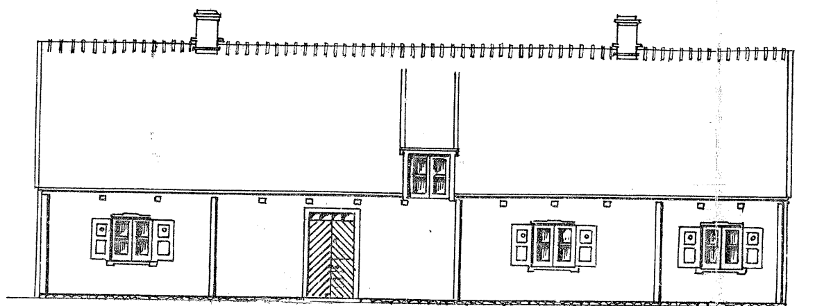
Fig. 20. Fasadritning av Västra Vrams prästgård i skala 1:100, Kulturhistoriska museet i Lund
