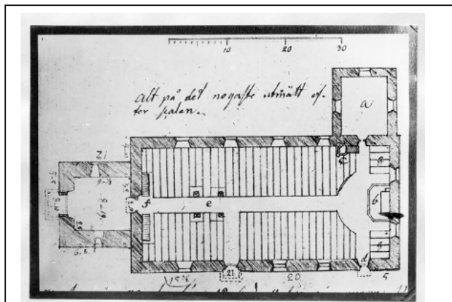
Bild 13 Plan över kyrkan, förmodligen ritad 1819 av Nils Isak Löfgren. Ur VOUP
