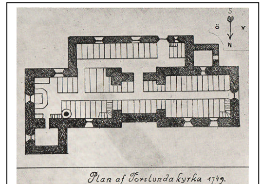
Bild 12 Plan över kyrkan med "nykyrkan" högst upp i bild (norr är nedåt). Teckning av Petrus Frigelius 1749. Ur Svennebring, 1976, sid. 14
