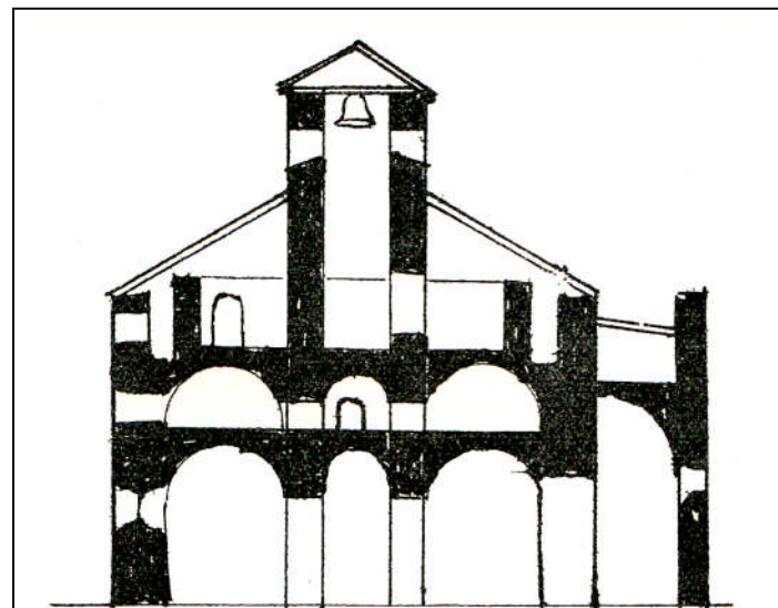
Bild 7 Rekonstruktion av äldsta kyrkan, genomskärning Ö-V Ur Karlsson, 1935, sid. 12
