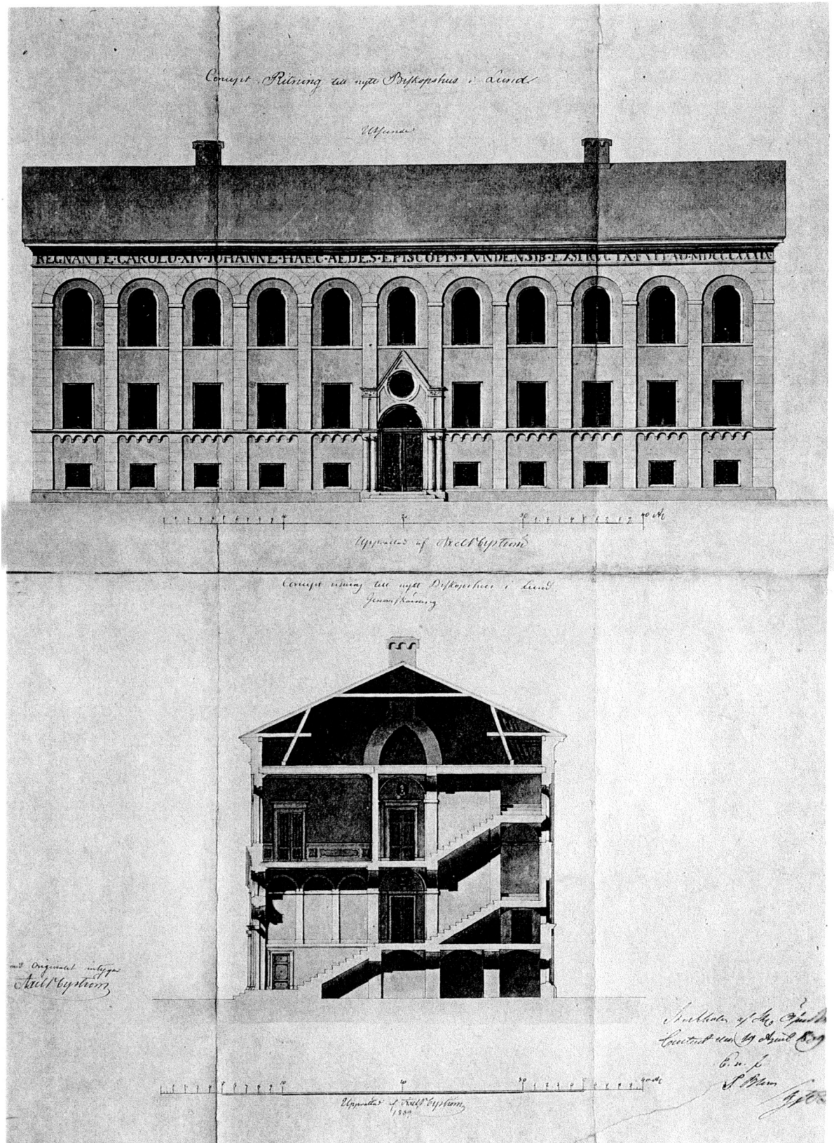
Ritning till nytt biskopshus i Lund, Axel Nyström. 1839. [Kulturens arkiv, Lund]
