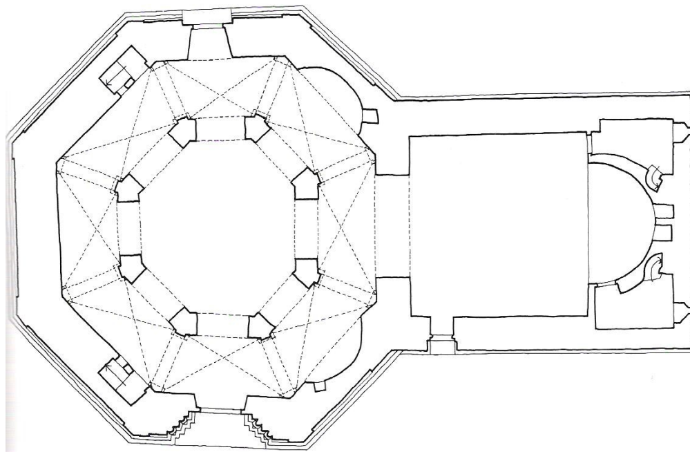
Fig 4. Planlösning för Helgeands i Visby (skala, 1:200).
