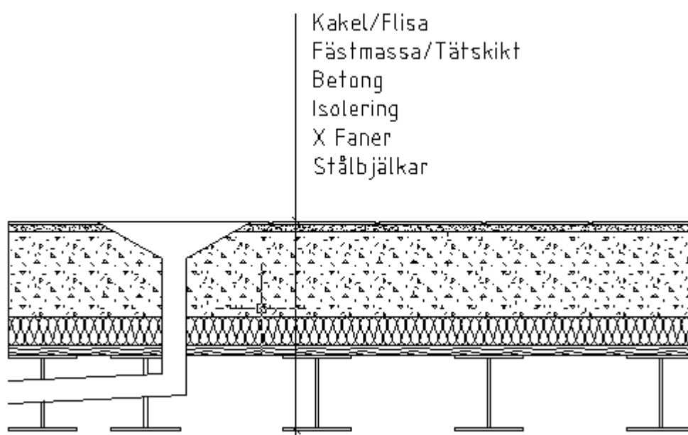
Figur 7. Golvkonstruktion med X faner.
