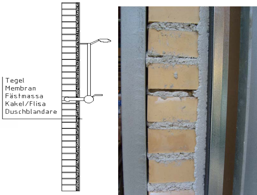
Figur 10. Tegelmurad vägg
