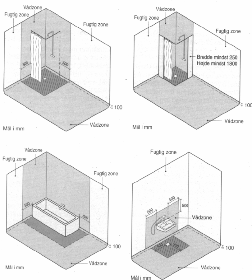
Figur 1. Våtrumsindelning enligt danska By og Byg Anvisning 200
