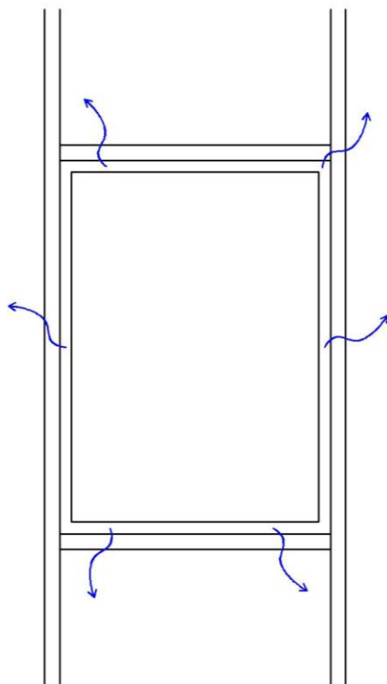
Figur 27 Spallläckage runt vindslucka
