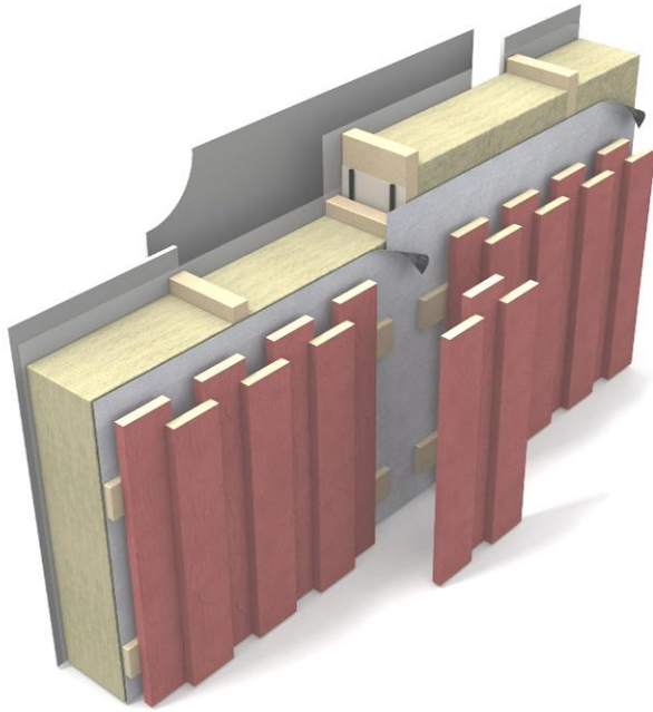
Figur 32 Anslutning mellan två prefabricerade träregelement (Paroc, 2010).
