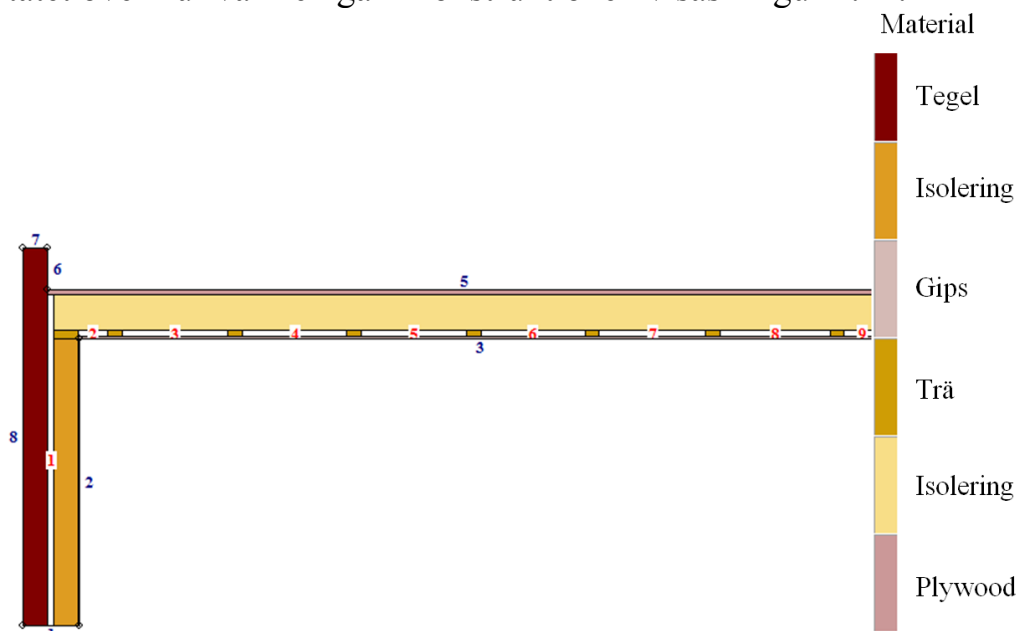
Figur 4.10 Anslutningen mellan taket och ytterväggen
