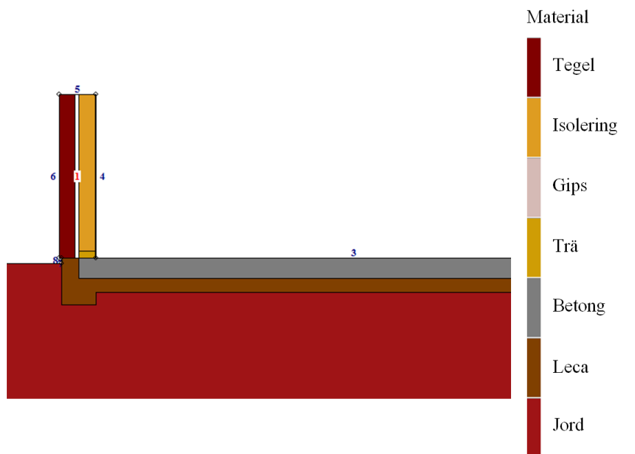
Figur 4.8 Anslutning yttervägg – grund
