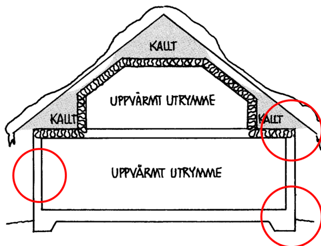
Figur 3.7 Köldbryggorna är störst där konstruktionsdelar möts av H Bülow-Hübe.
