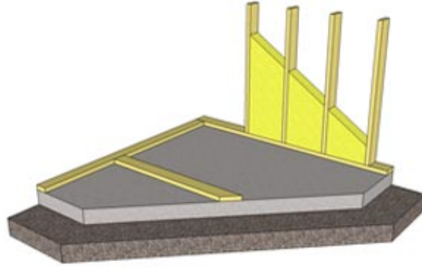
Figur 3.18 Tryckimpregnerad träsyll rakt mot betongen [35].
