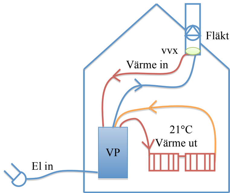
Figur 3.12 Principskiss av ett frånluftssystem med värmeåtervinning av H Bülow-Hübe.
