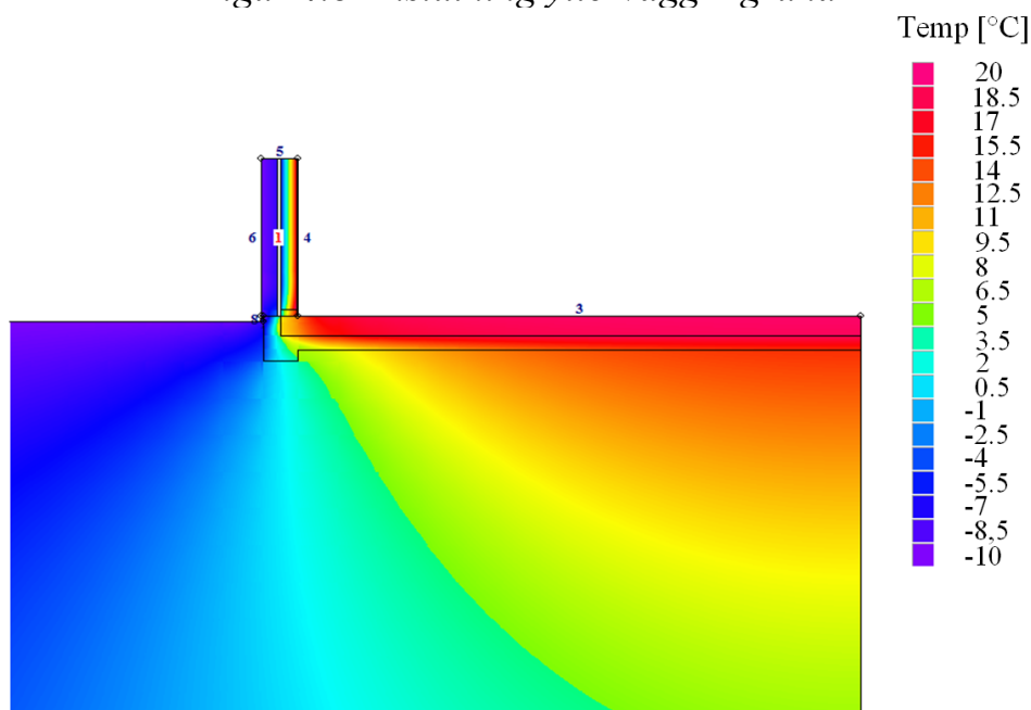
Figur 4.9 Värmefflöde anslutning yttervägg – grund
