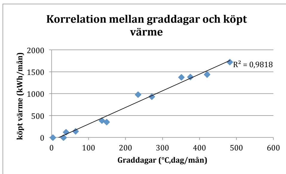
Diagram 8.1 Korrelation mellan graddagar och uppskattad köpt värme
