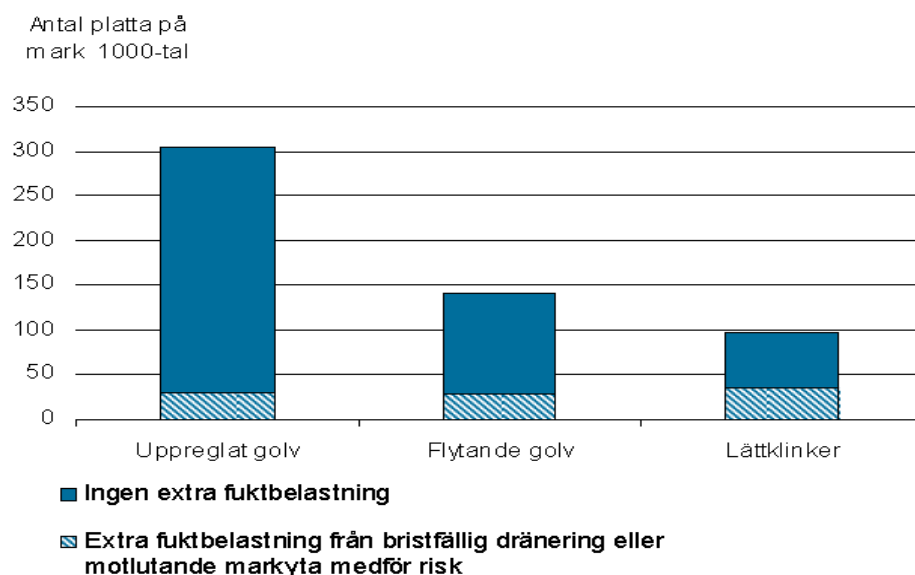
Diagram 2.3 Olika typer av platta på mark konstruktioner och antalet av dem som har risk för fuktskada, med eller utan extra fuktbelastning [13].
