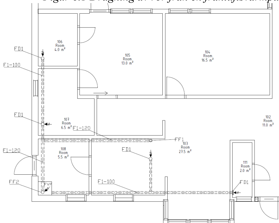
Figur 6.2 Dragning av rör från en frånluftsvärmpump.
