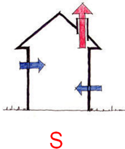
Figur 3.9 Principskiss av ett självdregssystem [25].
