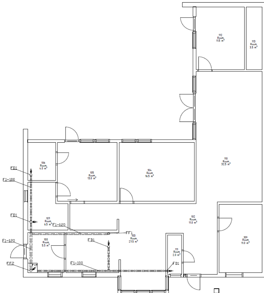
Figur 6.1 Dragning av rör från en frånluftsvärmpump.
