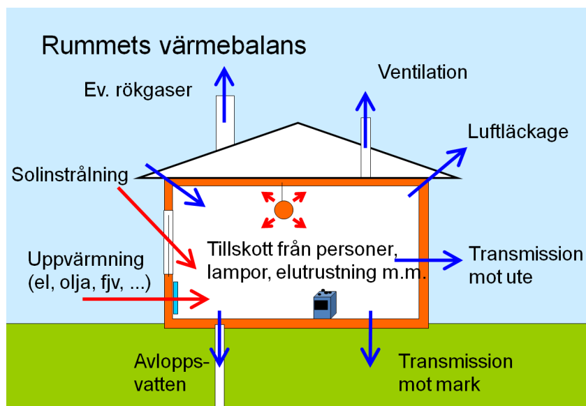
Figur 3.1 Rummets värmebalans av H Bülow-Hübe / P Wallentén.
