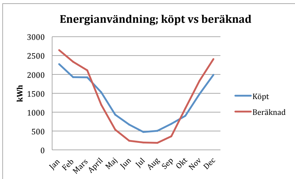
Diagram 8.2 Samband mellan köpt och beräknad energianvändning.
