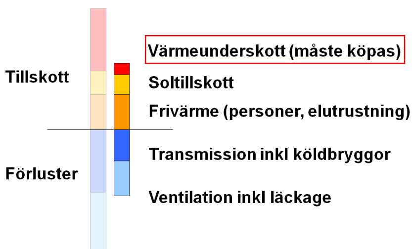
Figur 3.2 Husets värmebalans av H Bülow-Hübe.
