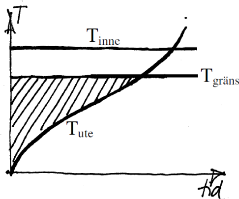
Figur 3.4 Det randiga området visar gradtimmarna för uppvärmning [18].
