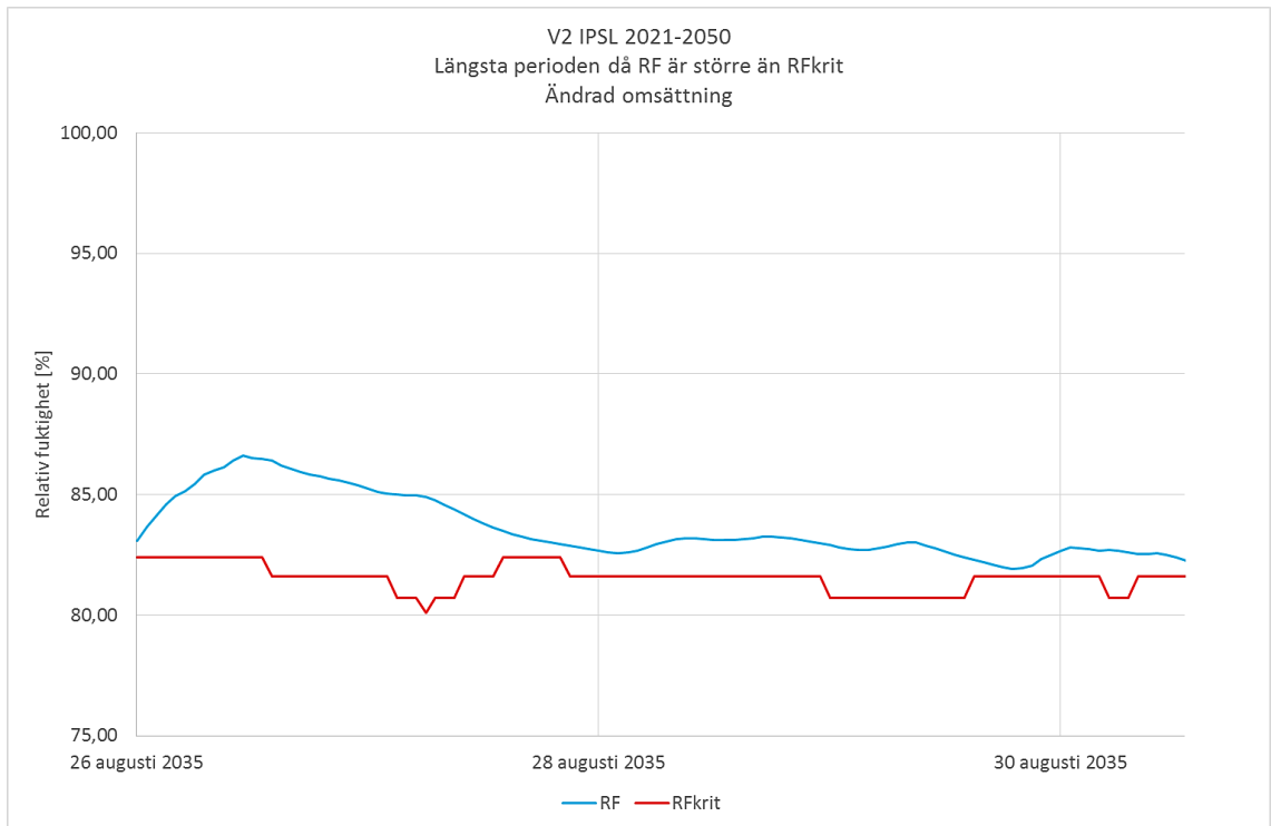
Figur 7.11 Längsta perioden då RF överskrider RF_{krit} är 4 dygn och 14 timmar.
