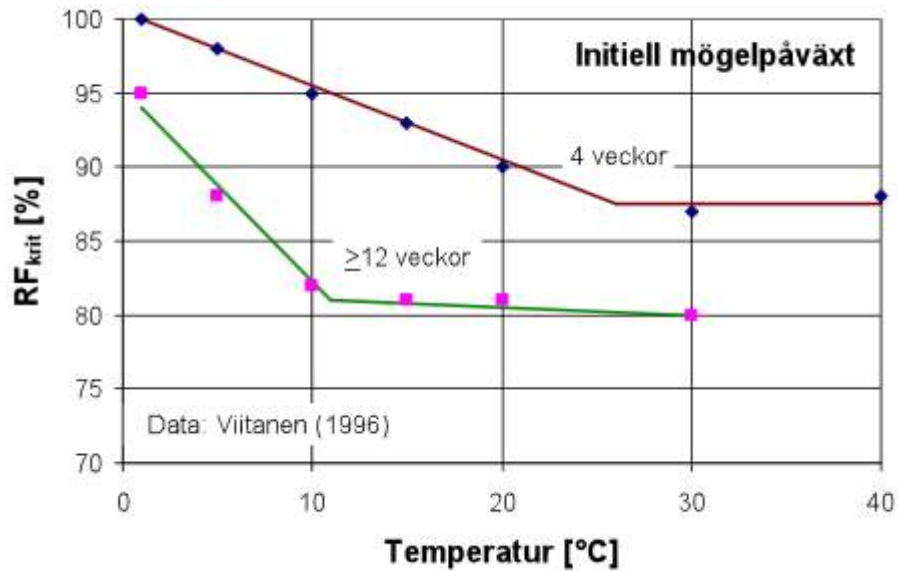
Figur 2.2 Kritiskt fuktillstånd för "initial" mögelpåväxt på trä vid olika temperaturnivåer och varaktigheter (Nilsson L-O, 2009).
