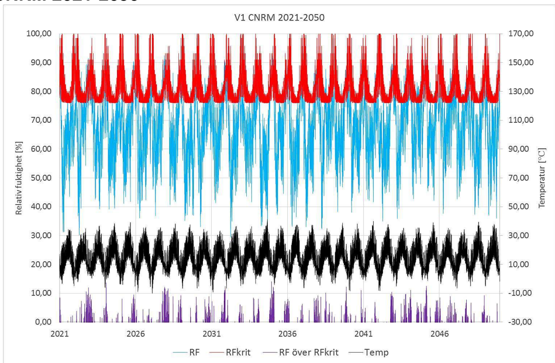
Figur 14.13 Folos-diagram för V1 CNRM 2021-2050.
