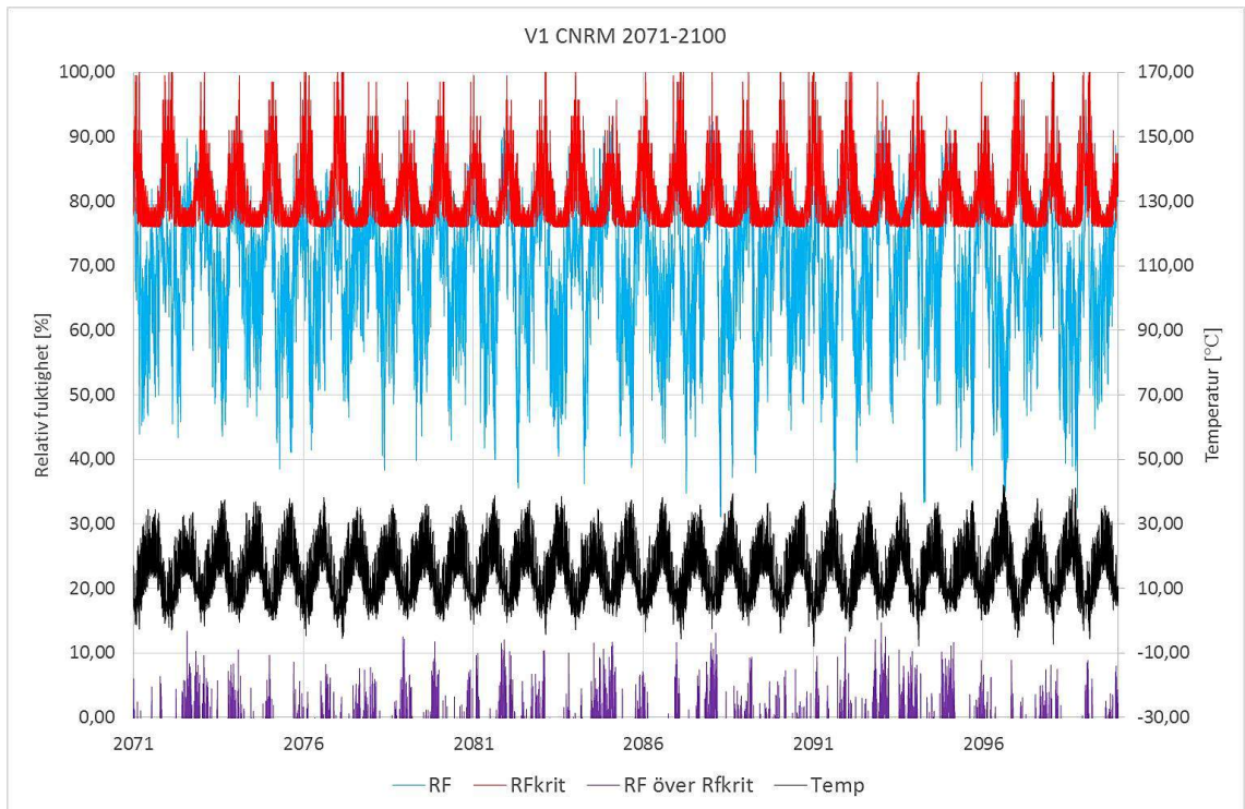
Figur 14.25 Folos-diagram för V1 CNRM 2071-2100.
