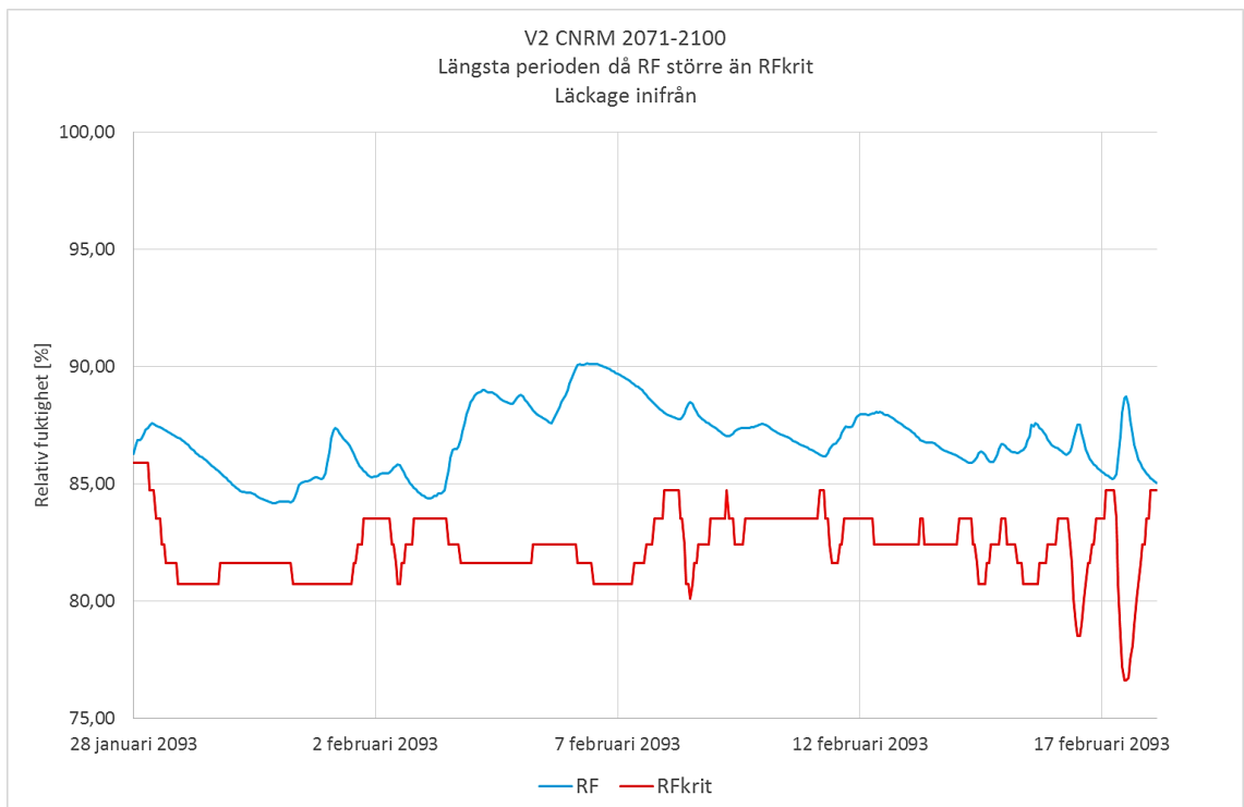
Diagram 6.9 Längsta perioden då RF överstiger RF_{krit} är 21 dygn och 4 timmar.
