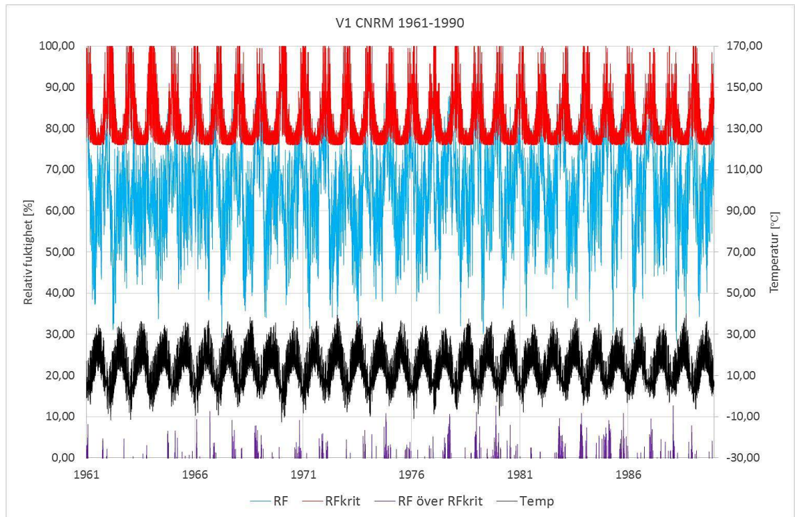
Figur 14.1 Folos-diagram för V1 CNRM 1961-1990.
