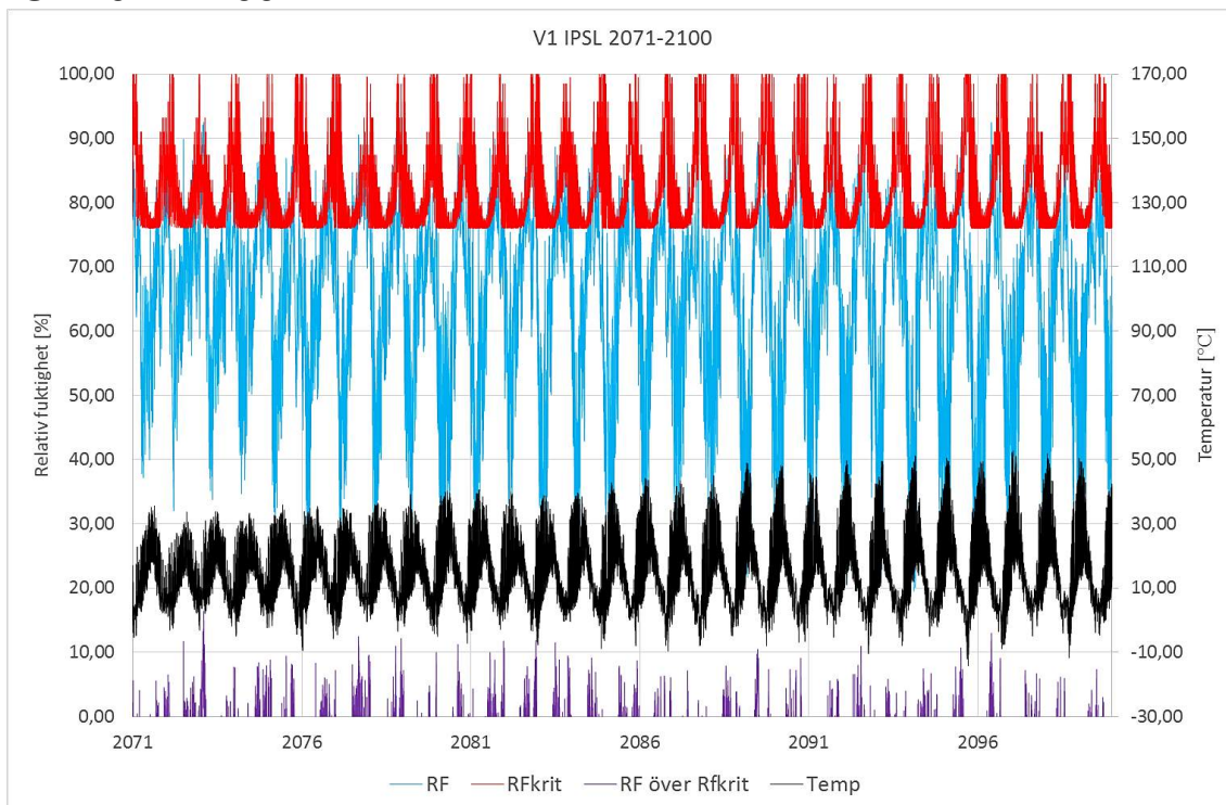
Figur 14.28 Folos-diagram för V1 IPSL 2071-2100.
