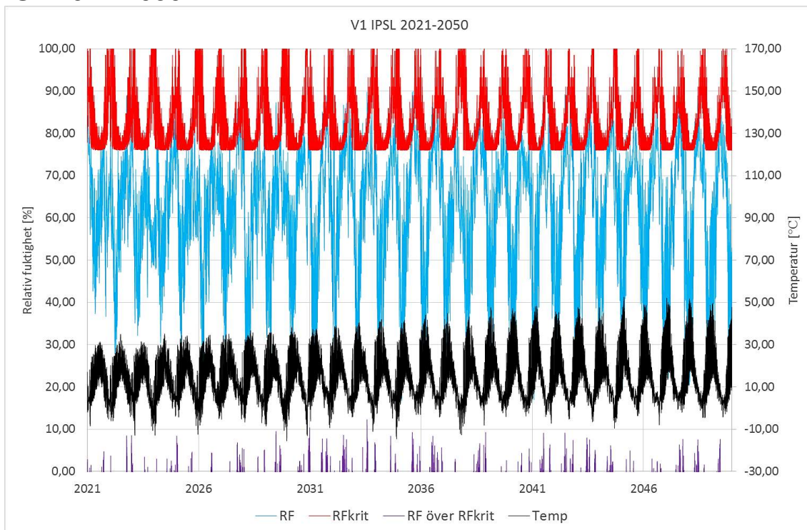
Figur 14.16 Folos-diagram för V1 IPSL 2021-2050.
