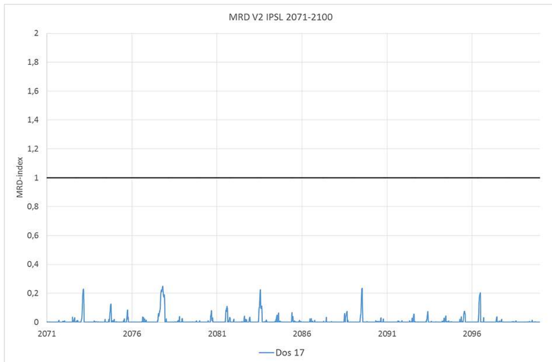
Figur 10.6 MRD-index (0-2) för V2 basfall.
