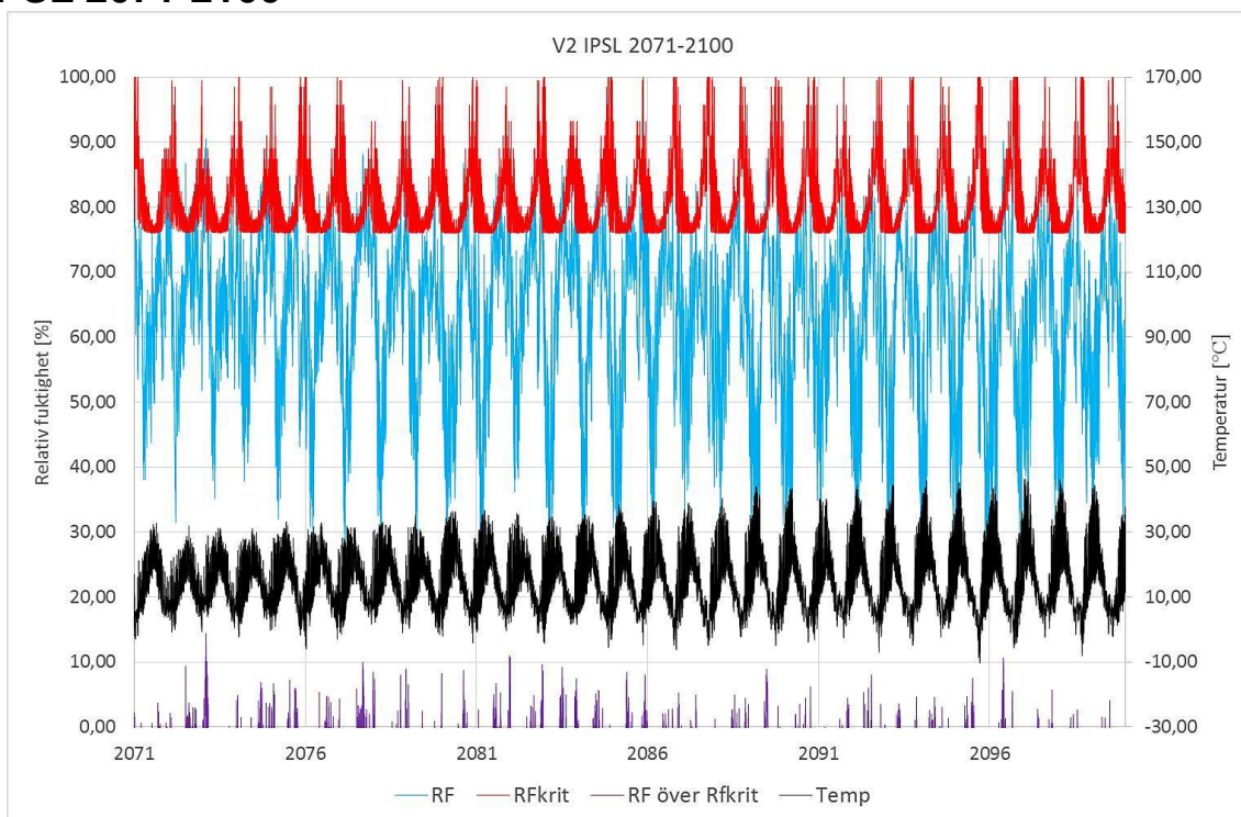
Figur 14.34 Folos-diagram för V2 IPSL 2071-2100.
