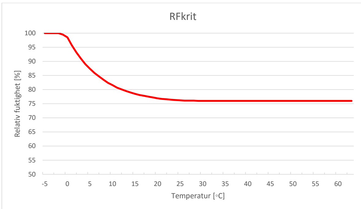
Figur 2.1 Kritisk fuktighet vid varierande temperatur. (Zedlbauer K, 2001)
