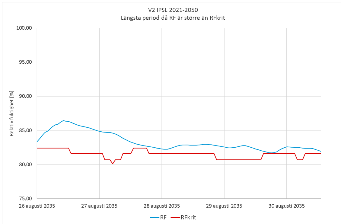
Figur 14.23 Längsta perioden då RF överskrider RF_{krit} är 4 dygn och 14 timmar.
