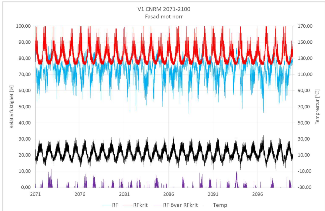
Figur 9.1 Folos-diagram för V1 CNRM 2071-2100 där fasaden är vänd mot norr.
