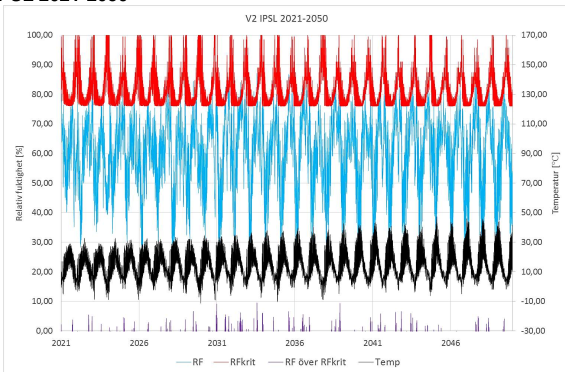
Figur 14.22 Fols-diagram för V2 IPSL 2021-2050.
