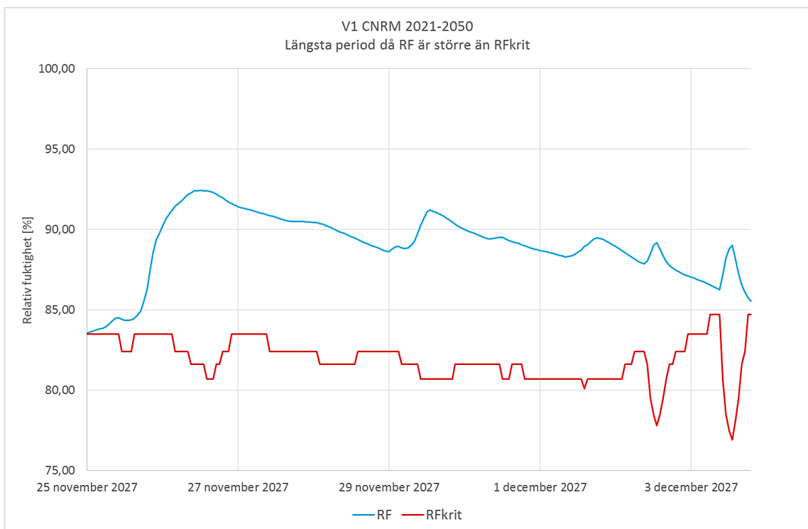
Figur 14.14 Längsta perioden då RF överskrider RF_{krit} är 8 dygn och 20 timmar.
