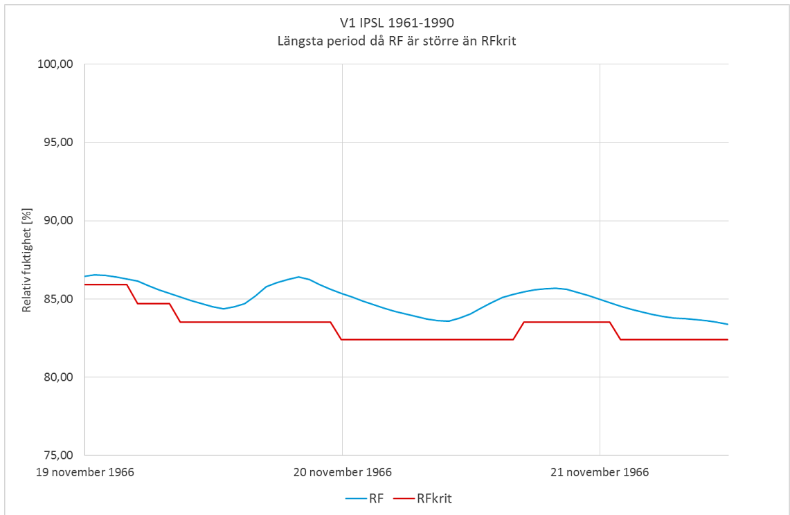
Figur 14.5 Längsta period då RF överstiger RF_{krit} är 2 dygn och 13 timmar.
