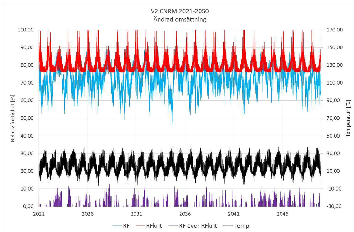
Figur 7.7 Folos-diagram för V2 CNRM 2021-2050.
