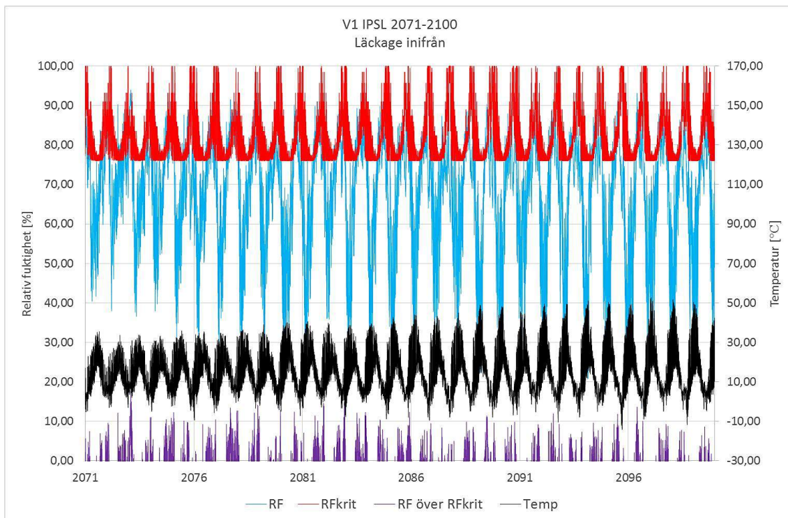
Figur 6.5 Folos-diagram för V1 IPSL 2071-2100.
