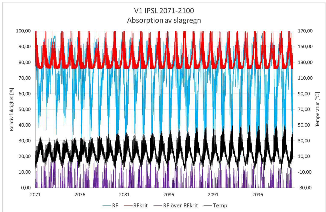
Figur 8.4 Folos-diagram för V1 IPSL 2071-2100.
