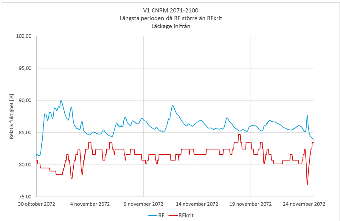
Figur 6.3 Längsta perioden som RF överskrider RF_{krit} är 25 dygn och 22 timmar.
