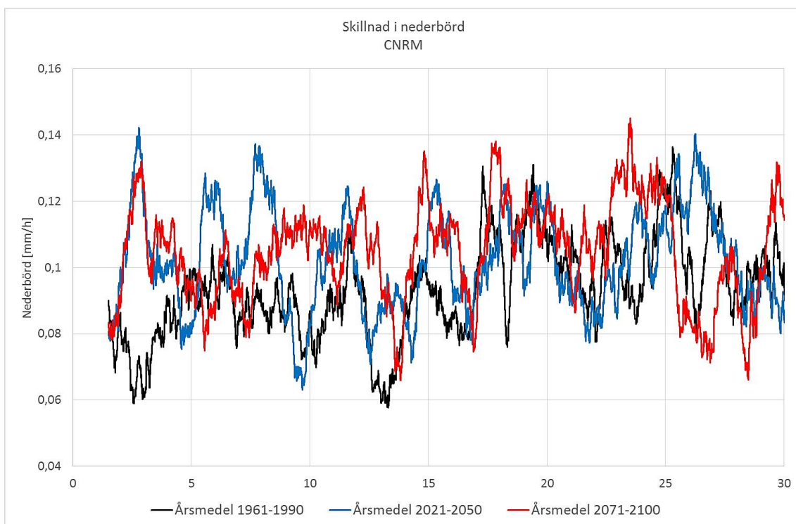
Figur 3.3 Skillnad i årsmedelnederbörd för klimatfil CNRM.
