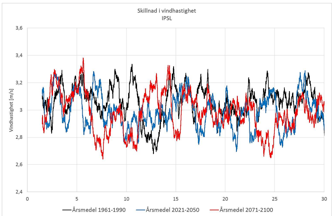
Figur 3.8 Skillnad i årsmedel, vindhastighet, för klimatfil IPSL.
