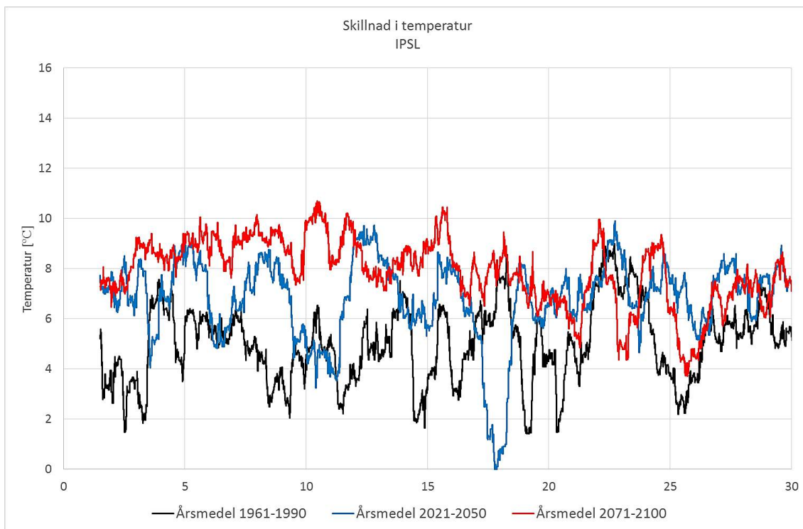
Figur 3.2 Skillnad i årsmedeltemperatur för klimatfil IPSL.
