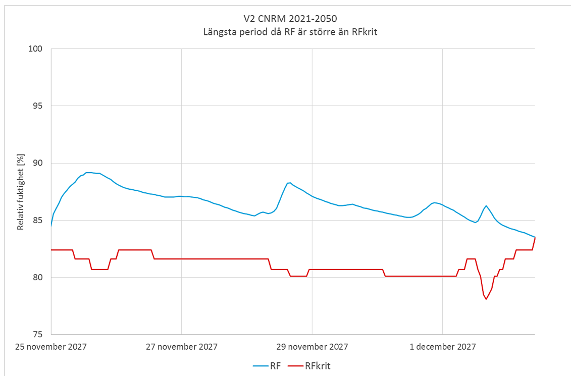
Figur 14.20 Längsta perioden då RF överskrider RF_{krit} är 7 dygn och 11 timmar.
