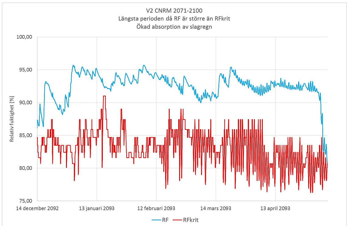
Figur 8.8 Längsta perioden då RF överskrider RF_{krit} är 146 dygn och 8 timmar.
