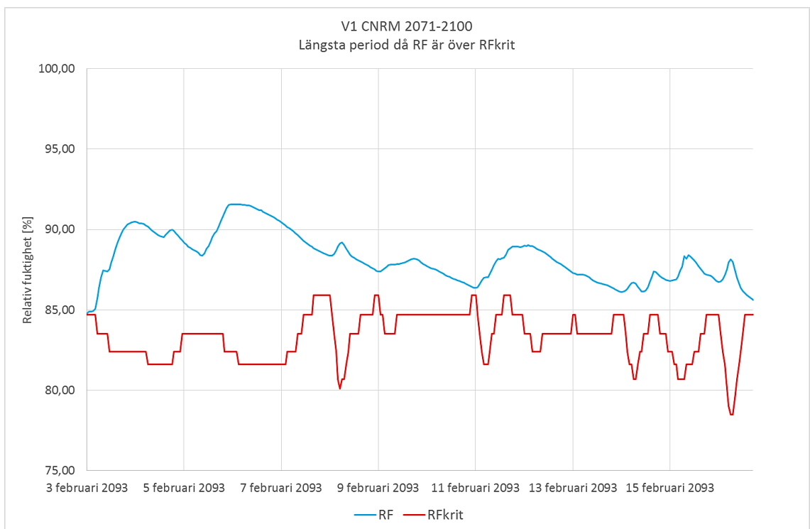
Figur 14.26 Längsta perioden då RF överskrider RF_{krit} är 13 dygn och 18 timmar.
