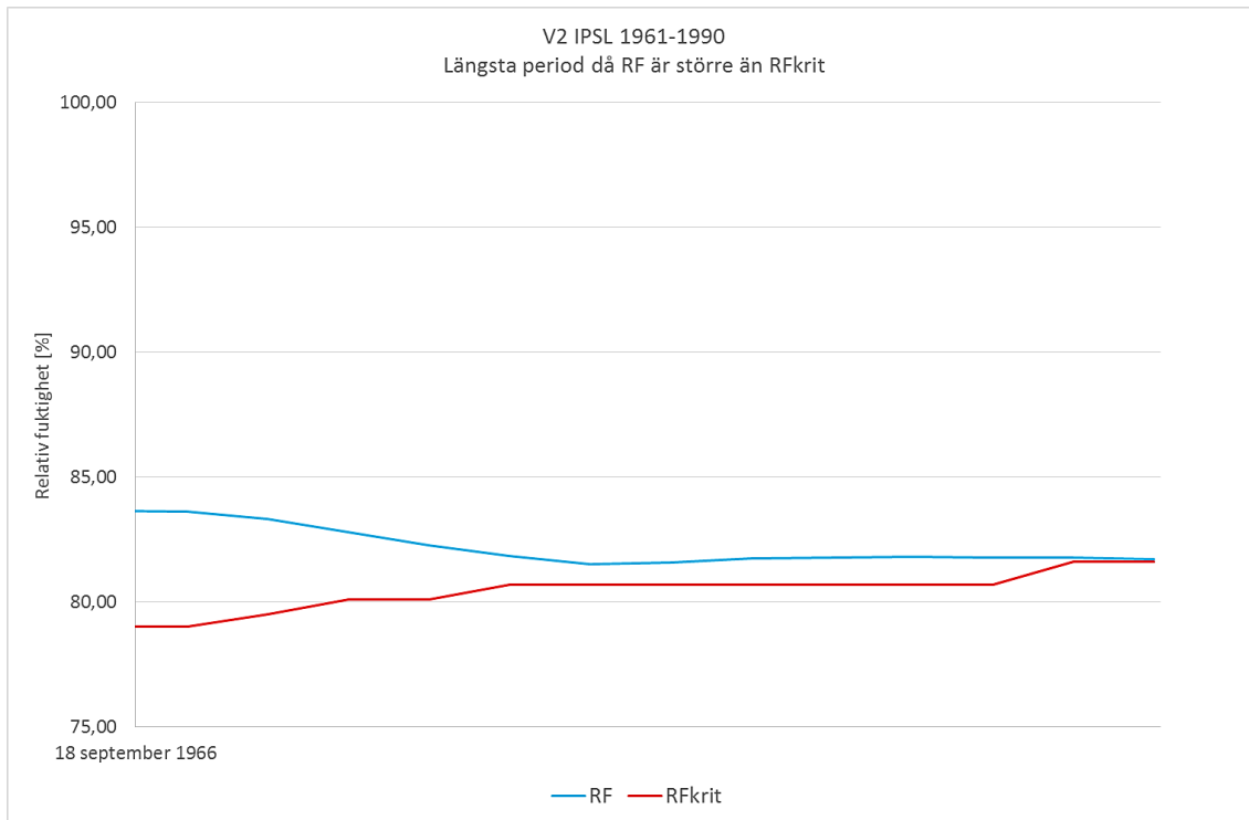
Figur 14.11 Längsta perioden då RF överstiger RF_{krit} är 18 timmar.
