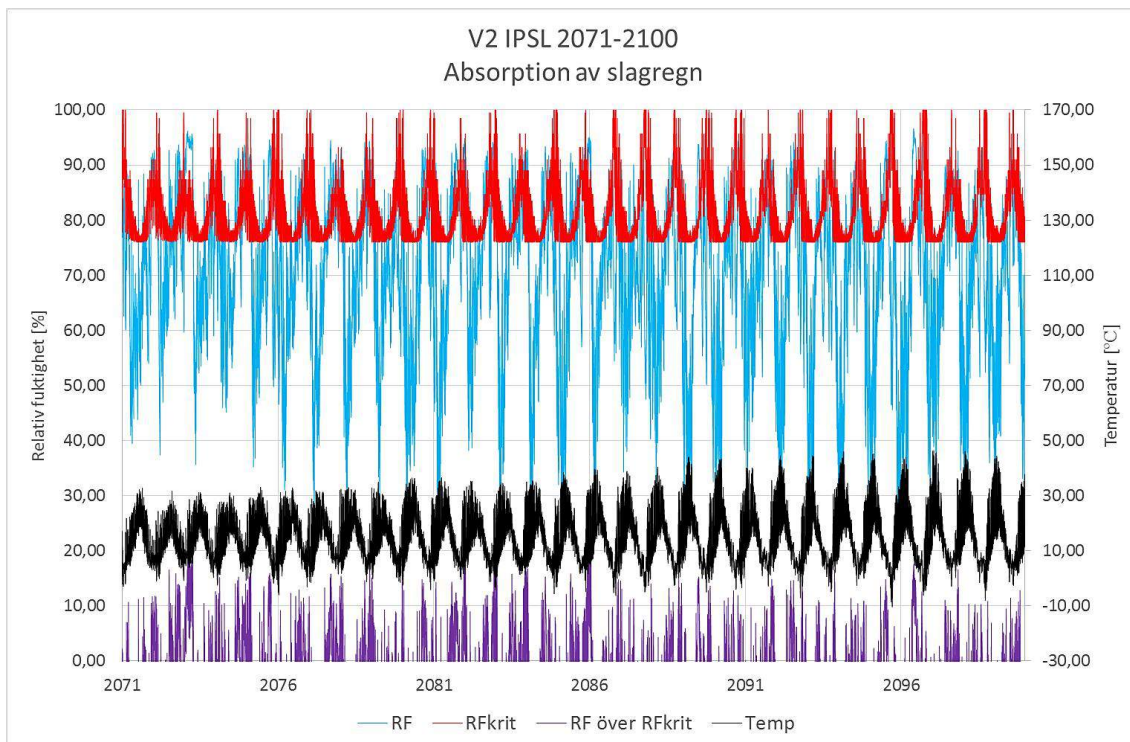
Figur 8.10 Folos-diagram för V2 IPSL 2071-2100.
