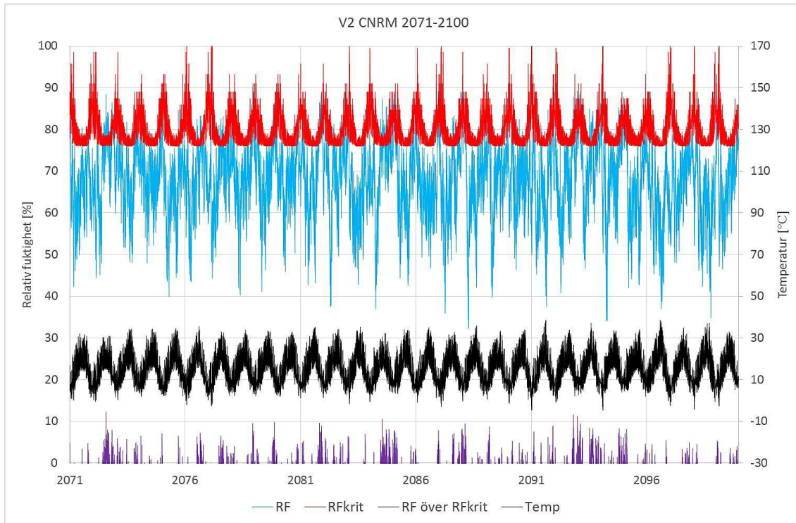
Figur 14.31 Folos-diagram för V2 CNRM 2071-2100.
