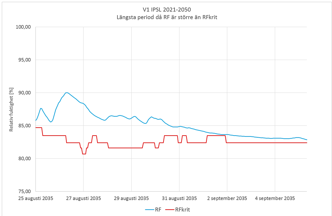
Figur 14.17 Längsta perioden då RF överskrider RF_{krit} är 11 dygn och 9 timmar.
