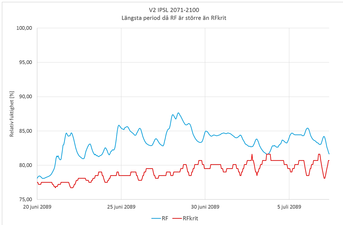
Figur 14.35 Längsta perioden då RF överstiger RF_{krit} är 17 dygn och 10 timmar.
