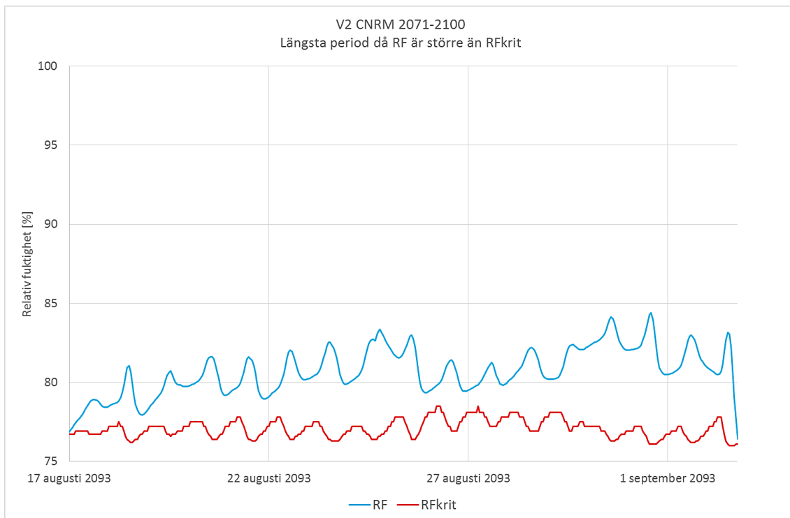
Figur 14.32 Längsta perioden då RF överstiger RF_{krit} är 16 dygn och 19 timmar.
