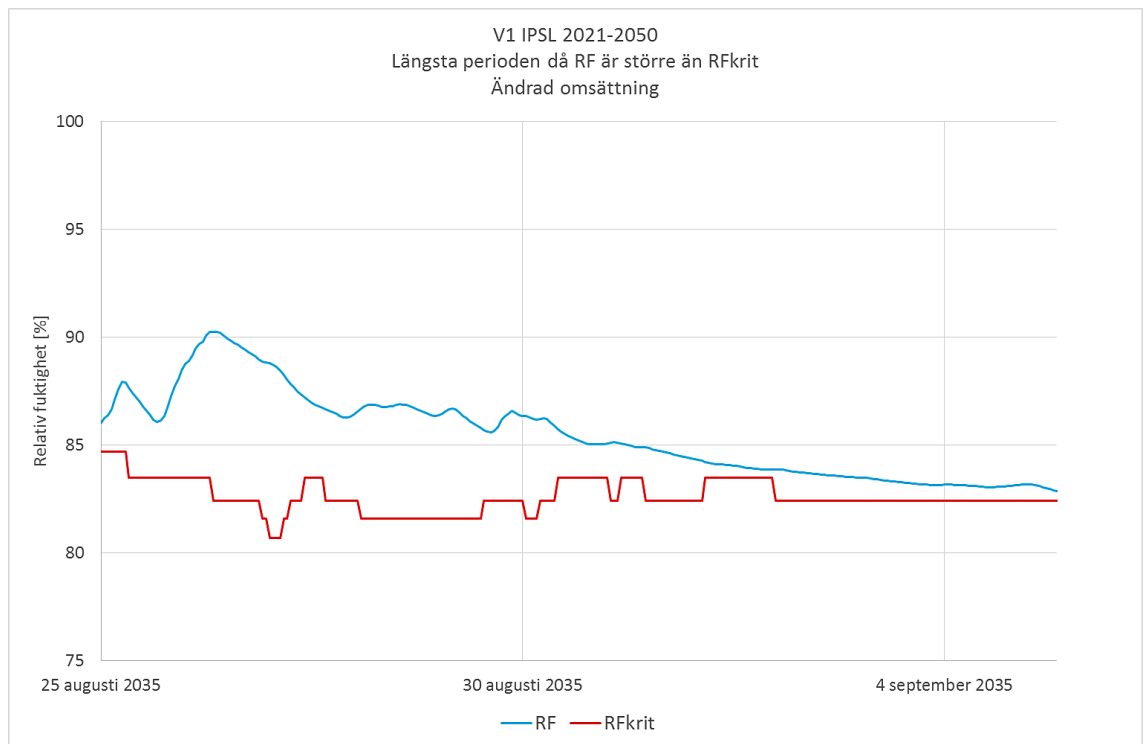
Figur 7.5 Längsta perioden då RF överstiger RF_{krit} är 11 dygn och 9 timmar.
