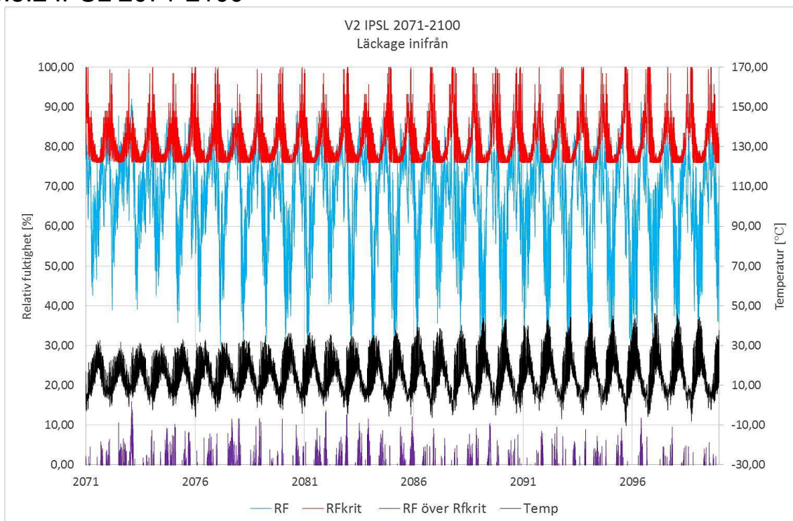
Figur 6.11 Folos-diagram för V2 IPSL 2071-2100.
