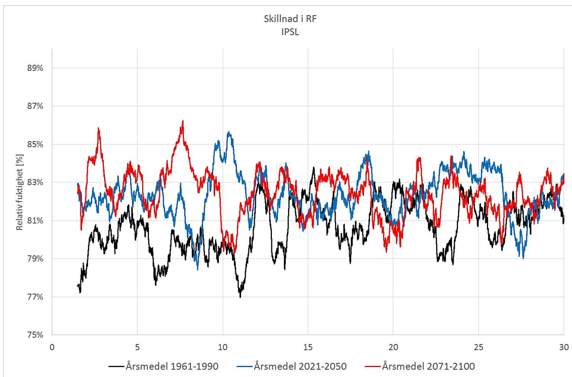
Figur 3.6 Skillnad i årsmedel, relativ, fuktighet, för klimatfil IPSL.
