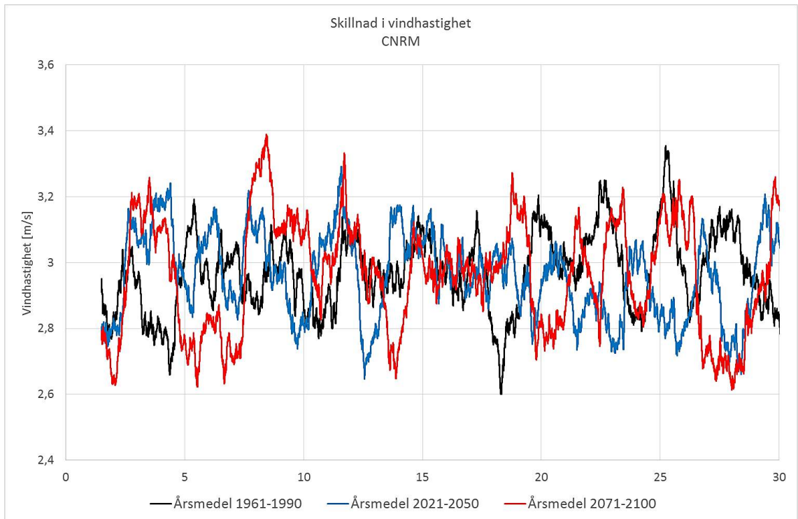
Figur 3.7 Skillnad i årsmedel, vindhastighet, för klimatfil CNRM.
