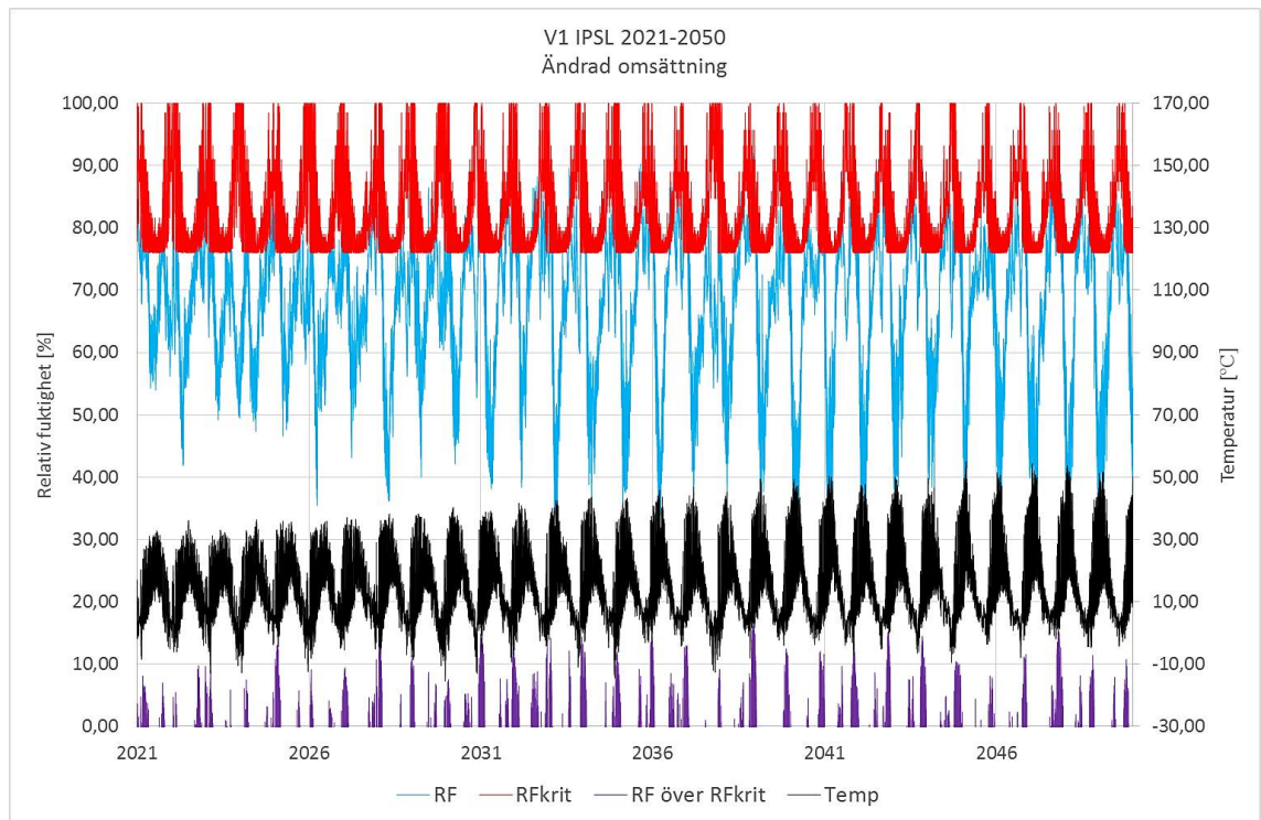
Figur 7.4 Folos-diagram för V1 IPSL 2021-2050.
