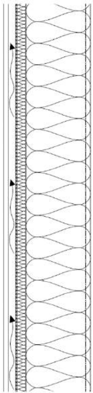
Figur 3.1 Uppbyggnad av V1
