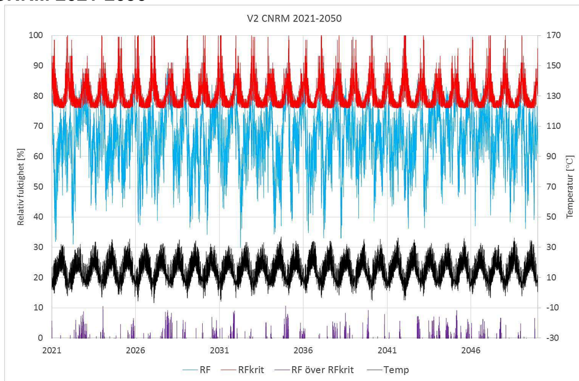
Figur 14.19 Folos-diagram för V2 CNRM 2021-2050.
