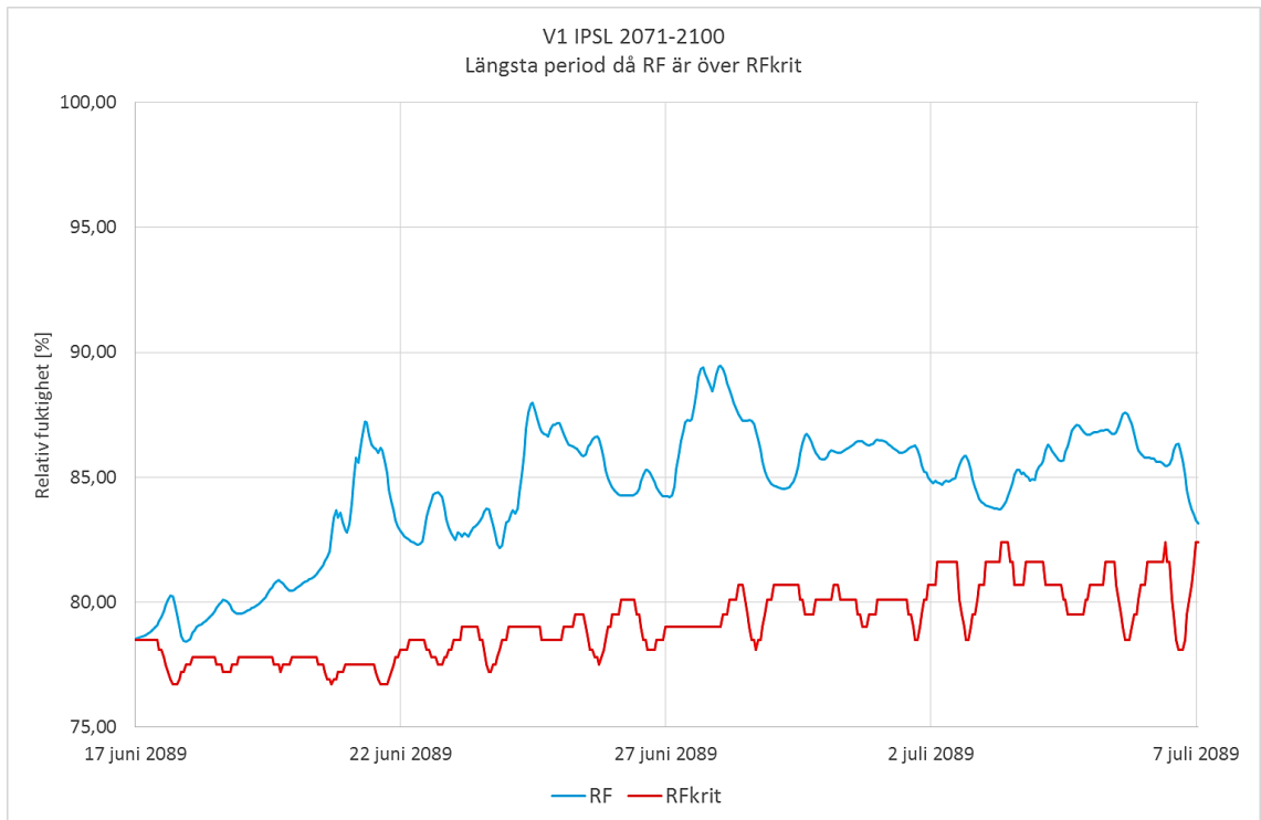
Figur 14.29 Längsta perioden då RF överstiger RF_{krit} 20 dygn och 2 timmar.
