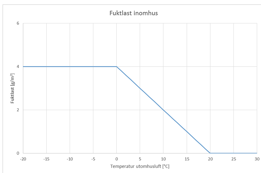
Figur 6.1 Fuktlast inomhus enligt WUFI:s EN13788 och fuktlast 2.
