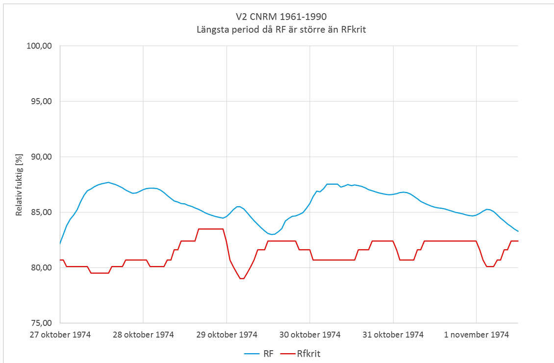
Figur 14.8 Längsta perioden då RF överstiger RF_{krit} är 5 dygn och 13 timmar.
