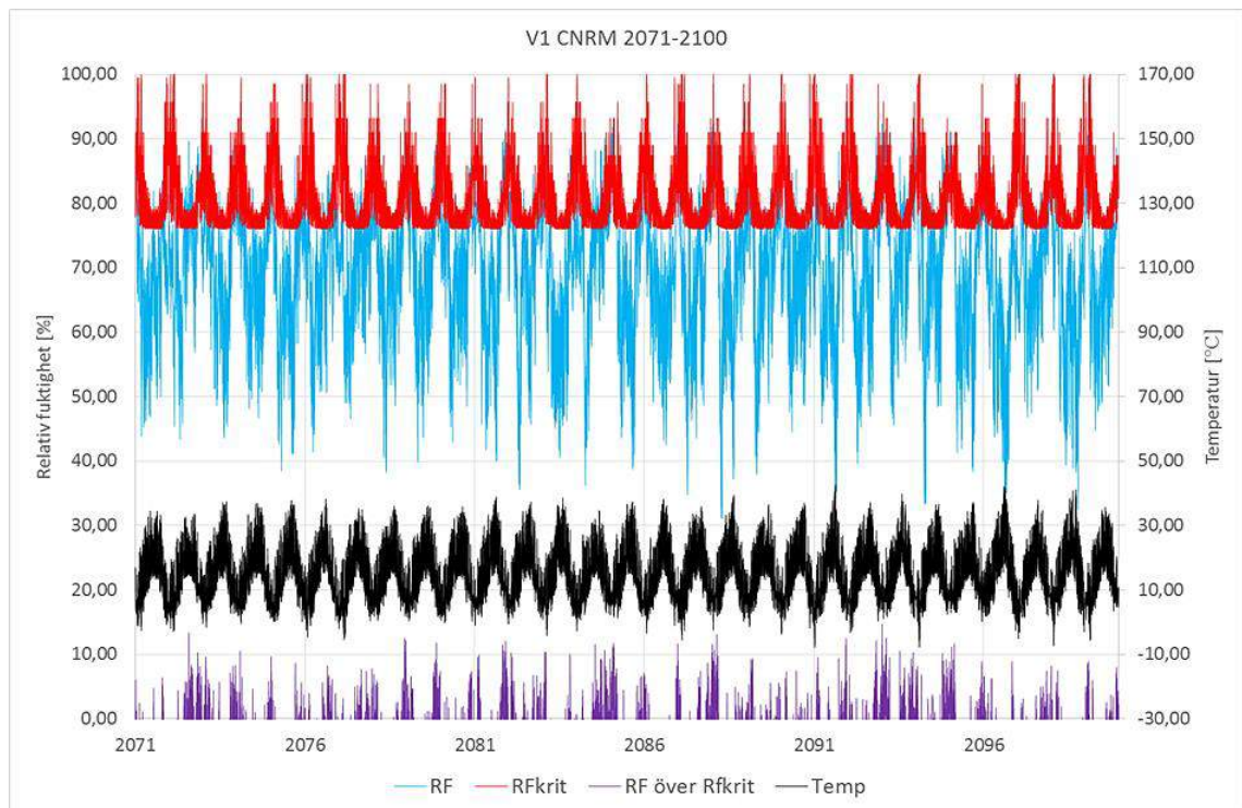
Figur 9.2 Folos-diagram för V1 CNRM 2071-2100 där fasaden är vänd mot syd.
