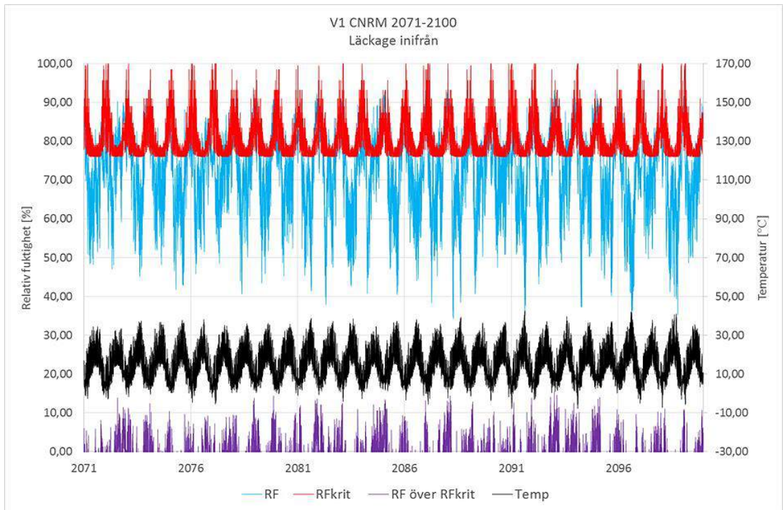
Figur 6.2 Folos-diagram för V1 CNRM 2071-2100.
