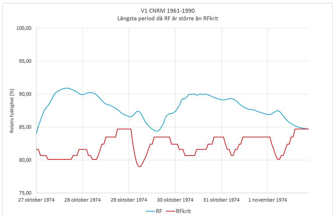
Figur 14.2 Längsta period då RF överskrider RF_{krit} är 5 dygn och 22 timmar.
