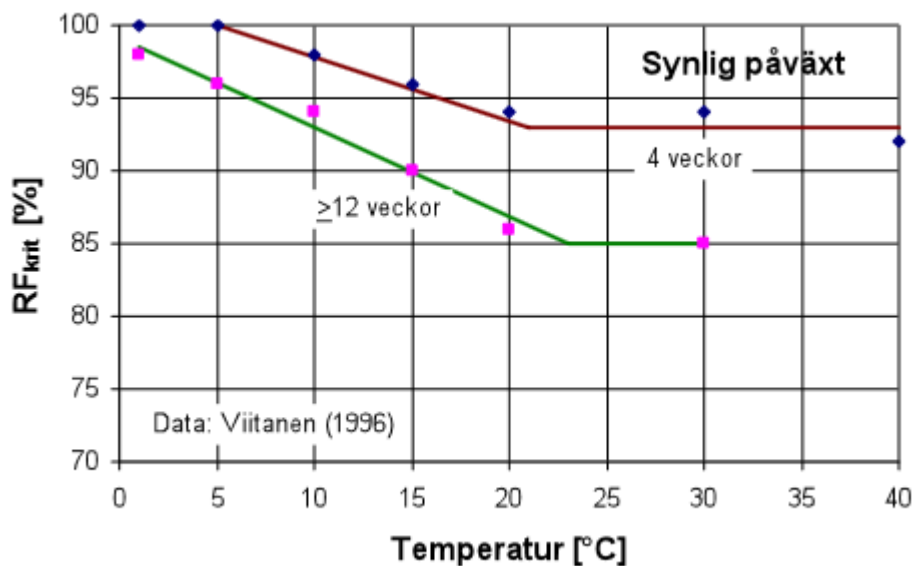
Figur 2.3 Kritiska fuktillstånd för "synlig" mögelpåväxt på trä vid olika temperaturnivåer och varaktigheter (Nilsson L-O, 2009).
