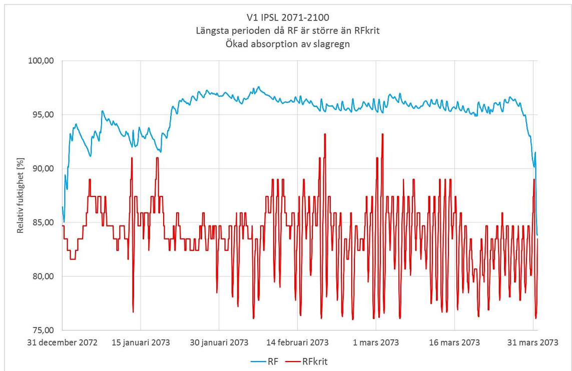
Figur 8.5 Längsta perioden då RF överskrider RF_{krit} är 90 dygn och 12 timmar.
