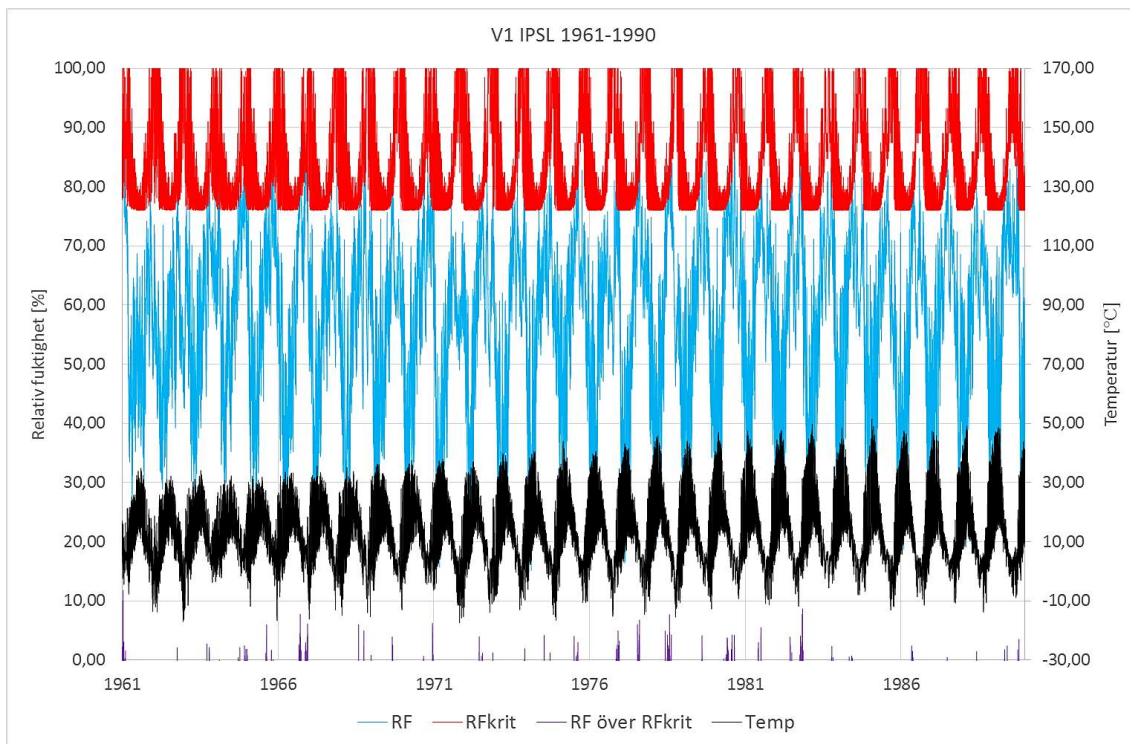
Figur 14.4 Folos-diagram för V1 IPSL 1961-1990.
