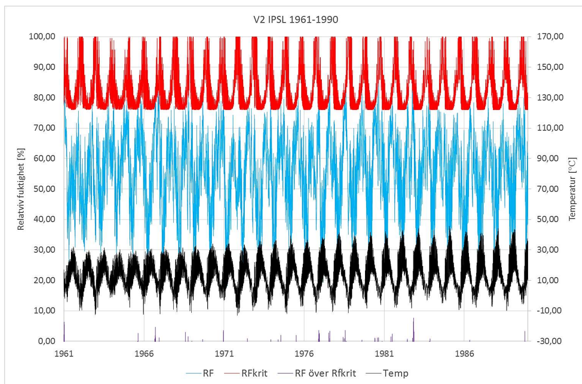
Figur 14.10 Folos-diagram för V2 IPSL 1961-1990.
