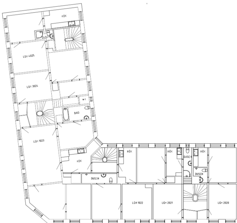
Figur 5-8: Planritning för plan 3. Ritningen visar var bärande tvärgående väggar finns.
