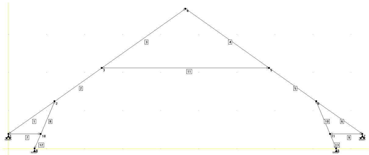
5-1: Geometri befintlig takstol med stödben.
