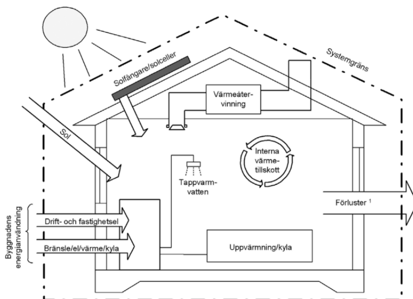
Figur 2-17: De olika posterna i en byggnads energianvändning (Boverket, 2008).
