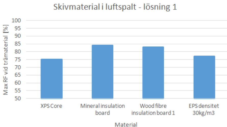
Figur 7-16: Olika fasadskivors inverkan på den relativa fuktigheten i ytterväggen, lösningsförslag 1.
