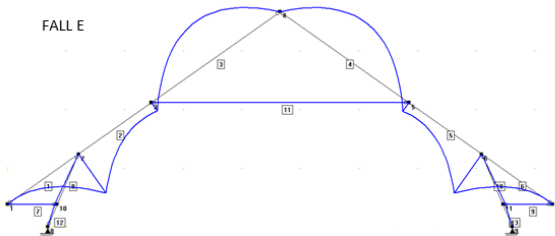
Figur 2-11: Momentfördelning, principfall 5.
