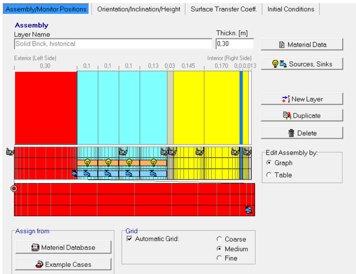
Figur 7-10: Modell av yttervägg, lösningsförslag 2.
