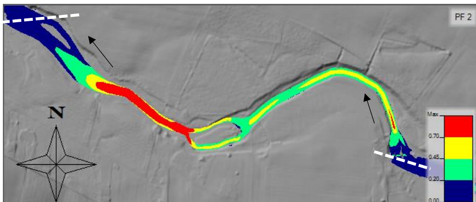
Figur 69 Strömshastigheter uppströms dämnet vid Bösmöllan vid djupare partiell utrivning, D-PU, sommartid, MQ, där blå är hastigheter under 0,2 m/s, grön är 0,2 – 0,45, gul är 0,45 och röd är hastigheter över 0,7 m/s. De vita streckade linjerna visar dämmens position. Bakgrund från höjddata 2 m raster, © Lantmäteriet.
