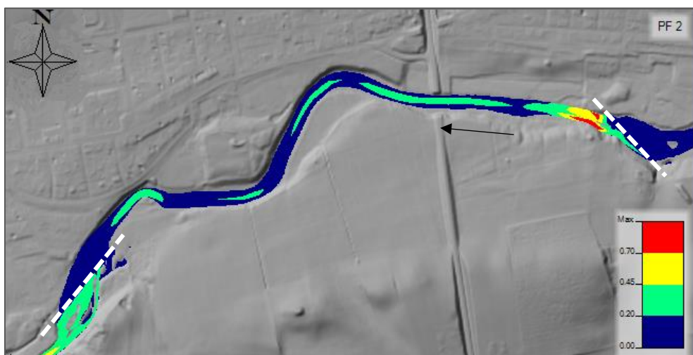
Figur 58 Strömshastigheter uppströms dämmet vid Silverforsen i dagsläget, sommartid, MQ, där blå är hastigheter under 0,2 m/s, grön är 0,2 – 0,45, gul är från 0,45 och röd är hastigheter över 0,7 m/s. De vita streckade linjerna visar dämmens position. Bakgrund från höjddata 2 m raster, © Lantmäteriet.
