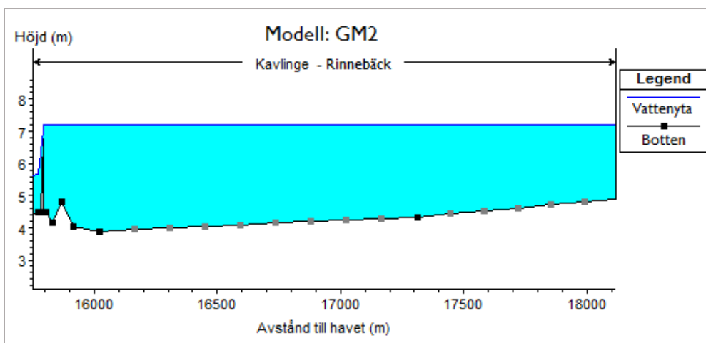
Figur 49 Modell 2: Maximalt djup i tvärsnitten (svarta/grå punkter) strax innan dämnet vid Rinnebäck, simulerat för lågt flöde (illustrerat i blått).
