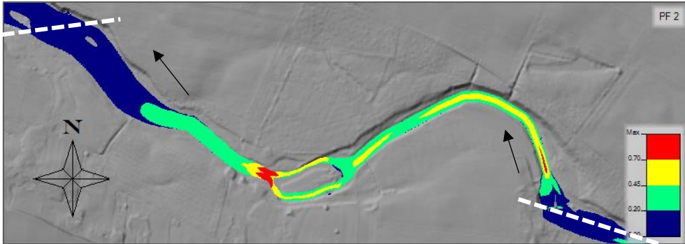
Figur 67 Strömhastigheter uppströms dämnet vid Bösmöllan i dagsläget, sommartid, MQ, där blå är hastigheter under 0,2 m/s, grön är 0,2 – 0,45, gul är från 0,45 och röd är hastigheter över 0,7 m/s. De vita streckade linjerna visar dämmens position. Bakgrund från höjddata 2 m raster, © Lantmäteriet.
