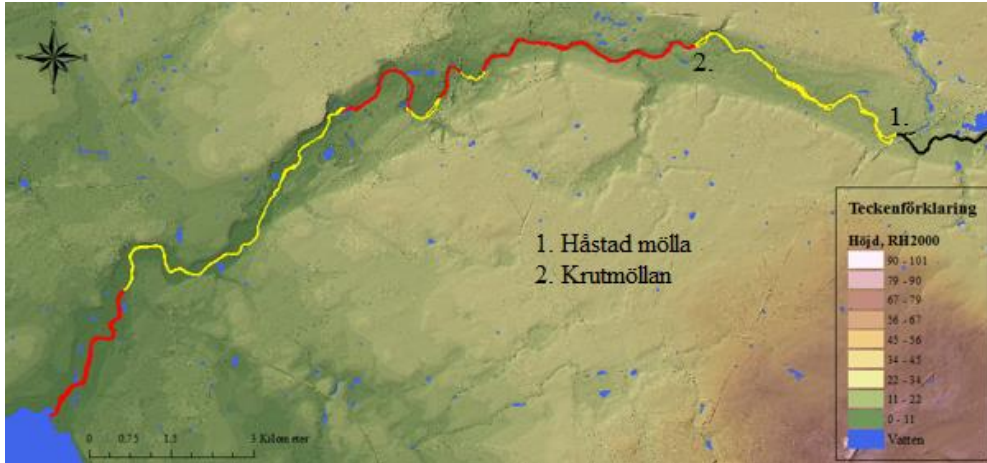
Figur 34 Dataunderlag till modellering. Det svarta området representerar åfåra baserat på tvärsektioner från broar, det röda området är baserat på ekolodsdata och det gula området är uppskattat efter övrigt dataunderlag. Det svarta området sträcker sig från Vombsjön ca 2,7 mil nedströms till Håstad mölla. Den kortare modellen börjar vid det ekolodade området, strax efter Krutmöllan. Höjddata med ursprung 2 m raster, © Lantmäteriet.
