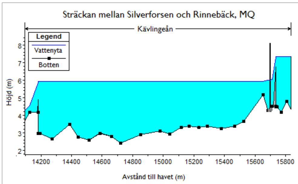
Figur 57 Profil över vattendjup vid MQ och botten så som modellen representerar dagsläget vid Silverforsen, GM1. Till vänster syns dämmet vid Silverforsen, till höger syns gångbron och dämmet vid Rinnebäck. Höjden på dämmena varierar över hela dämmets längd, den nivå som syns här är lägsta punkten på dämmet.
