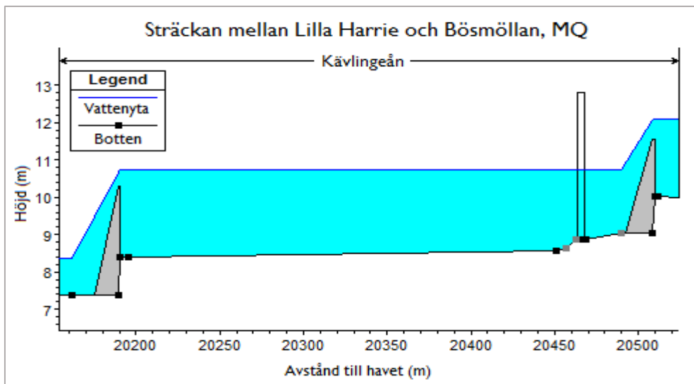
Figur 64 Profil över vattendjup vid MQ och botten så som modellen representerar dagsläget vid Lilla Harrie, GM2. Till vänster syns dämnet vid Lilla Harrie, till Höger syns gångbron och dämnet vid Bösmöllan. Höjden på dämmena varierar över hela dämmets längd, den nivå som syns här är lägsta punkten på dämnet.
