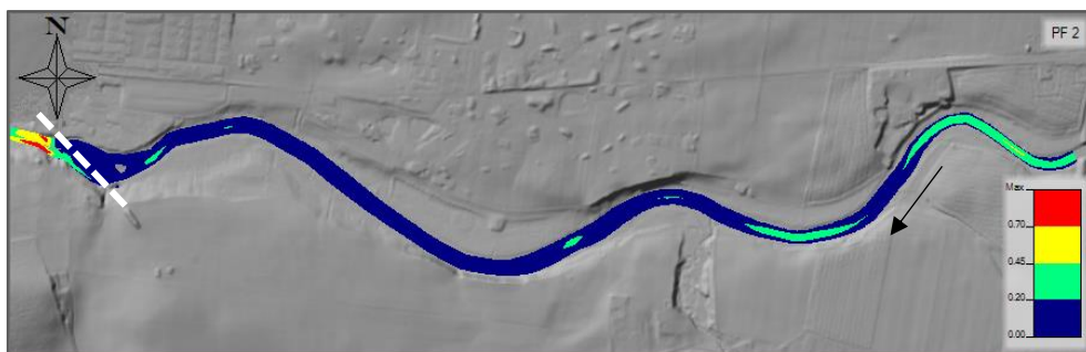
Figur 62 Strömförhållanden uppströms Rinnebäck i dagsläget vid MQ då majoriteten av området är svagt strömmande. GM1. De vita streckade linjerna visar dämmens position. Bakgrund från höjddata 2 m raster, © Lantmäteriet.
