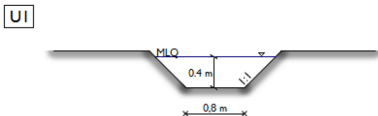
Figur 45 Utskov, U1, utformat efter förslag från miljökonsekvensbeskrivningar.
