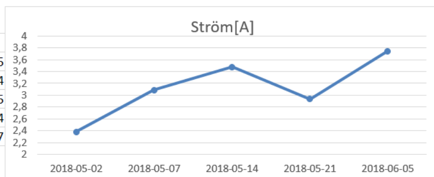
Figur 14. Genomsnittliga strömförbrukningen under mätningarna på maskin 2
