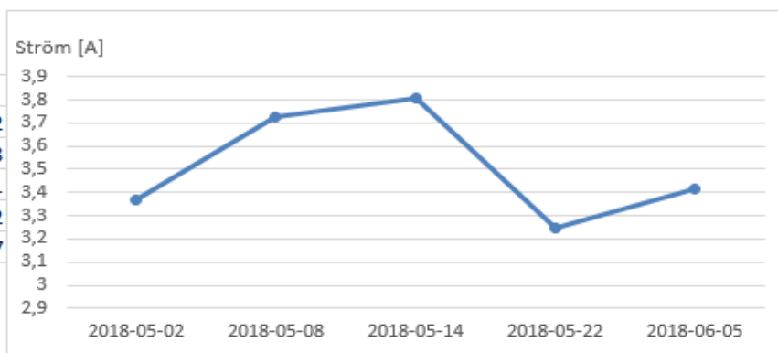
Figur 13. Genomsnittliga strömförbrukningen under mätningarna på maskin 1
