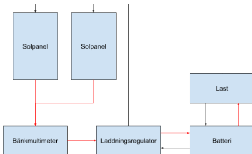
Figur. 15. Mätning; solpaneler
