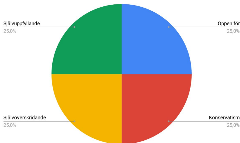
Figur 4.1: Redogörelse för vilka färger som representerar de fyra dimensionerna som utgör grunden för partiernas två index.
