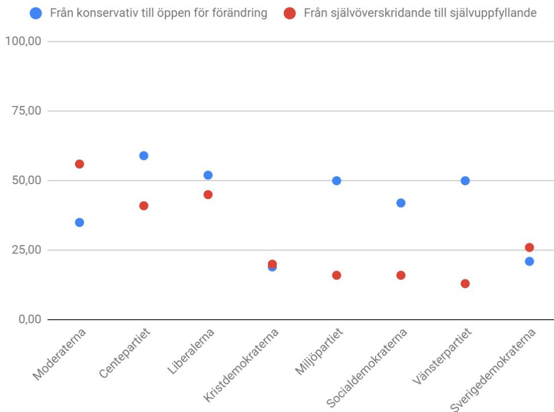
Figur 4.4: Sammanställning av riksdagspartiernas index. De blå prickarna står för index K-ÖFF. Ju närmare värdet 0 ett parti hamnar desto mer konservativa är dem och ju närmare värdet 100 desto mer öppet för förändring. De röda prickarna står för Index SÖ-SU. Ju närmare värdet 0 desto mer självöverskridande är partiet och ju närmare värdet 100 desto mer självuppfyllande är partiet.
