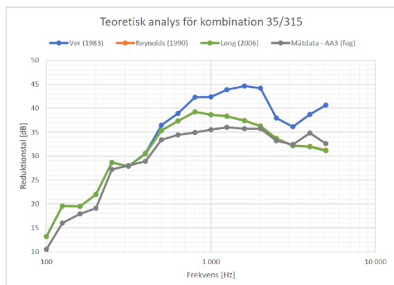
Genomföring av kanal med dimension \varnothing 315 mm i vägg med lägst ljudklass, R'w : 35 dB. Jämförelse av tre befintliga teorier mot mätdata.
