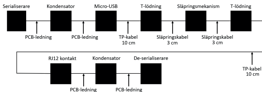
Figur 9: Blockdiagram för uppställningen då släpringen är kopplad mellan serialiseraren och de-serialiseraren med T-lödingar. MicroUSB-kontakt och RJ12-kontakt användes på respektive PCB.
