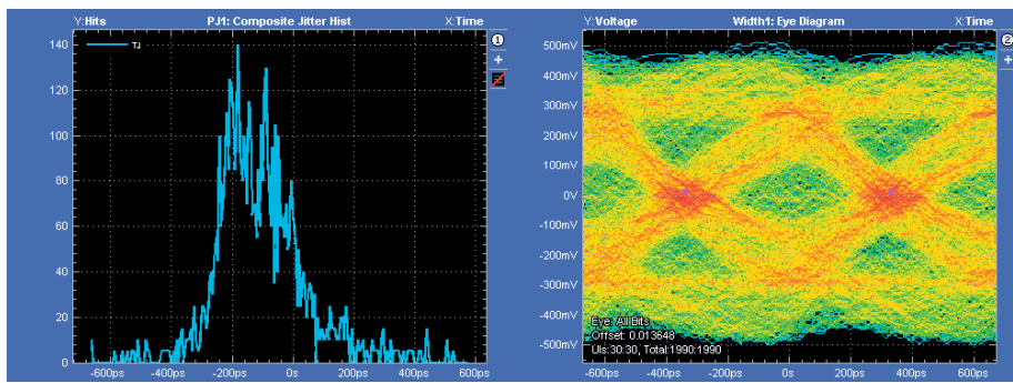
Figur 24: Ögonogram samt jitterhistogram på de-serialiseraren från att först vara stationär till att sedan rotera, med uppställning enligt figur 13 med en släpning som roterat tre miljoner varv.
