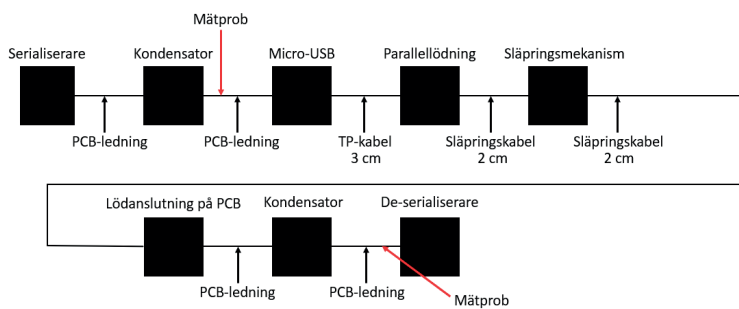
Figur 13: Blockdiagram för uppställningen då ögonogram och jitterhistogram gjordes. Mätningen gjordes differentiellt mellan data+ och data- då släpringsladdar var kopplad mellan serialiseraren och de-serialiserearen med parallellödningskablar. MicroUSB-kontakt användes mellan serialiseraren och lödning direkt på PCBet där RJ12-kontakten satt användes mot de-serialiserearen.
