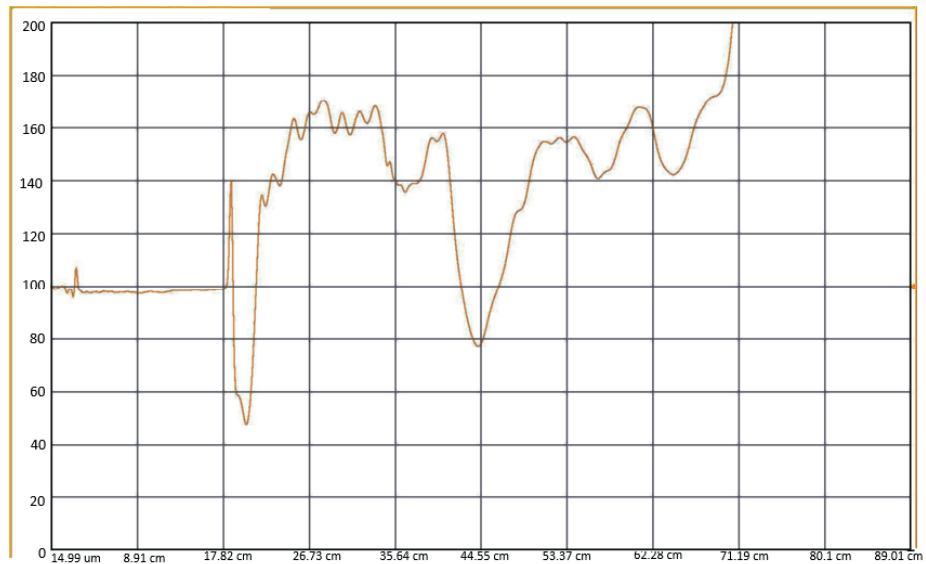
Figur 27: TDR-mätning över släpring med en öppen krets på den borte änden i mätupställningen. Uppställning enligt figur 15. Y-led visar karakteristisk impedans i ohm [\Omega] . X-led visar placering i den länk som mätningen görs på, med startpunkt i instrumentets kabelkontakt, i enhet meter [m] .
