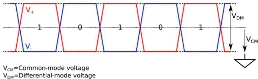
Figur 7: Typutseende för en differentiell signal, V_+ skickas synkroniserat med sin invers V_- . [12]
