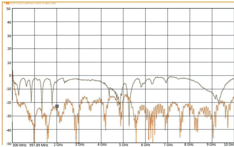
Figur 29: Ett frekvenssvöp som visar den reflekterade energin i länken som testas, för respektive frekvens. Den nedre kurvan visar kalibreringskurvan och den övre visar energin som reflekteras i länken med släpringen. Y-led visar reflektioner i enhet decibel [dB], X-led visar frekvensi enhet Hertz [Hz].
