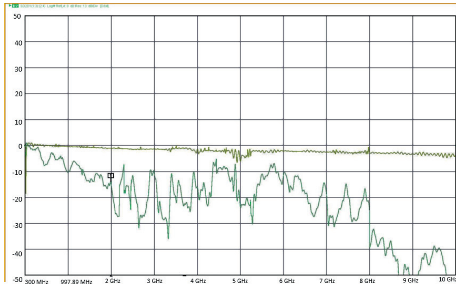
Figur 28: Ett frekvenssvop som visar den energin som kommit igenom länken som testas, för respektive frekvens. Den nedre kurvan visar den energin som kommit igenom länken med släpringen för respektive frekvens. Den övre kurvan visar kalibreringskurvan. Y-led visar förluster i enhet decibel [dB], X-led visar frekvens i enhet hertz [Hz].
