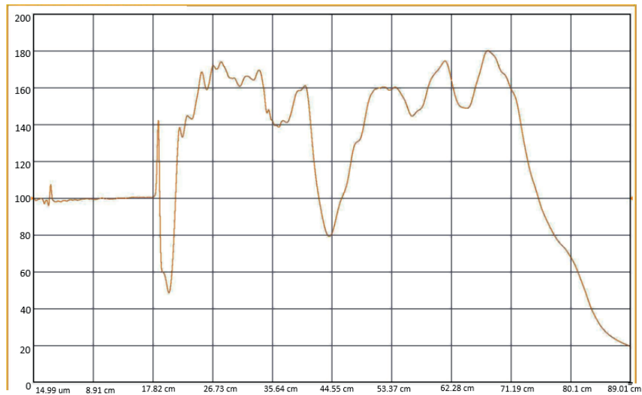
Figur 26: TDR-mätning över släpring med en kortslutning på den bortre änden i mätupställningen. Uppställning enligt figur 15. Y-led visar karakteristisk impedans i ohm [Ω]. X-led visar placering i den länk som mätningen görs på, med startpunkt i instrumentets kabelkontakt, i enhet meter [m].
