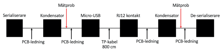
Figur 12: Blockdiagram för uppställningen då ögonogram och jitterhistogram gjordes. Mätningar gjordes differentiellt mellan data+ och data- då medföljande 8 m originalkabel användes mellan serialiseraren och de-serialiserearen.
