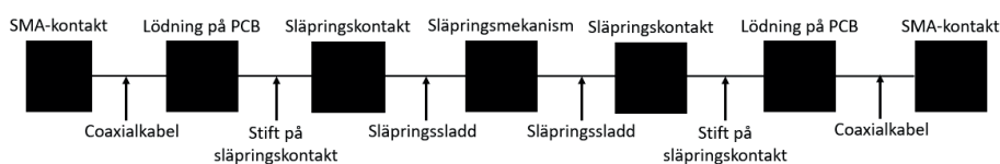
Figur 15: Blockdiagram för uppställning när impedans och frekvensanalyser gjordes. SMA-kontakter i ändarna fastlödda på släpringskontakten där släpringen var inkopplad.
