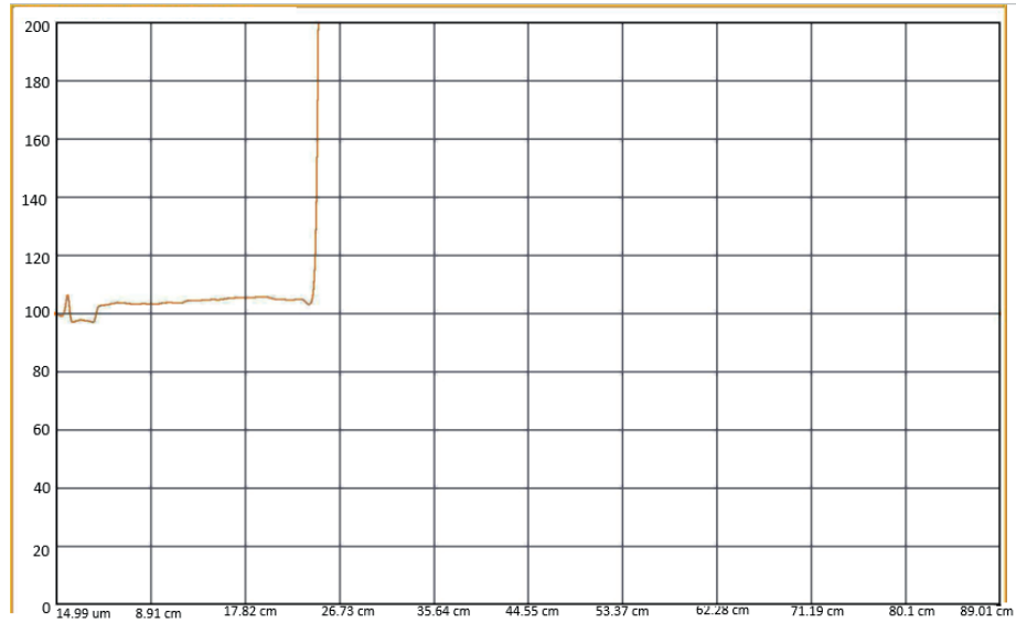
Figur 25: Kalibrering av mätutrustning inför TDR-mätningar, med öppen ändpunkt. Y-led visar karakteristisk impedans i ohm [ \Omega ]. X-led visar placering i den länk som mätningen görs på, med startpunkt i instrumentets kabelkontakt, i enhet meter [m].
