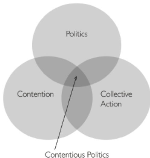
Figur 1: Den analytiska skärningspunkt som uppstår när begreppen "contention", "collective action" och "politics" överlappar varandra (Brink Pinto, Ericsson & Nyzell 2015, s. 97)
