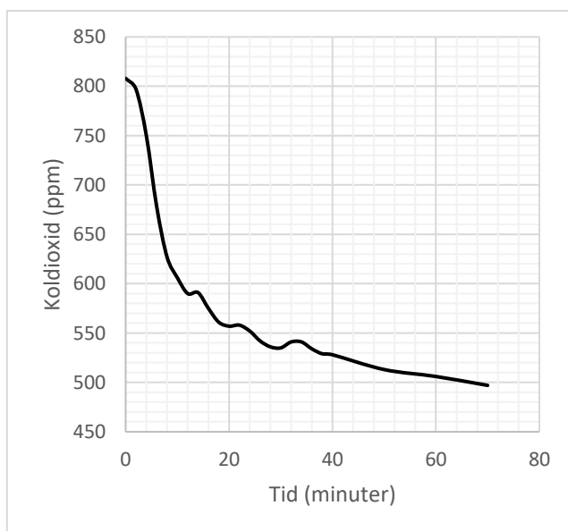
Fig. 21. Koldioxid i rummet från att fönstret öppnas.
