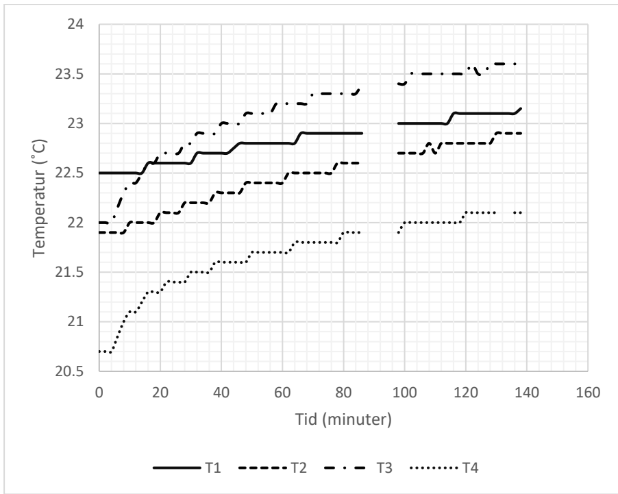
Fig. 4. Temperatur för 750 W element.
