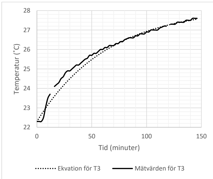
Fig. 16. Jämförelse mellan ekvation (18) och mätvärden för sensor T3 med elementet på 2000 W.
