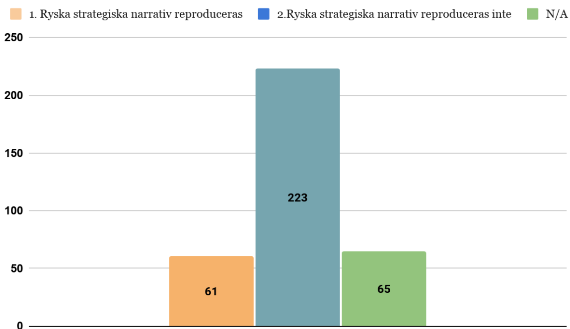
Figur 1, variablernas frekvens
