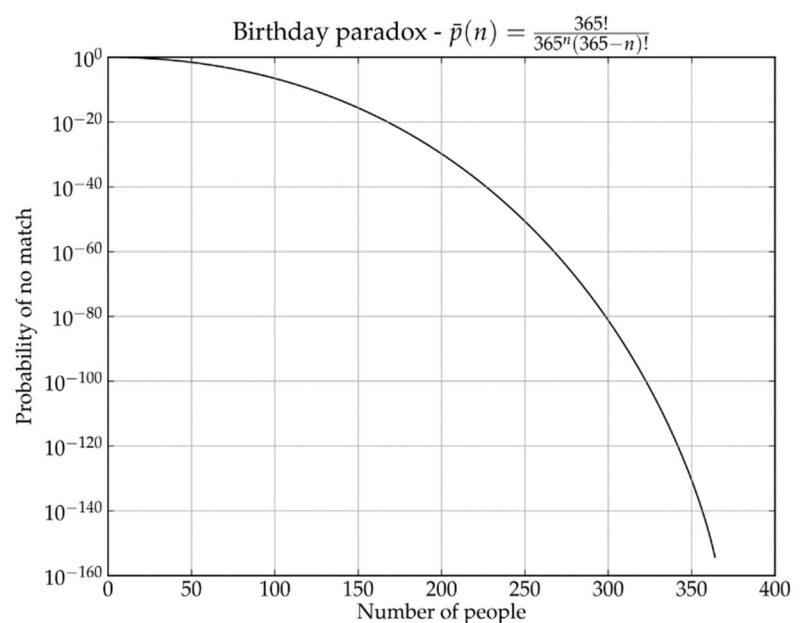
Figur 4 Födelsedagsproblemet som graf. Källa: Wikipedia, 2021.
