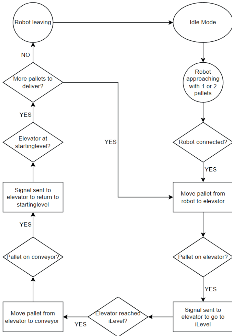
Figur 12: Flödesschema för en DropOff-sekvens
