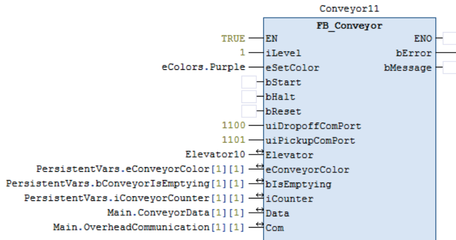
Figur 10: Instans av funktionsblocket FB_Conveyor
