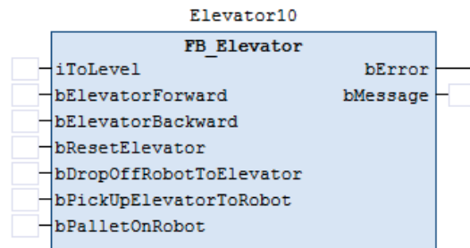
Figur 9: Instans av funktionsblocket FB_Elevator
