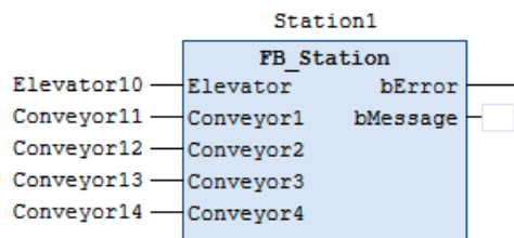
Figur 8: Instans av funktionsblocket FB_Station
