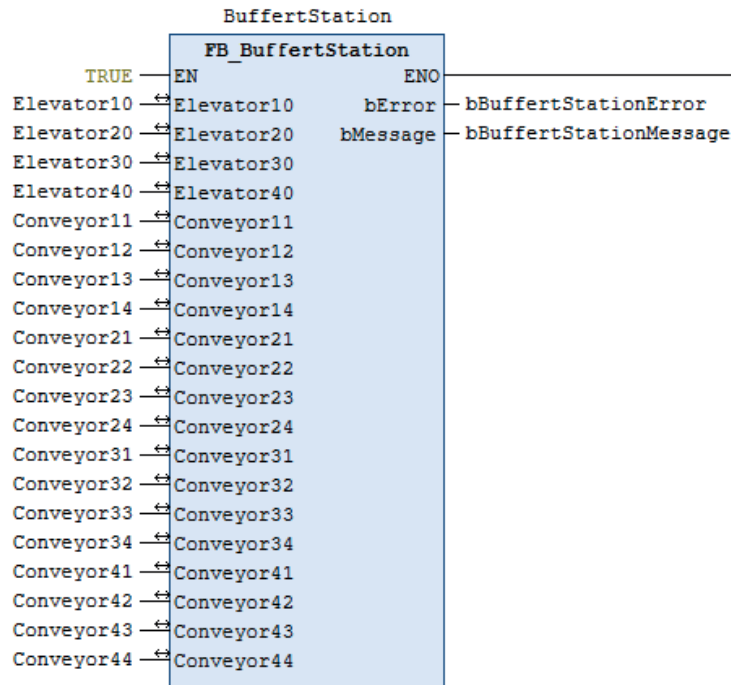
Figur 7: Instans av funktionsblocket FB_BufferStation
