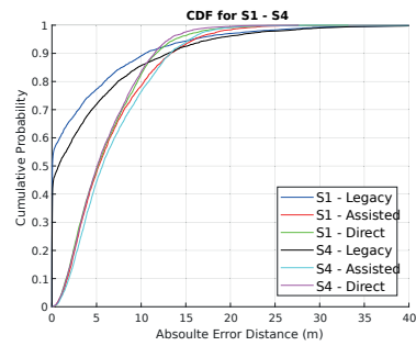
(d) CDFs for Scenario 1 and 4
