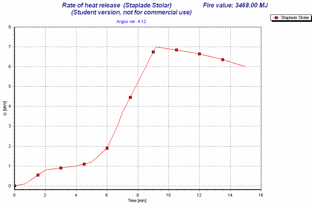
Figur 9.3 Effektkurva, Tankerummet
