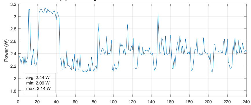
(d) CPUFreq + CPUIdle + Wiegand + JMeter.
