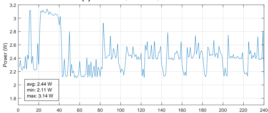
(d) CPUIdle + Wiegand + JMeter.
