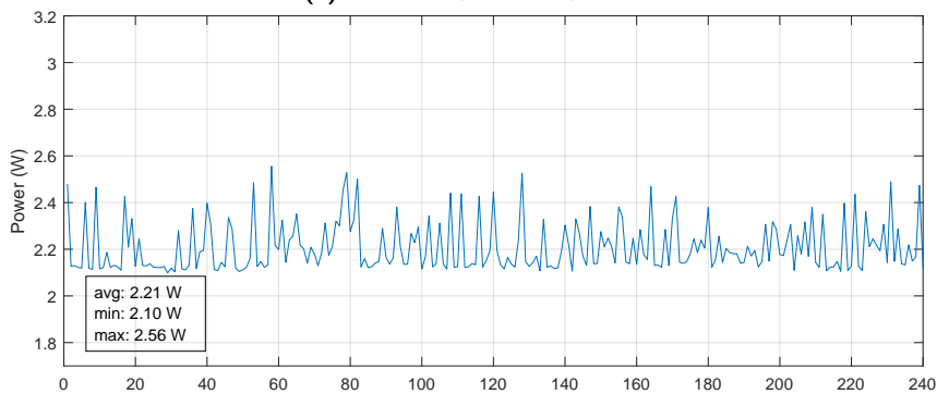
(b) CPUIdle + Wiegand + Idle.
