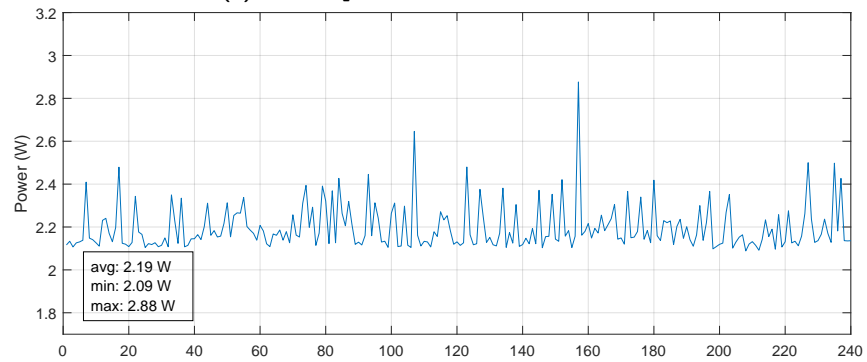
(b) CPUFreq + CPUIdle + Wiegand + Idle.
