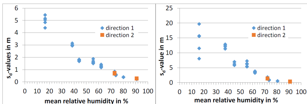
Figur 2.16 Uppmätta S_d - värde för produkt C och D, (Fechner och Meißner, 2017).
