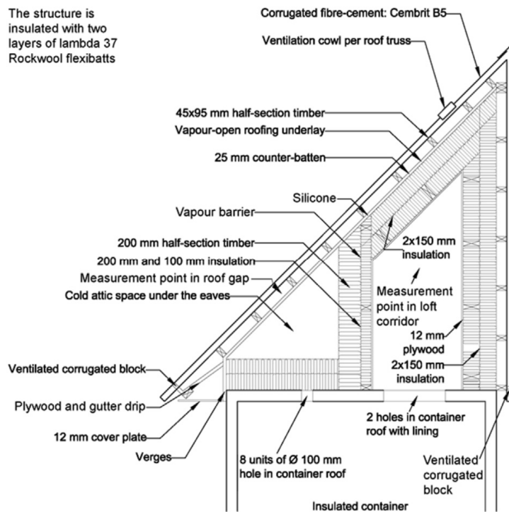
Figur 2.2 Sektion av provhuset i Lyngby.
