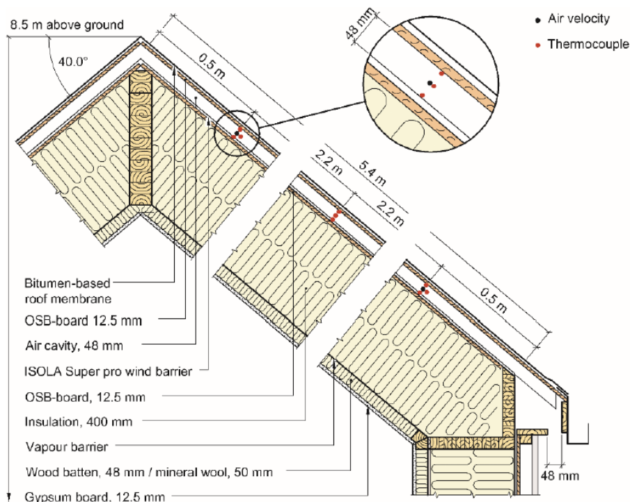
Figur 2.18 Principiell uppbyggnad av det kompakta taket i provhuset i Trondheim, (Gullbrekken et al, 2017).
