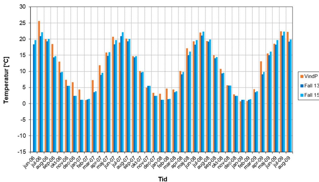
Figur 5.9 Jämförelse mellan uppmätta och beräknade månadsmedelvärden mot norr av temperaturen (°C) i vindsutrymme med traditionell underlagstäckning av papp. Betydelsen av VindP framgår av tabell 3.1.
