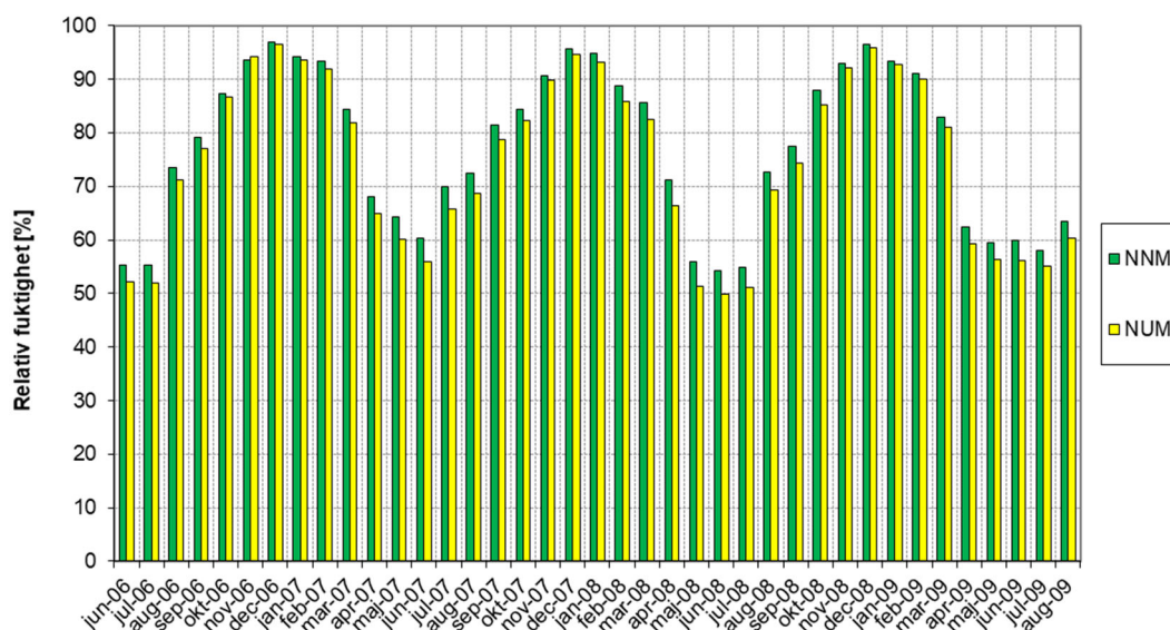
Figur 3.16 Månadsmedelvärden för relativ fuktighet (%) från två loggrar mot norr med ånggenomsläppligt ytskikt på råsponten.
