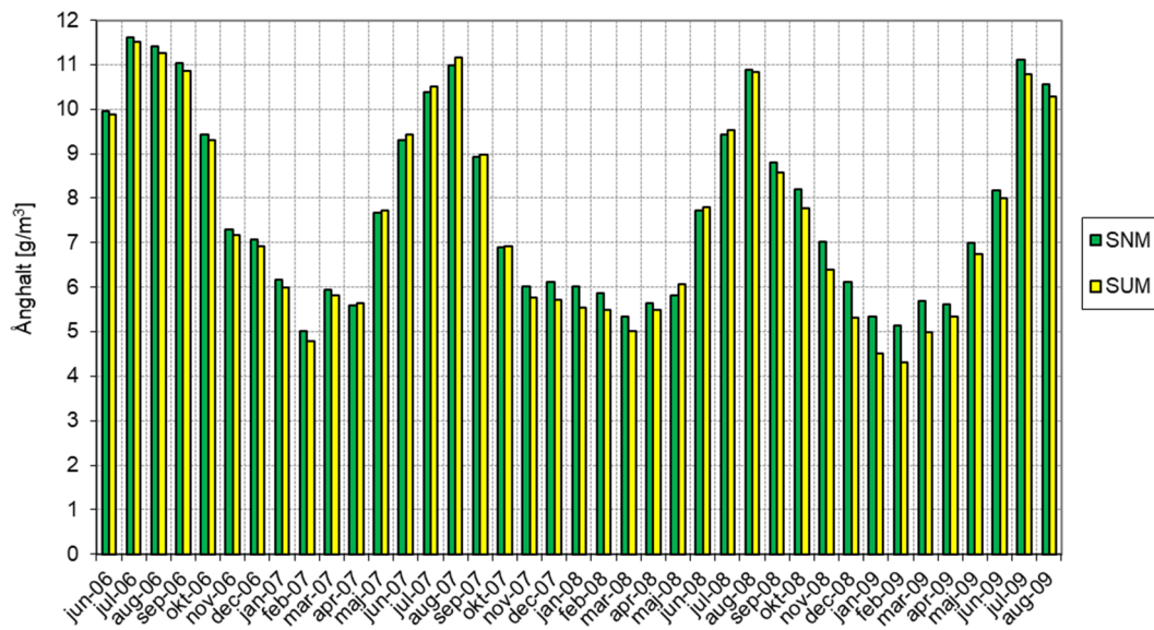
Figur 3.20 Månadsmedelvärden för ånghalt ( \text{g/m}^3 ) från de två loggrar mot söder som fanns ovanför takdelen med ånggenomsläppligt ytskikt på råsponten.
