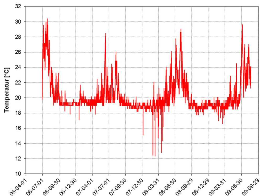
Figur 3.7 Inomhustemperatur under hela mätperioden.
