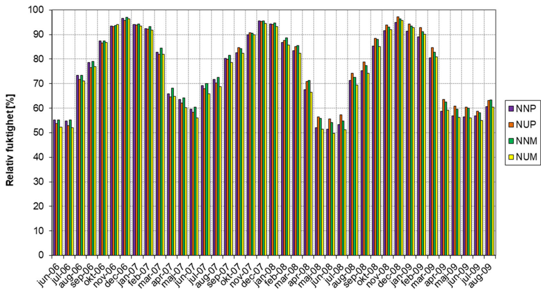
Figur 3.14 Månadsmedelvärden för relativ fuktighet (%) från samtliga fyra loggrar mot norr.
