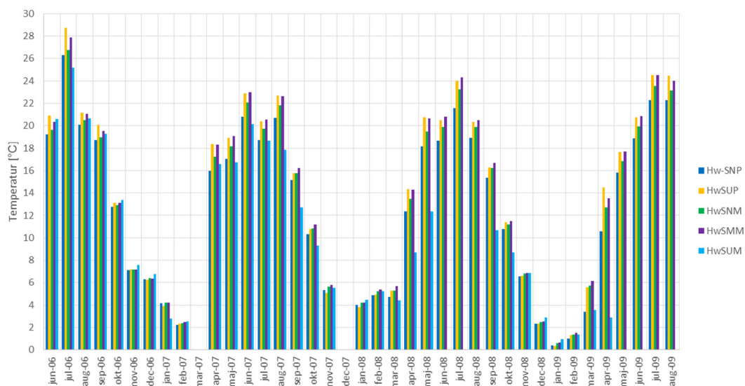
Figur 3.36 Månadsmedeltemperaturer mot söder från samtliga sensorer mellan råspont och underlagstäckning.
