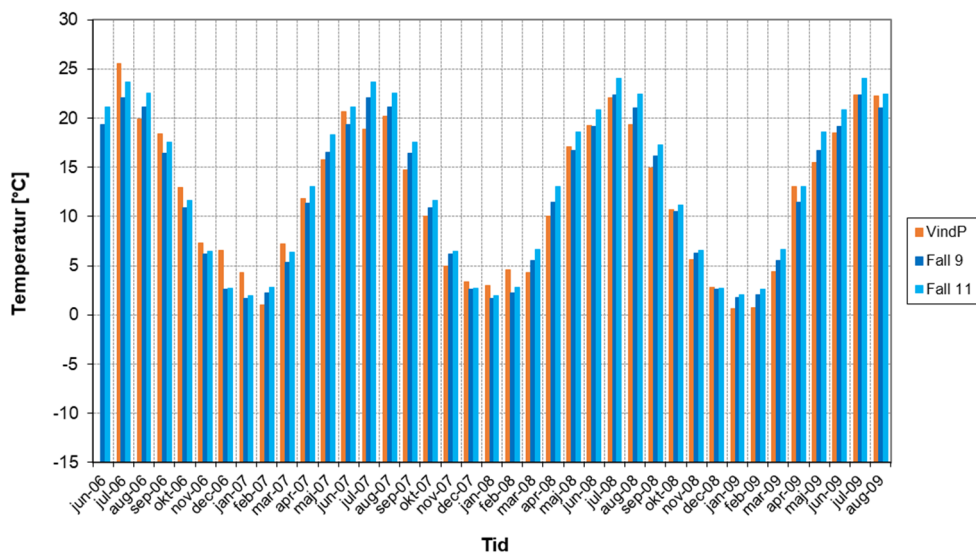
Figur 5.8 Jämförelse mellan uppmätta och beräknade månadsmedelvärden mot söder av temperaturen (°C) i vindsutrymme med traditionell underlagstäckning av papp. Betydelsen av VindP framgår av tabell 3.1.
