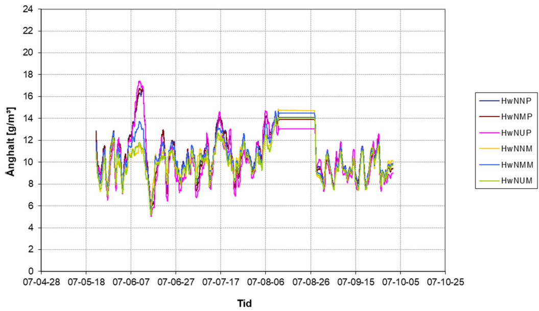
Provhuset - tak, Honeywell Norr Glidande dygnsmedelvärde 070521-071001
