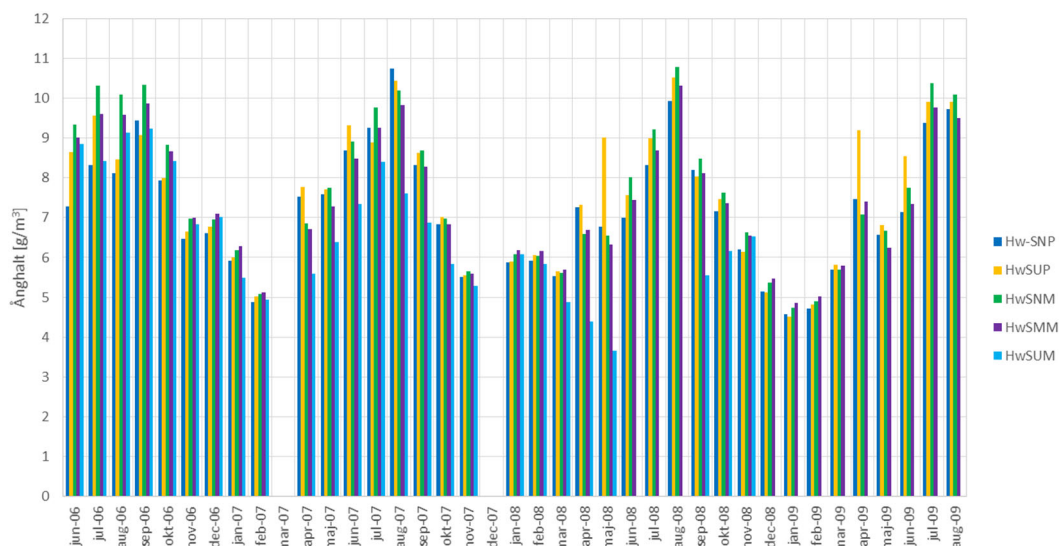
Figur 3.53 Månadsmedelvärde för ånghalt ( \text{g}/\text{m}^3 ) avseende samtliga fem sensorer mot söder mellan råspont och underlagstäckning.
