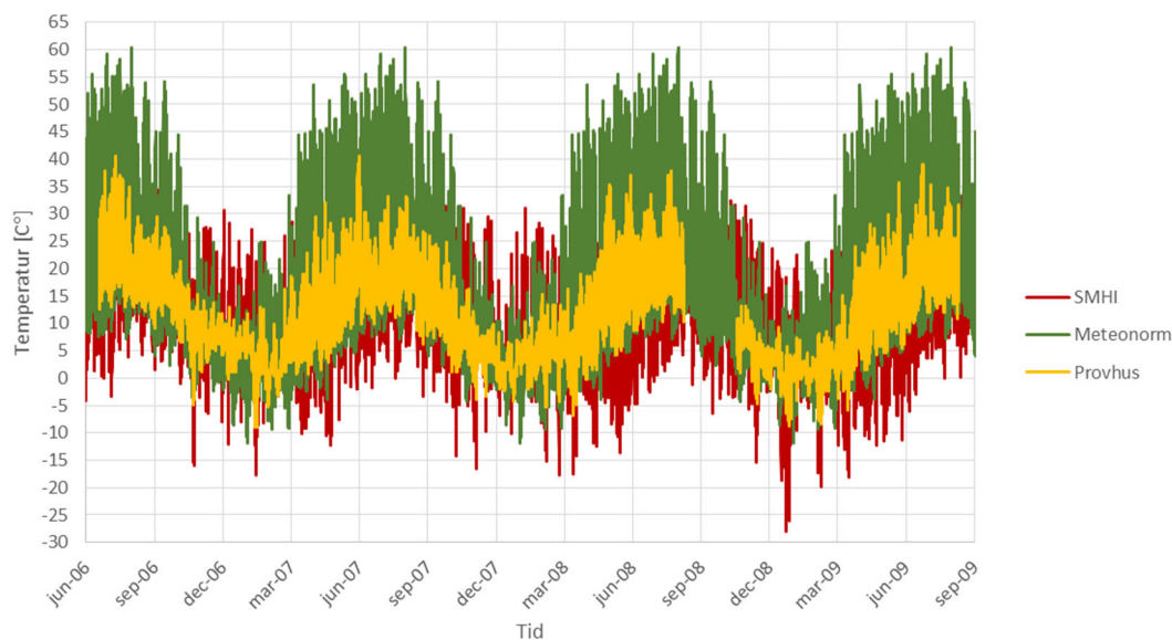
Figur 5.1 Uppmätt temperatur intill provhuset samt utomhustemperatur från SMHI och Meteonorm för samma tidsperiod.
