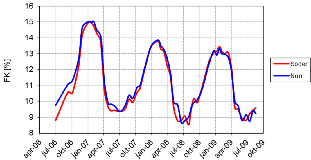
Figur 3.31 Uppmätt temperaturkorrigerad fuktkvot (%) på vinden. Medelvärde för samtliga mätpunkter mot söder respektive mot norr.
