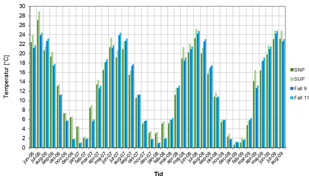
Figur 5.2 Jämförelse mellan uppmätta och beräknade månadsmedelvärden av temperaturen (°C) mot söder under takpannorna med traditionell underlagstäckning av papp. Betydelsen av SNP respektive SUP framgår av tabell 3.1.
