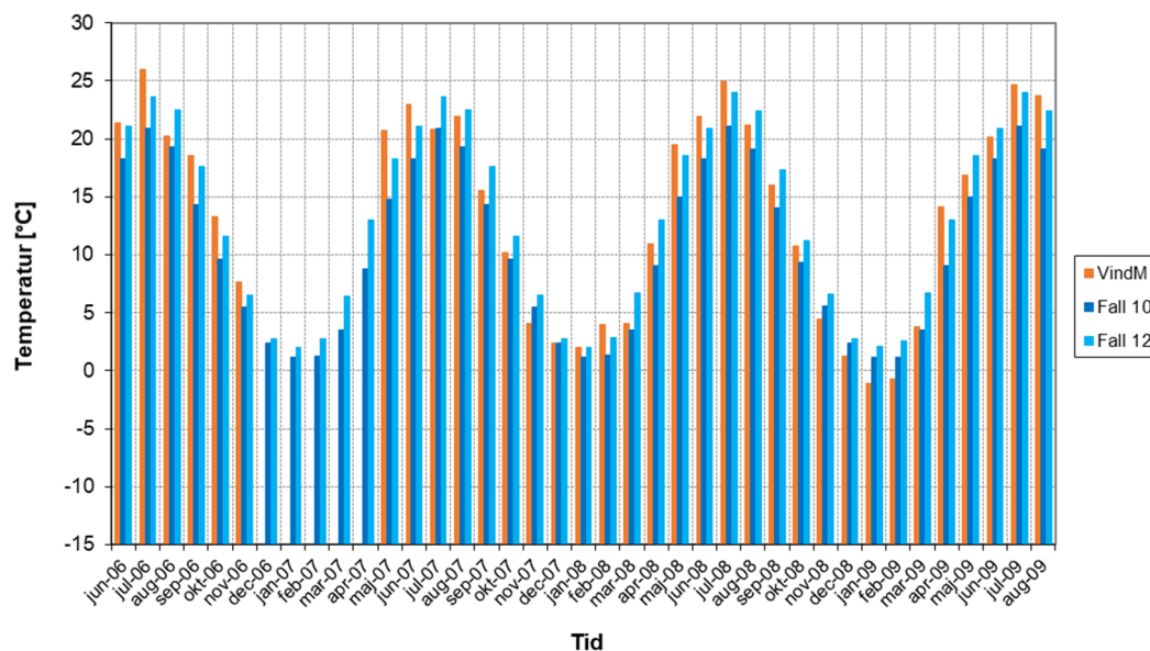
Figur 5.6 Jämförelse mellan uppmätta och beräknade månadsmedelvärden mot söder av temperaturen (°C) i vindsutrymme med diffusionsöppen underlagstäckning. Betydelsen av VindM framgår av tabell 3.1.
