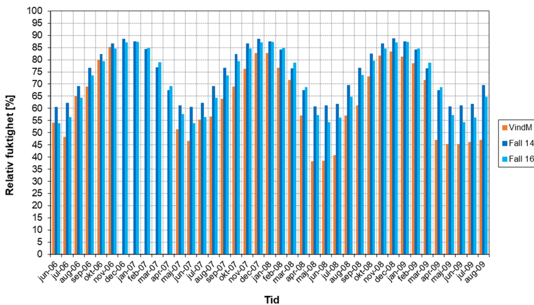
Figur 5.19 Jämförelse mellan uppmätta och beräknade månadsmedelvärden mot norr av relativ fuktighet (%) i vindsutrymme med diffusionsöppen underlagstäckning. Betydelsen av VindM framgår av tabell 3.1. I Fall 14 är antagen luftomsättning på vinden 2,75 oms/h medan den reducerats till 0,55 oms/h i Fall 16.
