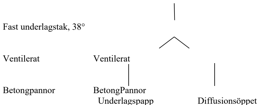
Figur 3.1 Försöksplan för mätningarna i provhuset i Lund.
