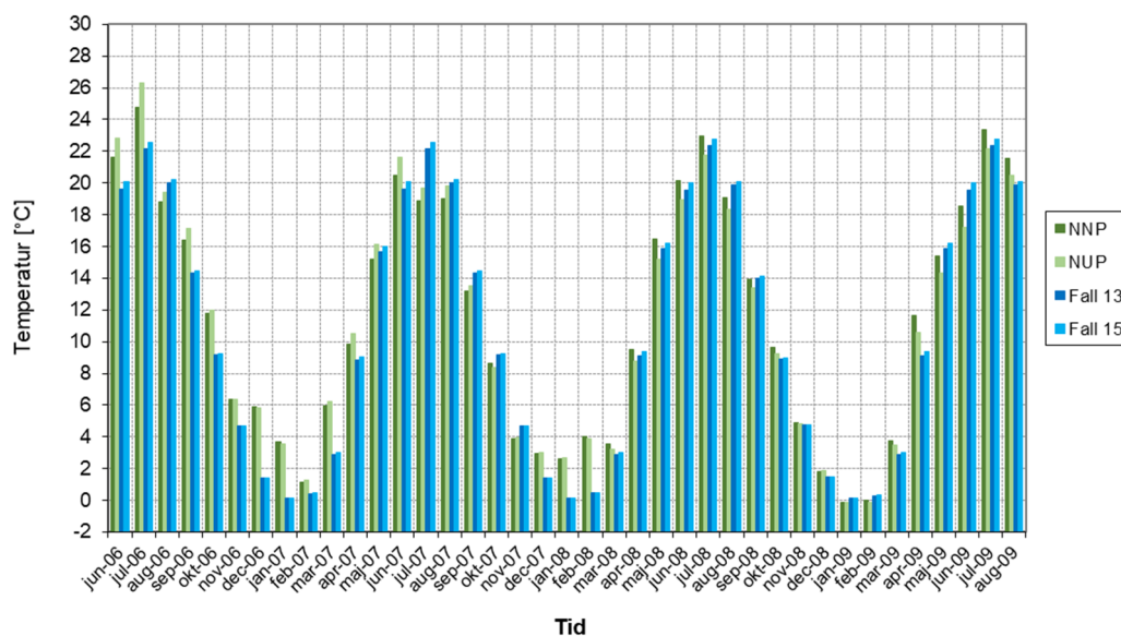
Figur 5.4 Jämförelse mellan uppmätta och beräknade månadsmedelvärden av temperaturen (°C) mot norr under takpannorna med traditionell underlagstäckning av papp. Betydelsen av NNP respektive NUP framgår av tabell 3.1.
