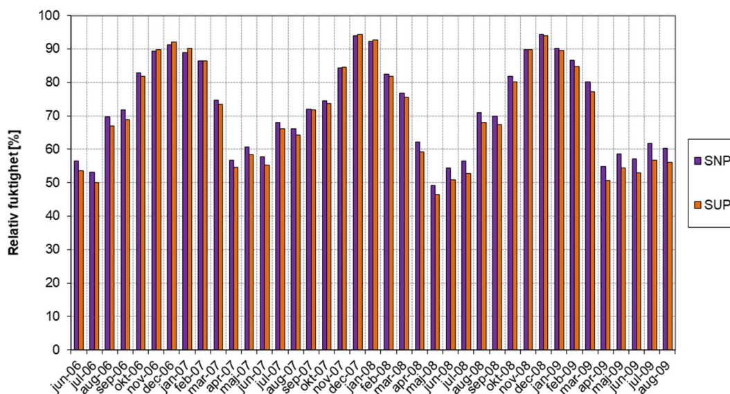
Figur 3.12 Månadsmedelvärden för relativ fuktighet (%) från två loggrar mot söder med traditionell underlagspapp på råsponten.
