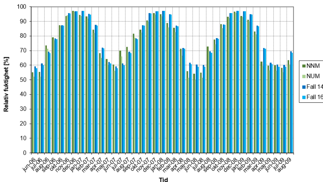
Figur 5.17 Jämförelse mellan uppmätta och beräknade månadsmedelvärden av relativ fuktighet (%) mot norr under takpannorna med diffusionsöppen underlagstäckning. Betydelsen av NNM respektive NUM framgår av tabell 3.1. I Fall 14 är antagen luftomsättning på vinden 2,75 oms/h medan den reducerats till 0,55 oms/h i Fall 16.
