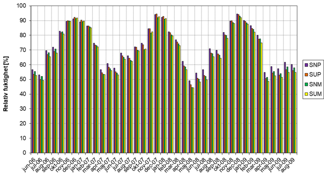
Figur 3.11 Månadsmedelvärden för relativ fuktighet (%) från samtliga fyra loggrar mot söder.
