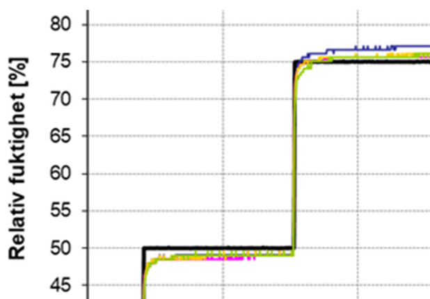
Figur 3.5 Förstorad del av figur 3.2 visar att tidskonstanten för givarna varierar något. Observera att samtliga givare visar något för låg RF vid 50 % medan de visar något för höga värden vid 75 % och därutöver.
