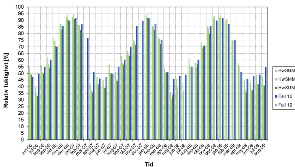
Figur 5.22 Jämförelse mellan uppmätta och beräknade månadsmedelvärden mot söder avseende relativ fuktighet (%) mellan råspont och diffusionsöppen underlagstäckning. Betydelsen av HwSNM, HwSMM och HwSUM framgår av tabell 3.3. I Fall 10 är antagen luftomsättning på vinden 2,75 oms/h medan den reducerats till 0,55 oms/h i Fall 12.
