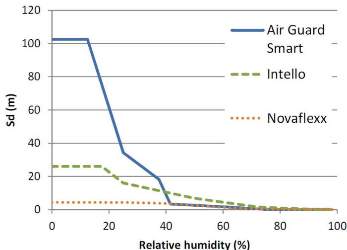
Figur 2.6 S_d -värde som funktion av den relativa fuktigheten för tre av ångbromsarna, (Geving & Thorsrud, 2014). Detaljerade mätningar för Hygrodioid 200A fanns inte tillgängliga.
