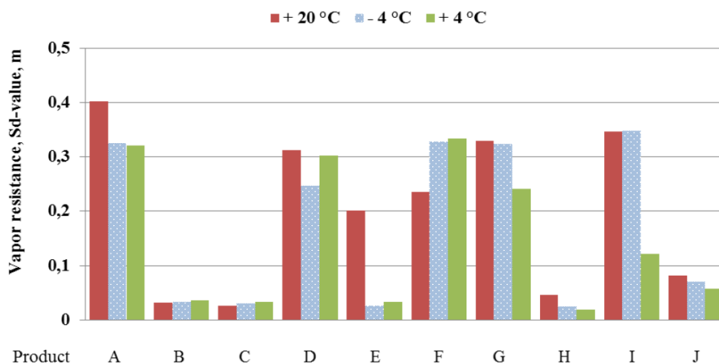
Figur 2.9 Uppmätta S_d värde för de tio olika underlagstäckningarna, (Uvsløkk, Vågen & Korsnes, 2014).
