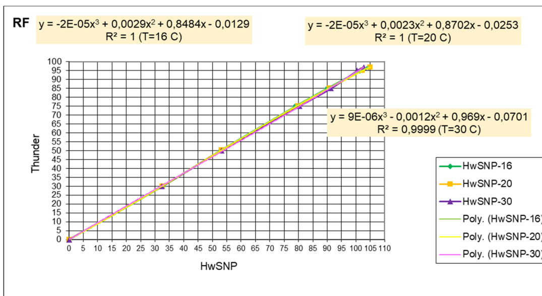
Figur. 3.3 Exempel på resultat från kalibrering avseende relativ fuktighet med inlagda polynomfunktioner för temperaturerna +16 °, +20 °C och +30 °C. Som framgår av ekvationerna går dessa nästan genom origo om RF är noll. Även om skillnaderna vid olika temperatur är liten har linjär interpolering med hänsyn till temperaturen vid varje mät-tillfälle ändå beaktats.
