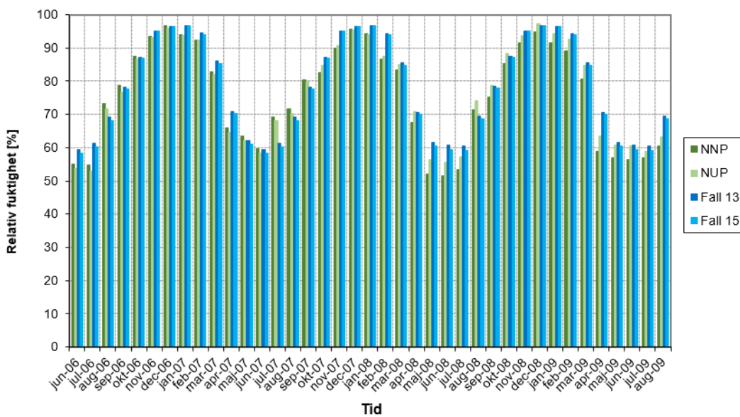
Figur 5.16 Jämförelse mellan uppmätta och beräknade månadsmedelvärden av relativ fuktighet (%) mot norr under takpannorna med traditionell underlagstäckning av papp. Betydelsen av NNP respektive NUP framgår av tabell 3.1. I Fall 13 är antagen luftomsättning på vinden 2,75 oms/h medan den reducerats till 0,55 oms/h i Fall 15.
