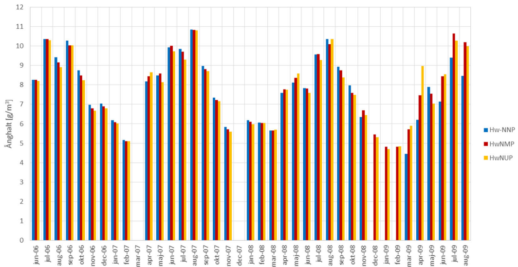
Figur 3.57 Månadsmedelvärde för ånghalt ( \text{g/m}^3 ) avseende de tre sensorerna mot norr mellan råspont och underlagstäckning av papp.
