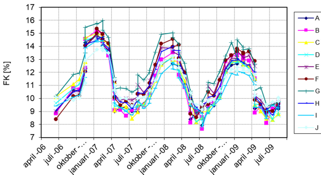
Figur 3.25 Uppmätt och temperaturkorrigerad fuktkvot (%) på vinden. Samtliga mät-punkter (A-J).
