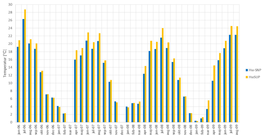
Figur 3.37 Månadsmedeltemperaturer från två sensorer mot söder med traditionell underlagspapp på råsponten.
