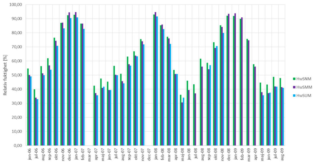
Figur 3.47 Månadsmedelvärden för relativ fuktighet (%) från tre sensorer mot söder med ånggenomsläppligt material på råsponen.
