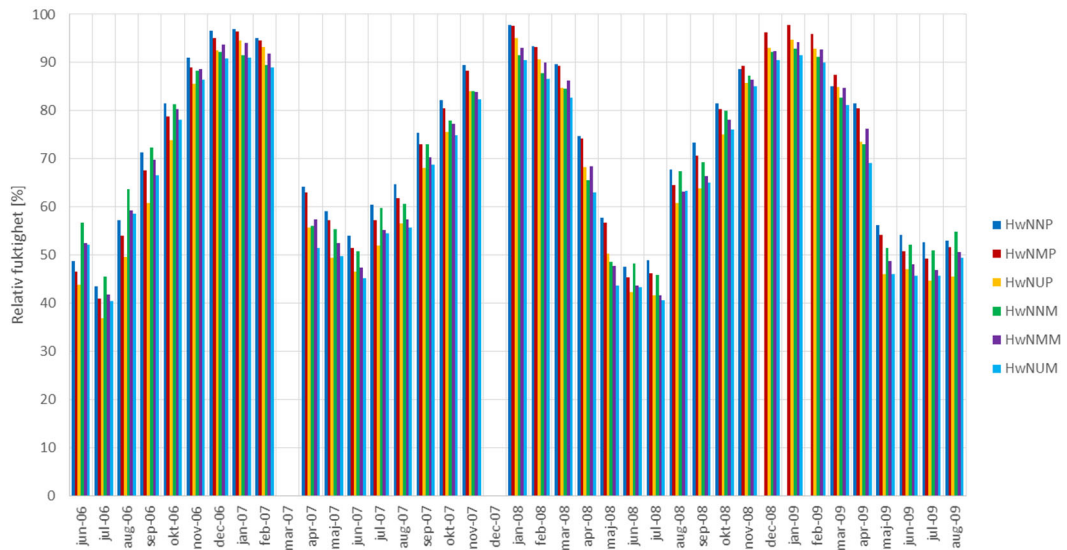
Figur 3.48 Månadsmedelvärden för relativ fuktighet (%) från samtliga sex sensorer mot norr.
