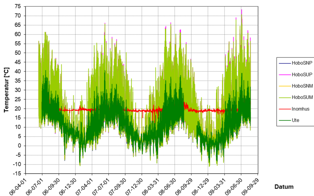
Figur 3.6 Temperatur för samtliga loggrar mot söder samt inne och ute.
