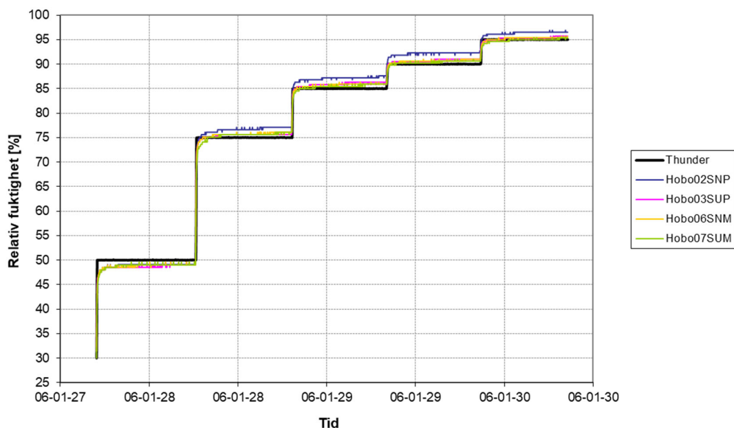
Figur 3.4 Exempel på resultat från kalibrering i precisionsfuktkammaren vid LTH. Som framgår av figuren är det alltid en viss fördröjning i förändring av RF hos givarna efter en omedelbar stegändring av RF i precisionsfuktkammaren vid konstant temperatur (Thunder, svart linje).
