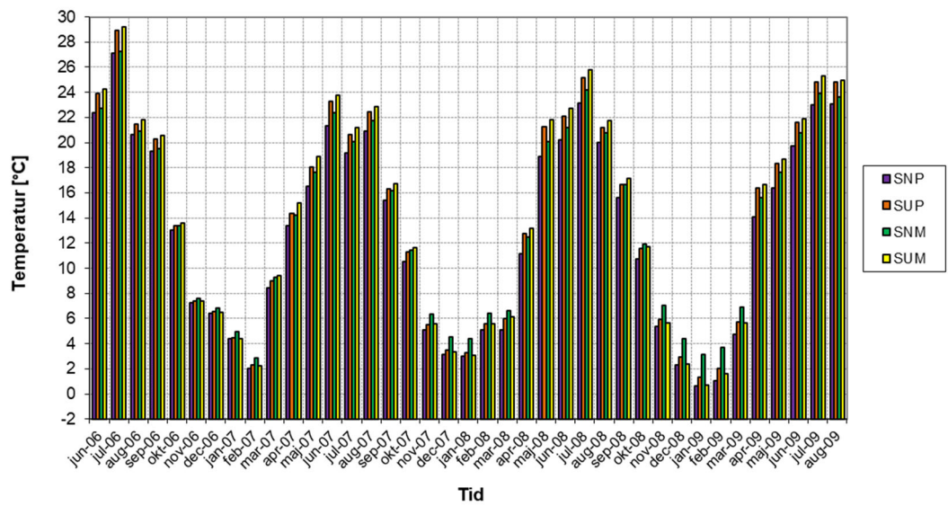
Månadsmedelvärde - temperatur, juni-06 – augusti-09
