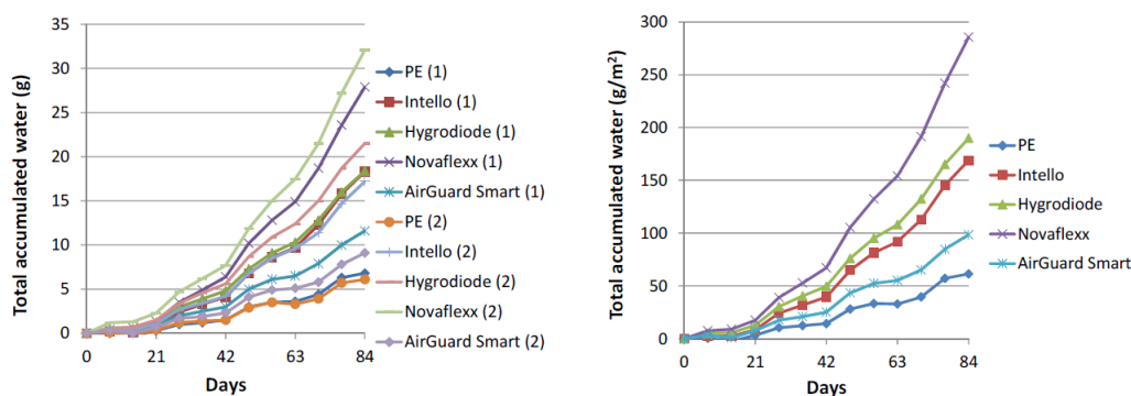
Figur 2.7 Total ackumulerad fukt mängd i samband med de fem olika försöksuppställningarna. Till vänster visas alla tio försöken (med två uppställningar per configuration). Till höger visas medelvärdet av de fem uppställningarna, (Geving & Thorsrud, 2014).
