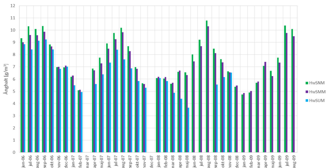
Figur 3.55 Månadsmedelvärde för ånghalt ( \text{g}/\text{m}^3 ) avseende de tre sensorerna mot söder mellan råspont och underlagstäckning av diffusionsöppen produkt.
