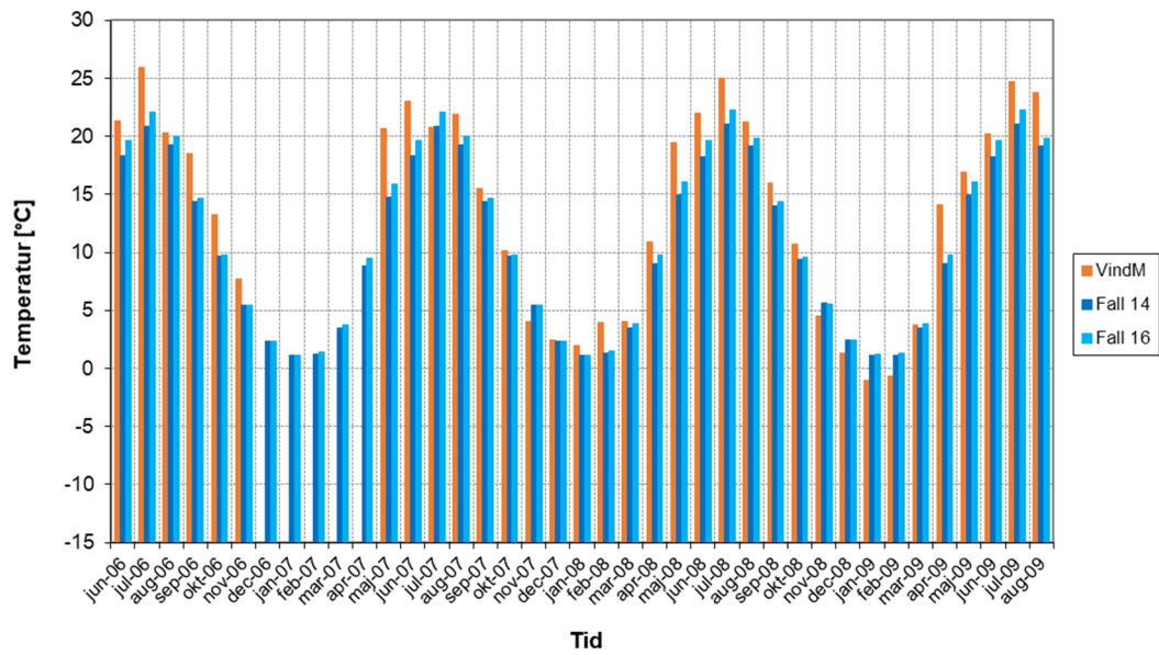
Figur 5.7 Jämförelse mellan uppmätta och beräknade månadsmedelvärden mot norr av temperaturen (°C) i vindsutrymme med diffusionsöppen underlagstäckning. Betydelsen av VindM framgår av tabell 3.1.
