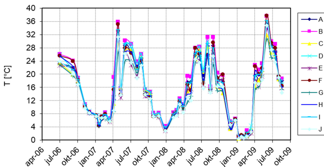
Figur 3.28 Uppmätt temperatur (°C) i trä på vinden. Samtliga mätpunkter (A-J).
