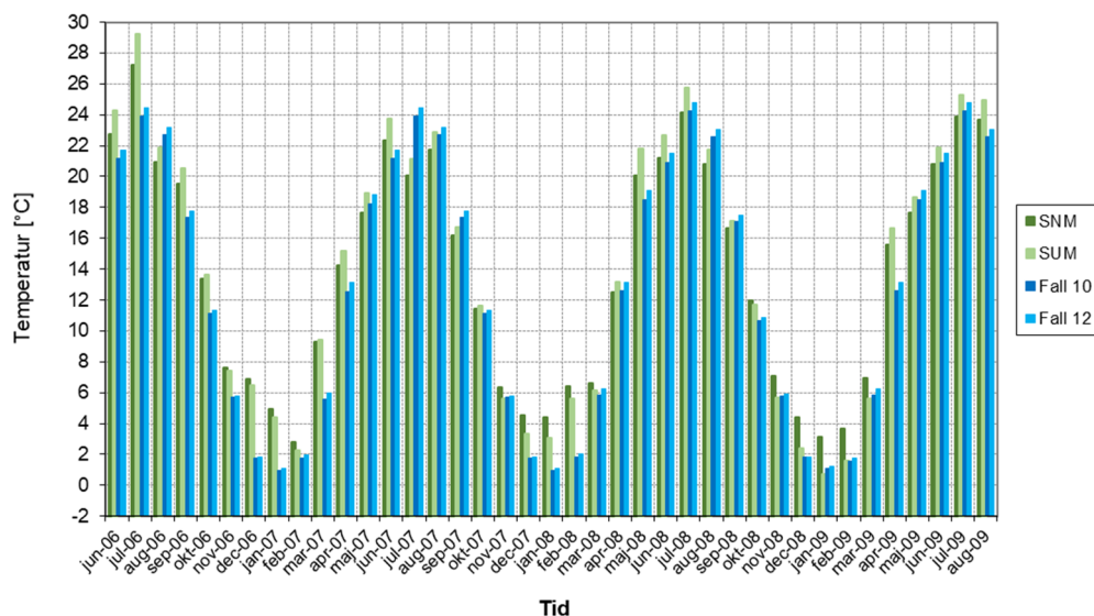
Figur 5.3 Jämförelse mellan uppmätta och beräknade månadsmedelvärden av temperaturen (°C) mot söder under takpannorna med diffusionsöppen underlagstäckning. Betydelsen av SNM respektive SUM framgår av tabell 3.1.
