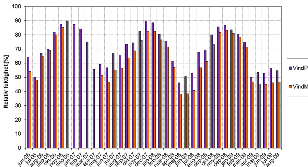
Figur 3.17 Månadsmedelvärden för relativ fuktighet (%) från de två loggrar som var placerade i de kalla vindsutrymmena.
