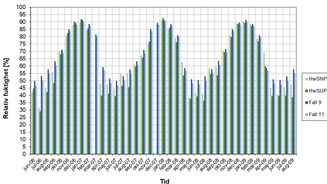
Figur 5.24 Jämförelse mellan uppmätta och beräknade månadsmedelvärden mot söder avseende relativ fuktighet (%) mellan råspont och traditionell underlagstäckning av papp. Betydelsen av HwSNP och HwSUP framgår av tabell 3.3. I Fall 9 är antagen luftomsättning på vinden 2,75 oms/h medan den reducerats till 0,55 oms/h i Fall 11.
