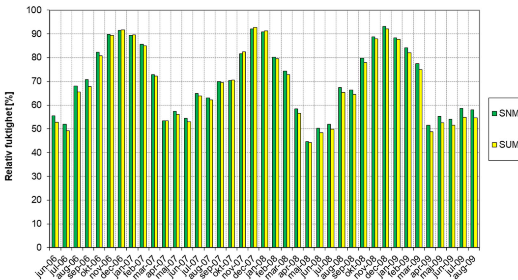
Figur 3.13 Månadsmedelvärden för relativ fuktighet (%) från två loggrar mot söder med ånggenomsläppligt ytskikt på råsponten.
