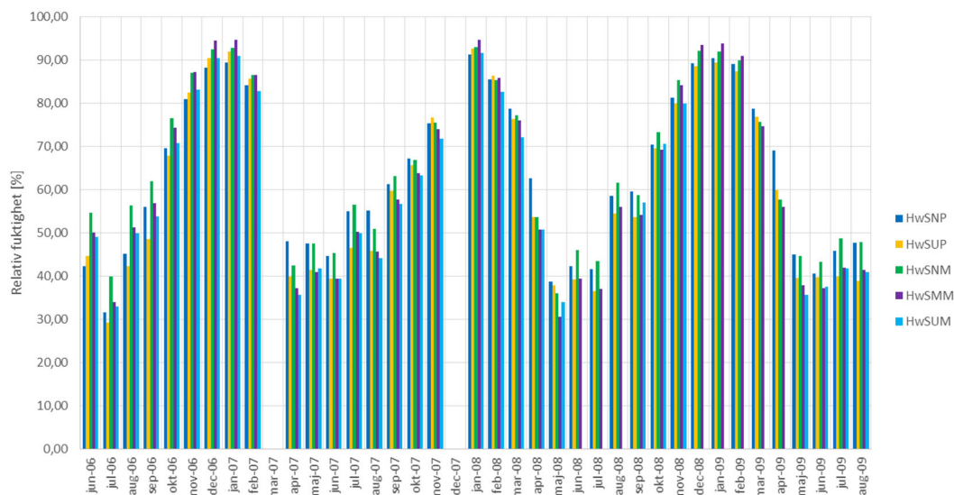
Figur 3.45 Månadsmedelvärden för relativ fuktighet (%) från samtliga fem sensorer mot söder.
