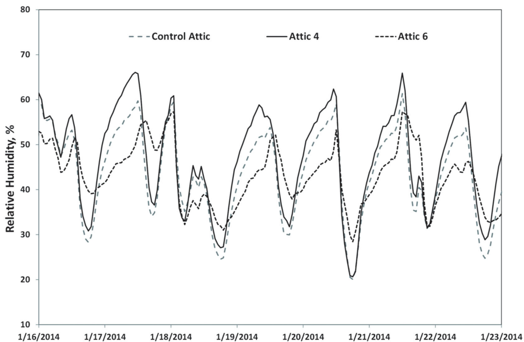
Figur 2.4 Uppmätt relativ fuktighet i de tre undersökta vindsutrymmena under perioden 16-23 januari 2014, (Shiao et al, 2016).
