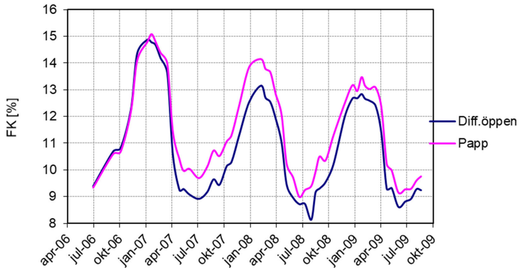
Figur 3.29 Uppmätt temperaturkorrigerad fuktkvot (%) på vinden. Medelvärde för de två vindshalvorna med diffusionsöppet respektive traditionell underlagspapp.
