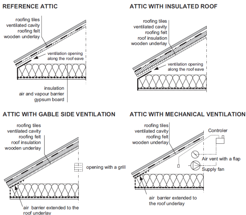
Figur 2.1 Sektioner av de fyra simulerade takkonstruktionerna ventilerade med utomhusluft, (Nik et al,2012).
