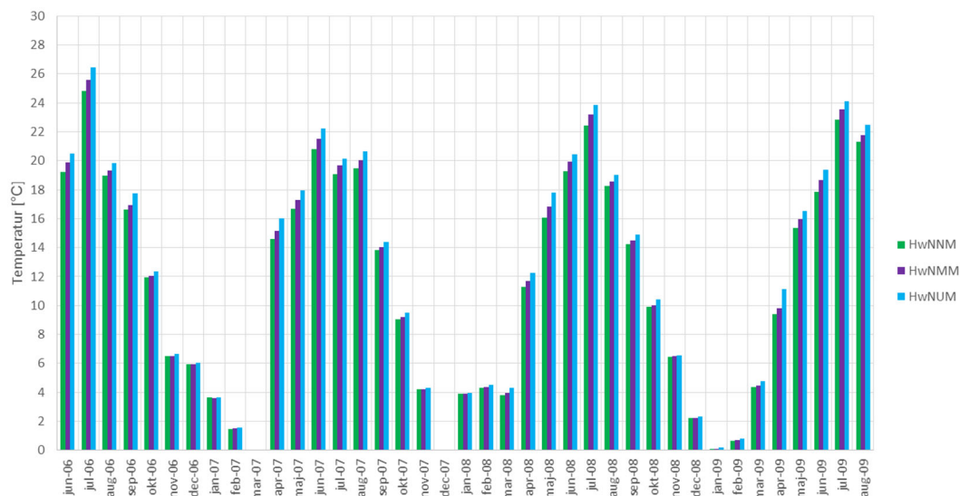
Figur 3.41 Månadsmedeltemperaturer från tre sensorer mot norr med diffusionsöppen underlagstäckning på råsponten.
