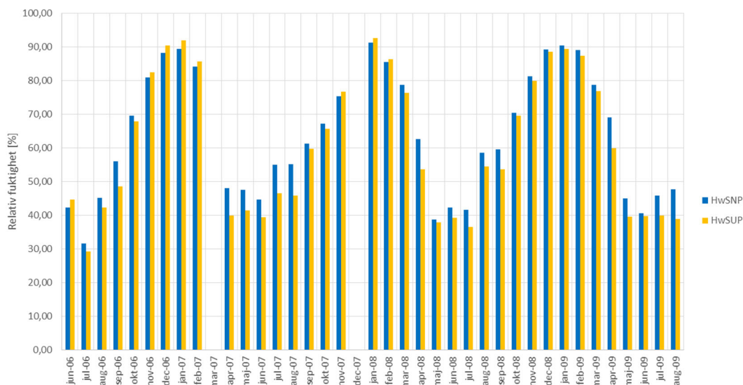
Figur 3.46 Månadsmedelvärden för relativ fuktighet (%) från två sensorer mot söder med traditionell underlagspapp på råsponten.
