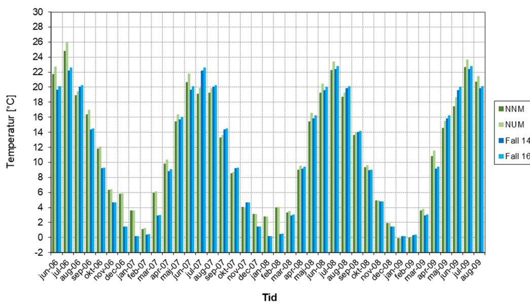
Figur 5.5 Jämförelse mellan uppmätta och beräknade månadsmedelvärden av temperaturen (°C) mot norr under takpannorna med diffusionsöppen underlagstäckning. Betydelsen av NNM respektive NUM framgår av tabell 3.1.
