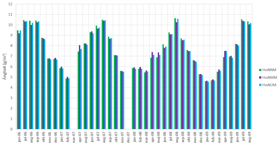
Figur 3.58 Månadsmedelvärde för ånghalt ( \text{g/m}^3 ) avseende de tre sensorerna mot norr mellan råspont och underlagstäckning av diffusionsöppen produkt.
