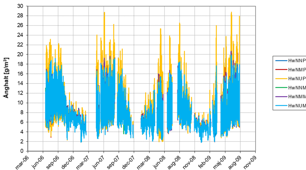
Figur 3.52 Ånghalt ( \text{g/m}^3 ) från samtliga sex sensorer mot norr mellan råspont och underlagstäckning.
