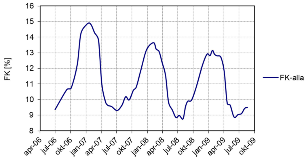
Figur 3.32 Uppmätt temperaturkorrigerad fuktkvot (%) på vinden. Medelvärde för samtliga mätpunkter (A-J).
