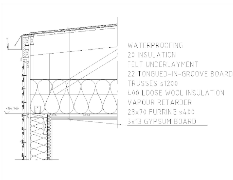
Figur 2.10 Sektion av taket i den undersökta byggnaden i Borås, (Kurkinen, 2014).
