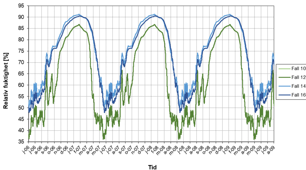
Figur 5.26 Beräknad relativ fuktighet (%) i råsponten med diffusionsöppet underlagstak. I Fall 10 och 14 är luftomsättningen 2,75 oms/h. För Fall 12 och 16 är luftomsättningen 0,55 oms/h. Fall 10 och 12 är orienterade mot söder medan Fall 14 och 16 är riktade mot norr.
