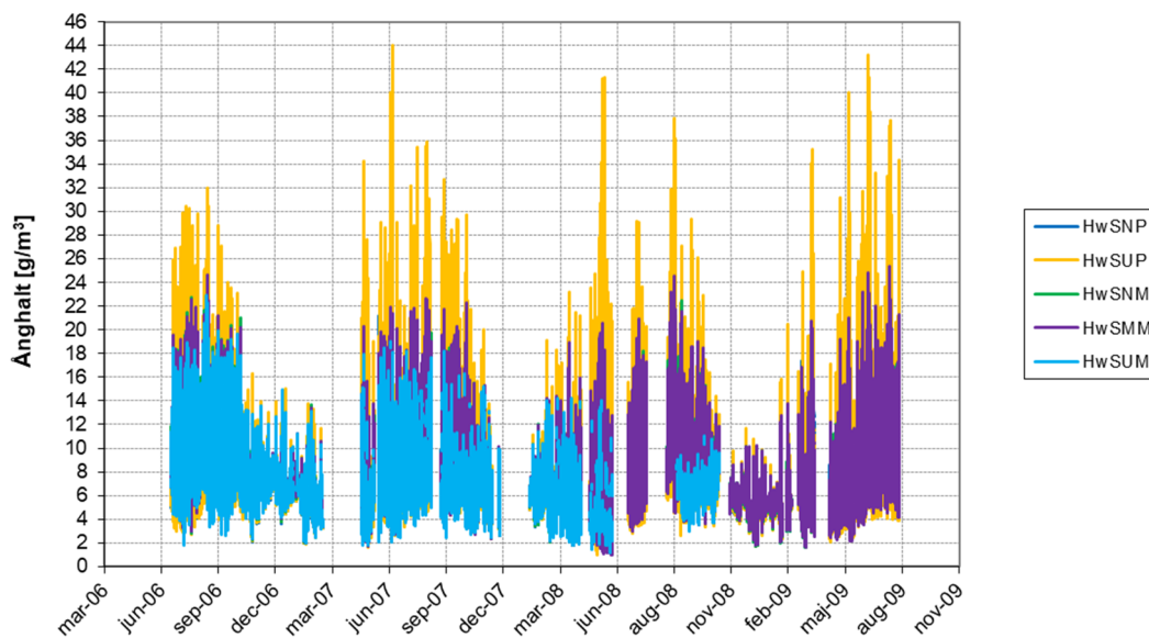
Figur 3.51 Ånghalt ( \text{g/m}^3 ) från samtliga fem sensorer mot söder mellan råspont och underlagstäckning.
