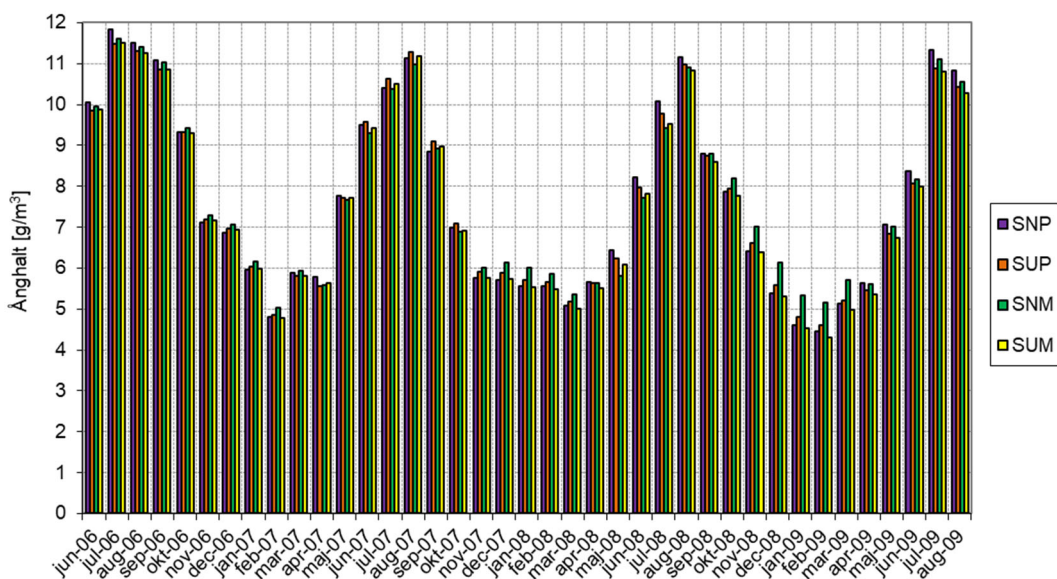
Figur 3.18 Månadsmedelvärden för ånghalt ( \text{g/m}^3 ) från samtliga fyra loggrar mot söder.
