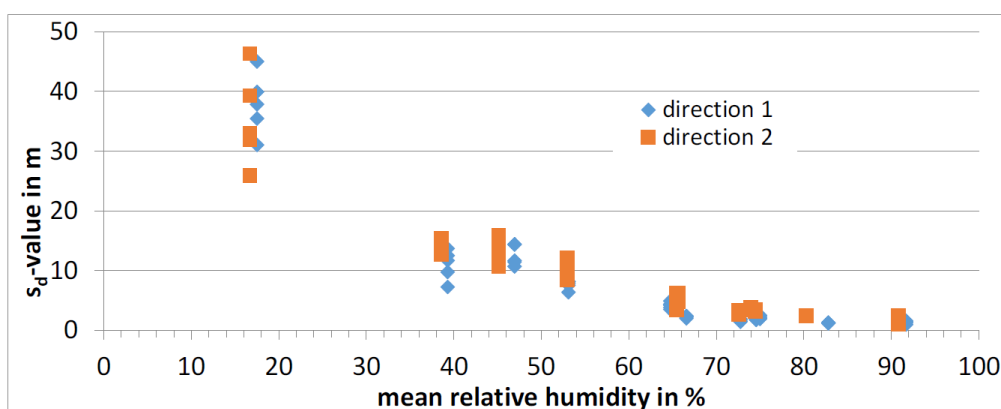
Figur 2.14 Uppmäta S d - värde för produkt A, (Fechner och Meißner, 2017).
