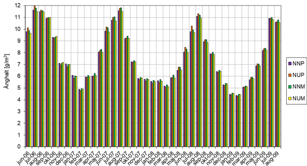
Figur 3.21 Månadsmedelvärden för ånghalt ( \text{g/m}^3 ) från samtliga fyra loggrar mot norr.
