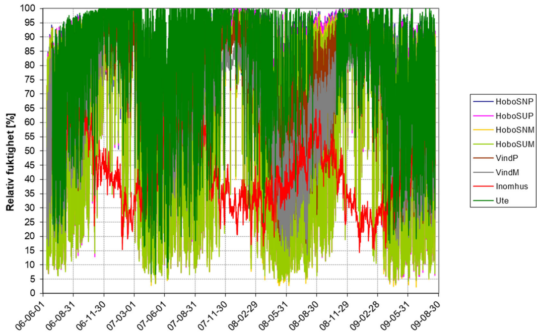
Figur 3.10 Relativ fuktighet (%) från samtliga loggrar mot söder, på vindarna samt inne och ute.
