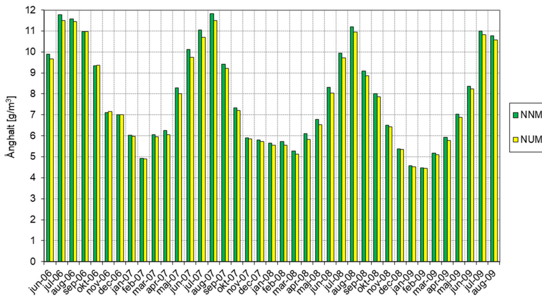
Figur 3.23 Månadsmedelvärden för ånghalt ( \text{g/m}^3 ) från de två loggrar mot norr som fanns ovanför takdelen med ånggenomsläppligt ytskikt på råsponten.
