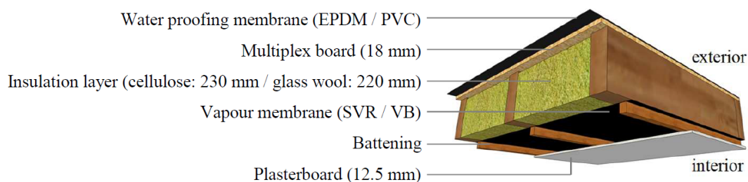
Figur 2.17 Principiell uppbyggnad av de kompakta takelementen, (Langerocka et al, 2017).
