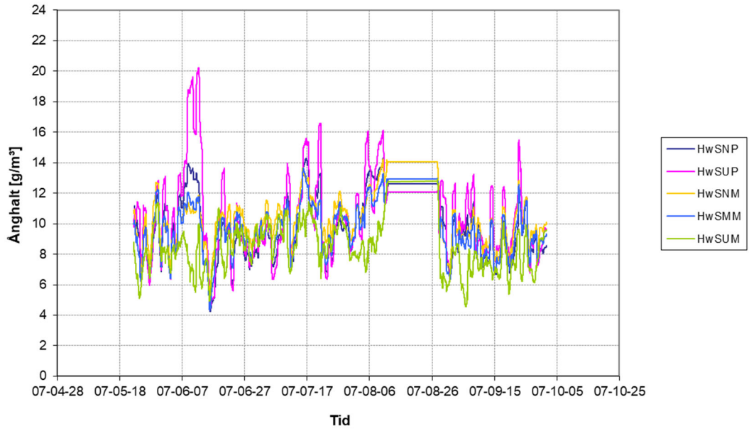
Provhuset - tak, Honeywell Söder Glidande dygnsmedelvärde 070521-071001
