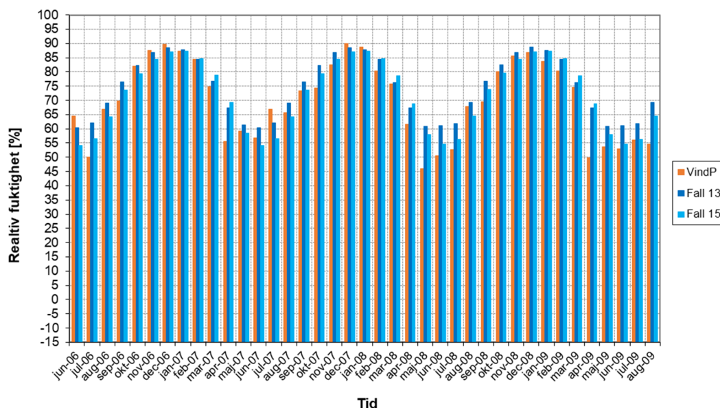
Figur 5.21 Jämförelse mellan uppmätta och beräknade månadsmedelvärden mot norr av relativ fuktighet (%) i vindsutrymme med traditionell underlagstäckning av papp. Betydelsen av VindP framgår av tabell 3.1. I Fall 13 är antagen luftomsättning på vinden 2,75 oms/h medan den reducerats till 0,55 oms/h i Fall 15.
