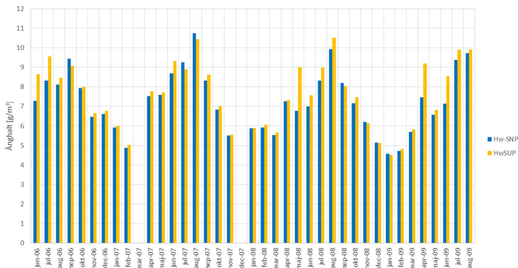
Figur 3.54 Månadsmedelvärde för ånghalt ( \text{g}/\text{m}^3 ) avseende de två sensorerna mot söder mellan råspont och underlagstäckning av papp.
