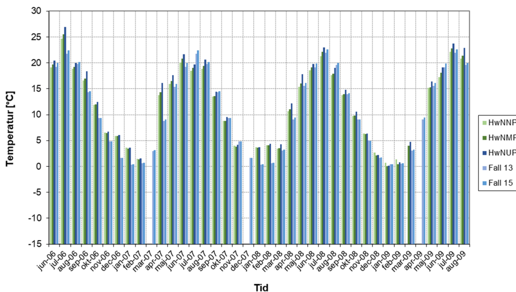
Figur 5.13 Jämförelse mellan uppmätta och beräknade månadsmedelvärden mot norr avseende temperaturen (°C) mellan råspont och traditionell underlagstäckning av papp. Betydelsen av HwNNP, HwNMP och HwNUP framgår av tabell 3.3. I Fall 13 är antagningen luftomsättning på vinden 2,75 oms/h medan den reducerats till 0,55 oms/h i Fall 15.
