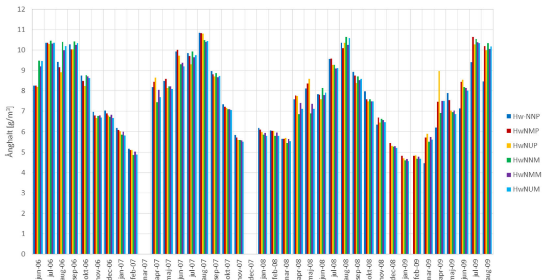
Figur 3.56 Månadsmedelvärde för ånghalt ( \text{g}/\text{m}^3 ) avseende samtliga sex sensorer mot norr mellan råspont och underlagstäckning.
