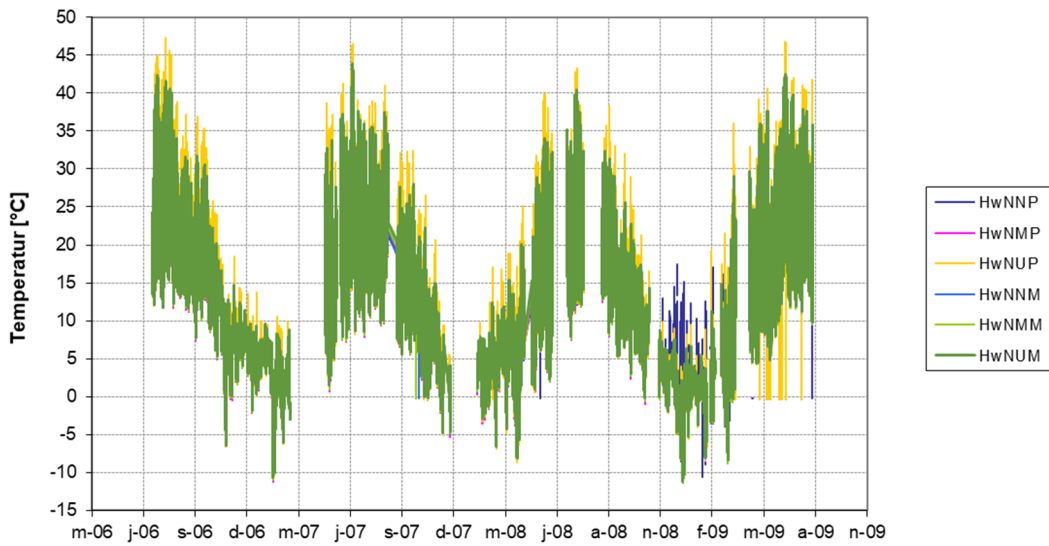
Figur 3.35 Temperatur för samtliga sensorer mot norr.
