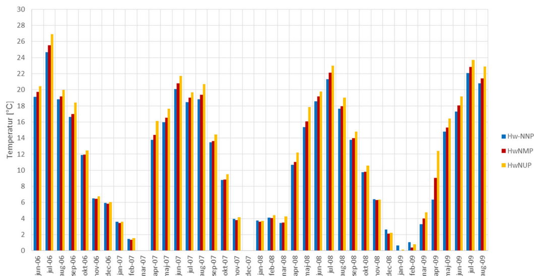
Figur 3.40 Månadsmedeltemperaturer från tre sensorer mot norr med traditionell underlagspapp på råsponten.
