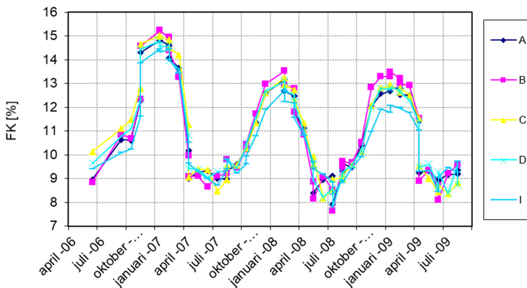
Figur 3.26 Uppmätt och temperaturkorrigerad fuktkvot (%) på vinden. Endast mät-punkter från vindsdelen med diffusionsöppen underlagstäckning på råsPonten, dvs. A-D samt I.
