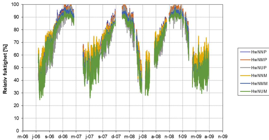
Figur 3.44 Relativ fuktighet för samtliga sensorer mot norr.
