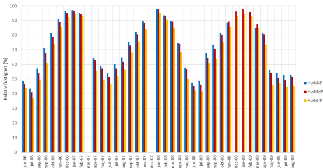
Figur 3.49 Månadsmedelvärden för relativ fuktighet (%) från tre sensorer mot norr med traditionell underlagspapp på råsponten.
