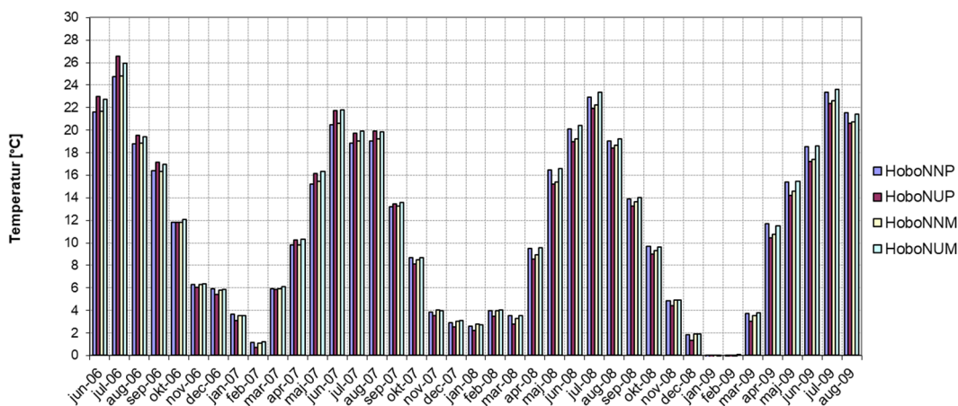
Figur 3.9 Månadsmedeltemperaturer mot norr mellan underlagstäckning och takpannor av betong.
