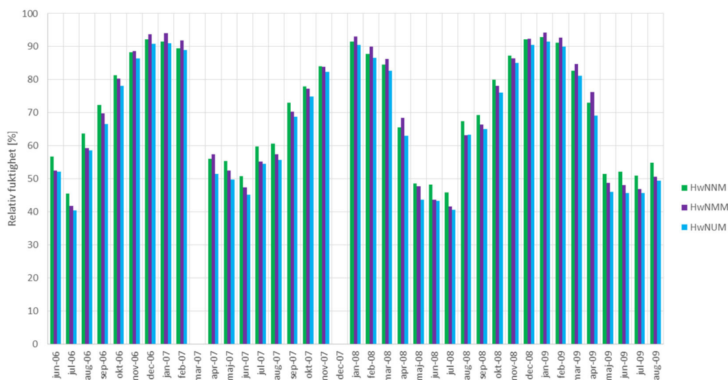
Figur 3.50 Månadsmedelvärden för relativ fuktighet (%) från tre sensorer mot norr med ånggenomsläppligt material på råsponten.
