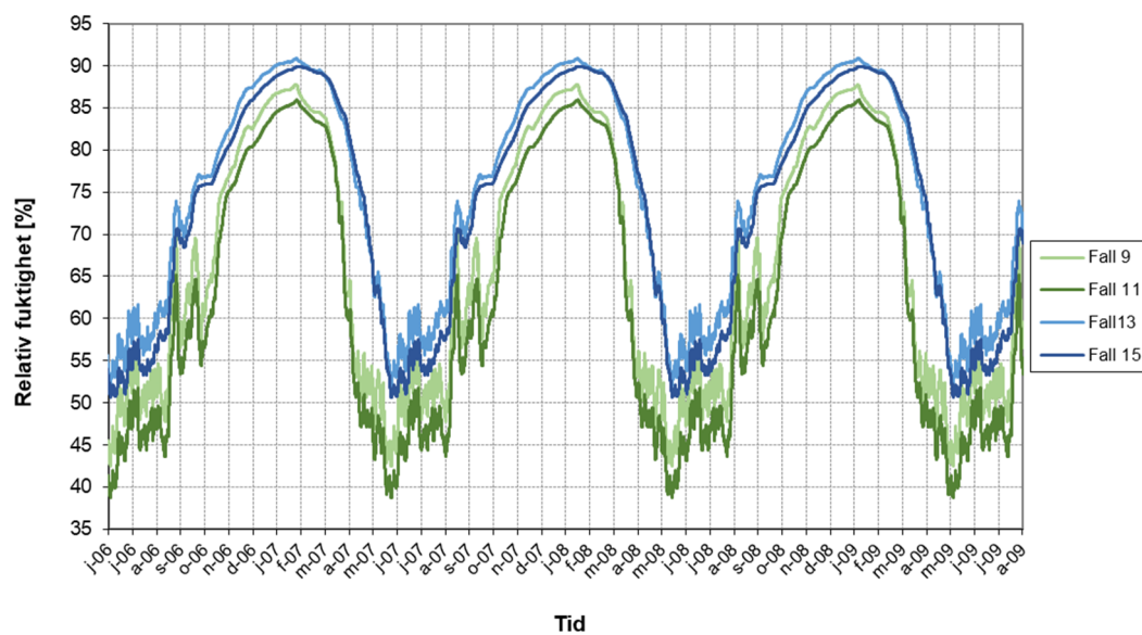
Figur 5.27 Beräknad relativ fuktighet (%) i råsponten med traditionellt underlagstak av underlagspapp. I Fall 9 och 13 är luftomsättningen 2,75 oms/h. För Fall 11 och 15 är luftomsättningen 0,55 oms/h. Fall 9 och 11 är orienterade mot söder medan Fall 13 och 15 är riktade mot norr.
