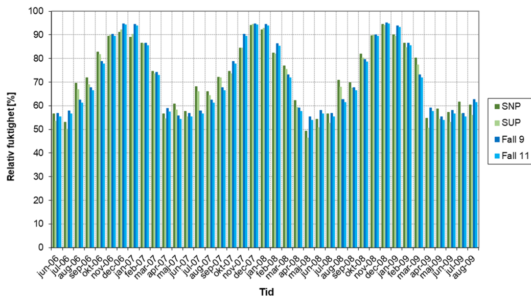
Figur 5.14 Jämförelse mellan uppmätta och beräknade månadsmedelvärden av relativ fuktighet (%) mot söder under takpannorna med traditionell underlagstäckning av papp. Betydelsen av SNP respektive SUP framgår av tabell 3.1. I Fall 9 är antagen luftomsättning på vinden 2,75 oms/h medan den reducerats till 0,55 oms/h i Fall 11.
