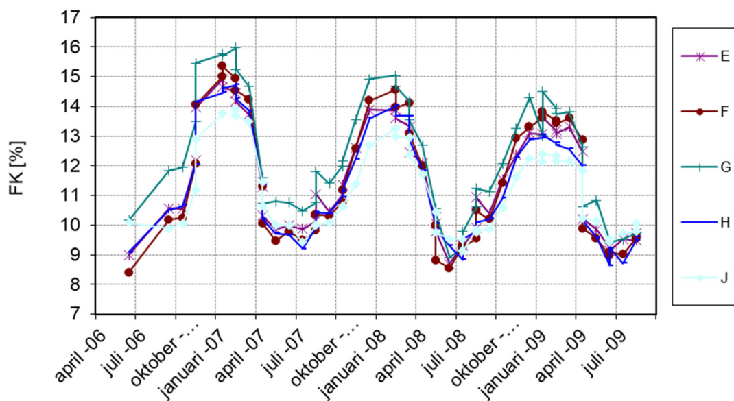
Figur 3.27 Uppmätt och temperaturkorrigerad fuktkvot (%) på vinden. Endast mät-punkter från vindsdelen med traditionell underlagspapp på råsponten, dvs. E-H samt J.
