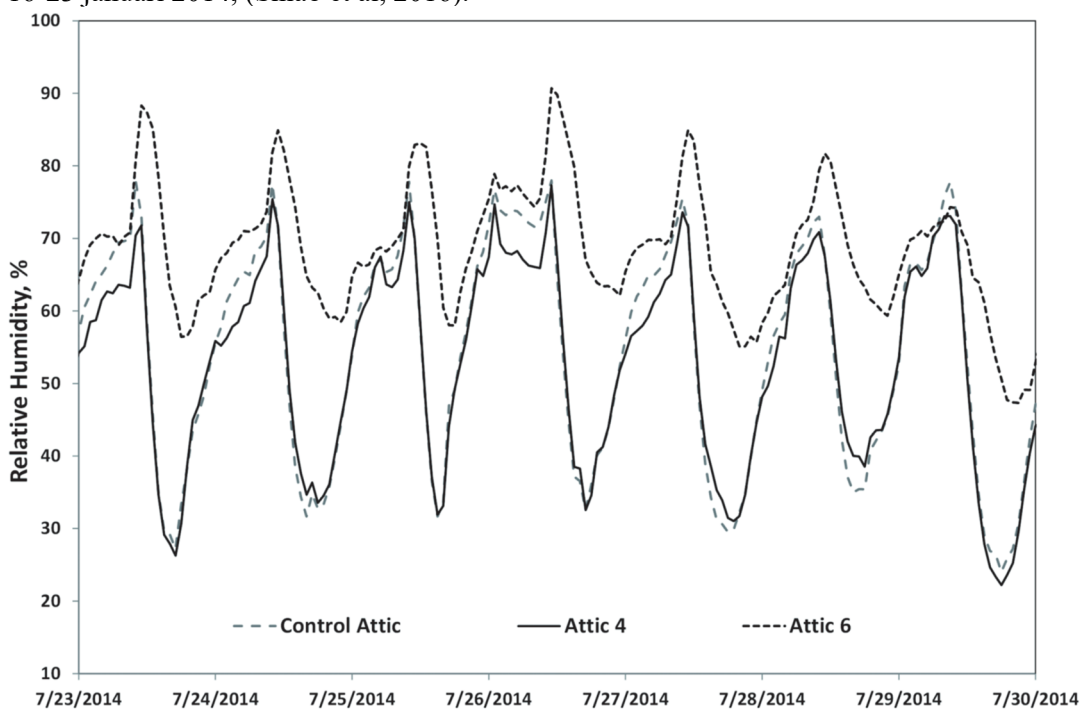
Figur 2.5 Uppmätt relativ fuktighet i de tre undersökta vindsutrymmena under perioden 23-30 juli 2014, (Shiao et al, 2016).
