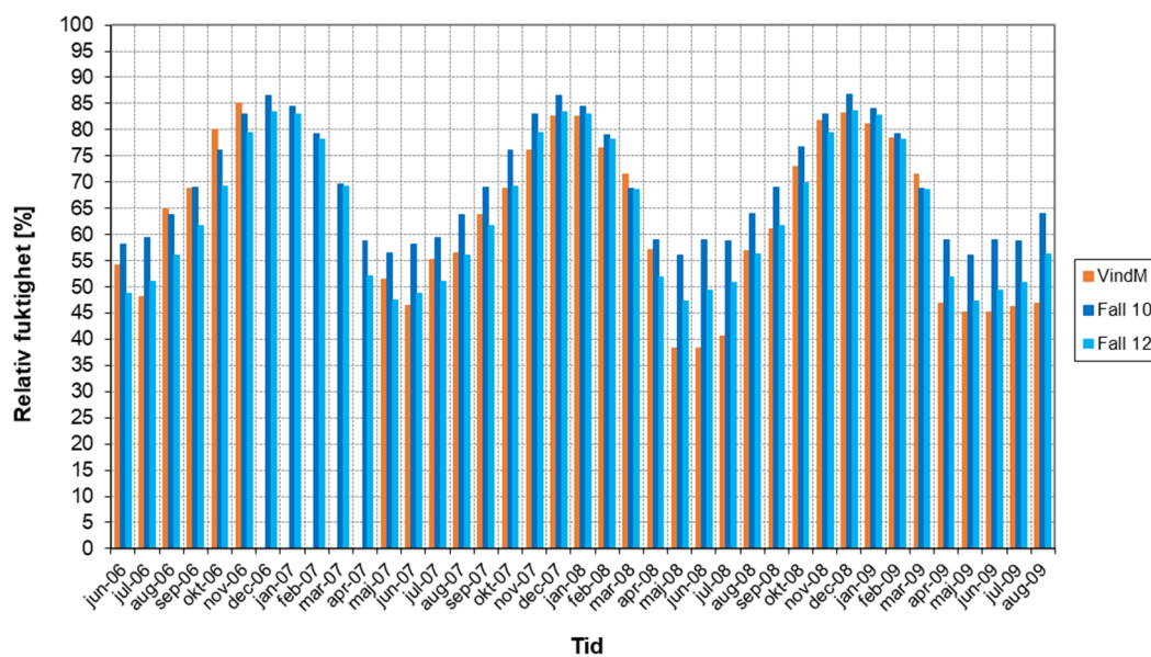
Figur 5.18 Jämförelse mellan uppmätta och beräknade månadsmedelvärden mot söder av relativ fuktighet (%) i vindsutrymme med diffusionsöppen underlagstäckning. Betydelsen av VindM framgår av tabell 3.1. I Fall 10 är antagen luftomsättning på vinden 2,75 oms/h medan den reducerats till 0,55 oms/h i Fall 12.
