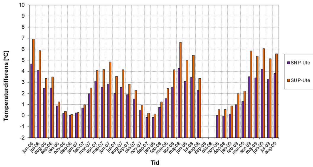
Månadsmedelvärde - temperaturdifferens, juni-06 – augusti-09
