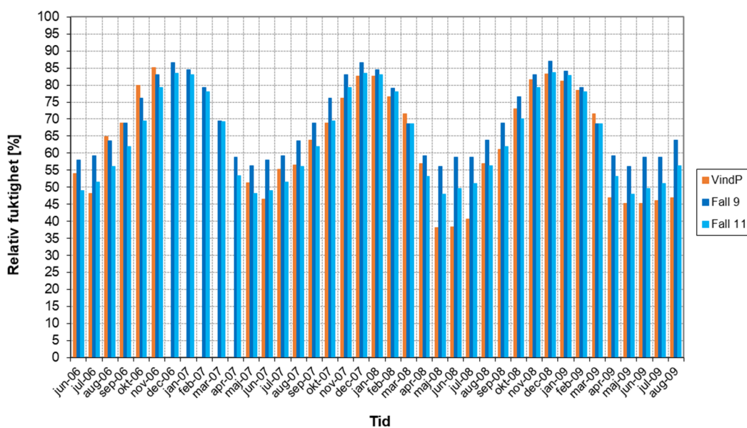
Figur 5.20 Jämförelse mellan uppmätta och beräknade månadsmedelvärden mot söder av relativ fuktighet (%) i vindsutrymme med traditionell underlagstäckning av papp. Betydelsen av VindP framgår av tabell 3.1. I Fall 9 är antagen luftomsättning på vinden 2,75 oms/h medan den reducerats till 0,55 oms/h i Fall 11.
