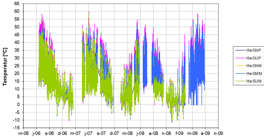
Figur 3.34 Temperatur för samtliga sensorer mot söder.
