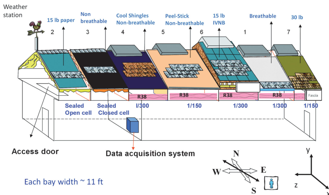
Figur 2.3 Beskrivning av de olika vindsutrymmena som ingår i försöket (Shiao et al, 2016).
