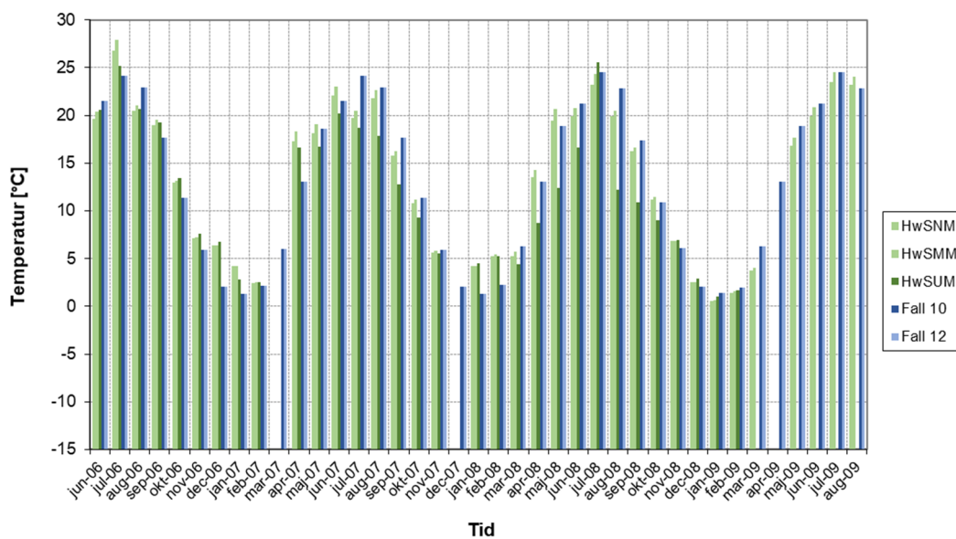
Figur 5.10 Jämförelse mellan uppmätta och beräknade månadsmedelvärden mot söder avseende temperaturen (°C) mellan råspond och diffusionsöppen underlagstäckning. Betydelsen av HwSNM, HwSMM och HwSUM framgår av tabell 3.3. I Fall 10 är antagen luftomsättning på vinden 2,75 oms/h medan den reducerats till 0,55 oms/h i Fall 12.
