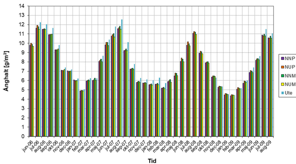
Månadsmedelvärde – ånghalt, juni-06 – augusti-09
