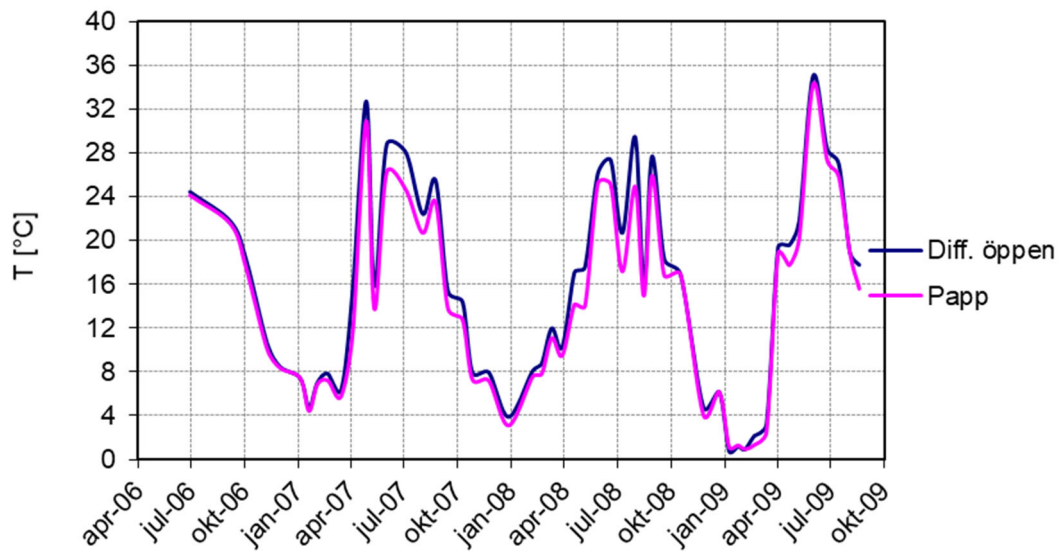
Figur 3.30 Uppmätt temperatur (°C) i trä på vinden. Medelvärde för de två vindshalvorna med diffusionsöppet respektive traditionell underlagspapp.
