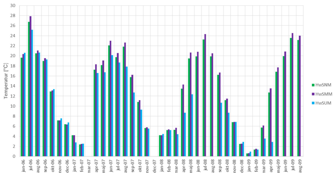
Figur 3.38 Månadsmedeltemperaturer från tre sensorer mot söder med diffusionsöppen underlagstäckning på råsponten.
