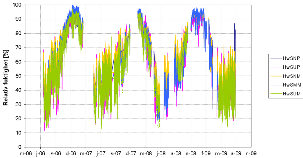
Figur 3.42 Relativ fuktighet för samtliga sensorer mot söder.
