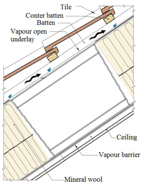
Figur 2.8 Sektionsskiss av ett tak. Plastlådorna som användas i försöken är markerad för att illustrera vilken del av taket som är simulerades i experimenten, (Uvsløkk, Vågen & Korsnes, 2014).
