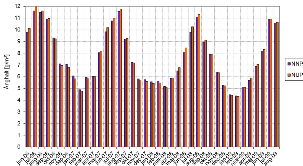
Figur 3.22 Månadsmedelvärden för ånghalt ( \text{g/m}^3 ) från de två loggrar mot norr som fanns ovanför takdelen med traditionell underlagspapp på råsponten.
