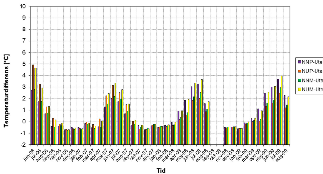
Månadsmedelvärde - temperaturdifferens, juni-06 – augusti-09
