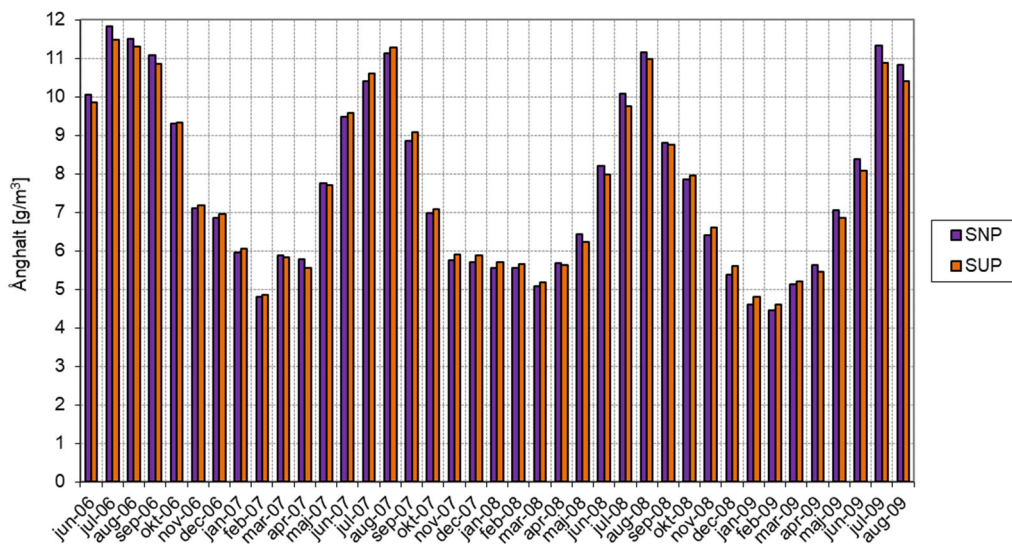
Figur 3.19 Månadsmedelvärden för ånghalt ( \text{g/m}^3 ) från de två loggrar mot söder som fanns ovanför takdelen med traditionell underlagspapp på råsponten.
