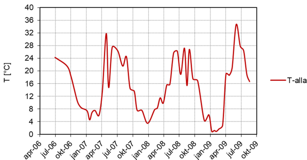
Figur 3.33 Uppmätt temperatur (°C) på vinden. Medelvärde för samtliga mätpunkter (A-J).
