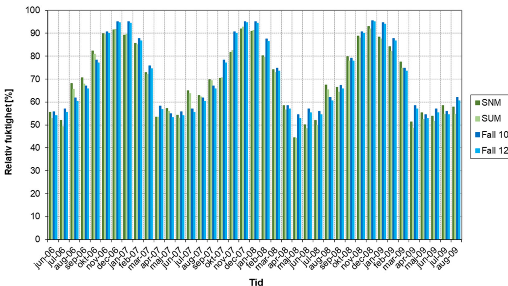
Figur 5.15 Jämförelse mellan uppmätta och beräknade månadsmedelvärden av relativ fuktighet (%) mot söder under takpannorna med diffusionsöppen underlagstäckning. Betydelsen av SNM respektive SUM framgår av tabell 3.1. I Fall 10 är antagen luftomsättning på vinden 2,75 oms/h medan den reducerats till 0,55 oms/h i Fall 12.
