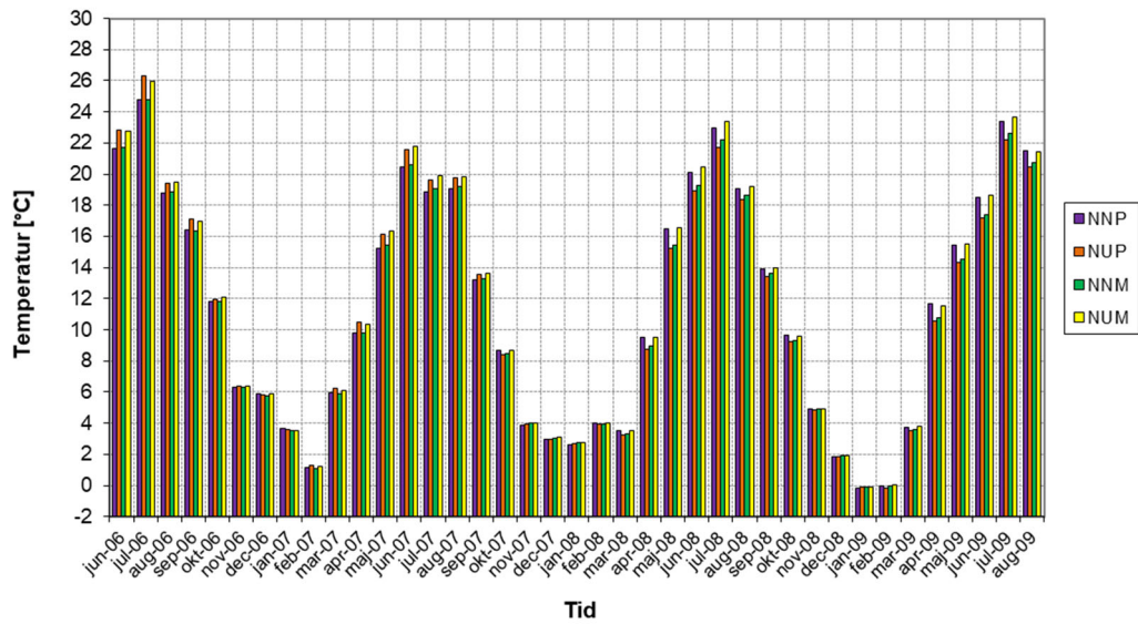
Månadsmedelvärde - temperatur, juni-06 – augusti-09
