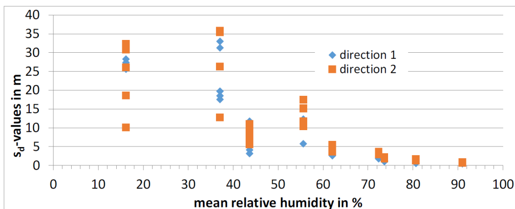
Figur 2.15 Uppmätta S_d - värde för produkt B, (Fechner och Meißner, 2017).
