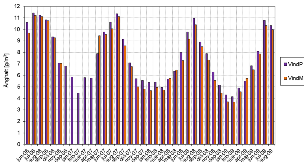
Figur 3.24 Månadsmedelvärden för ånghalt ( \text{g/m}^3 ) från de två loggrar som var placerade i de kalla vindsutrymmena.
