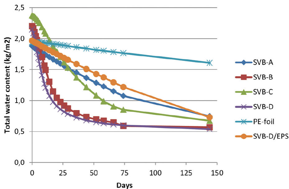
Figur 2.12 Totalt vatteninnehåll i de sex olika takkonstruktionerna som funktion av tiden.
