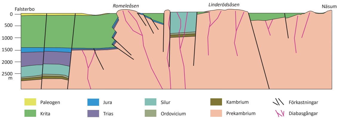
Figur 12. Ett tvärsnitt genom Skåne, från Falsterbo i sydväst till Näsium i nordost, visar hur berggrunden är uppdelad i block som rört sig i vertikalled.
