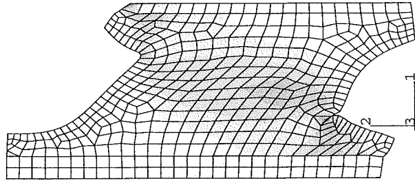
Figur 6: Töjningsenergis fördelning.
