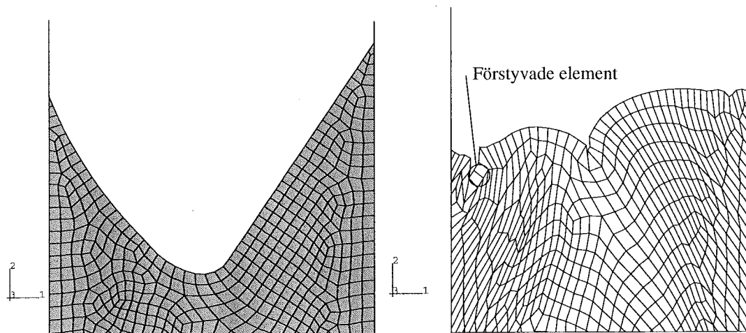
Figur 19: Asymmetriskt förslag nummer 5. Till vänster innan kompression och till höger vid full kompression \Delta r = 3.38mm .
