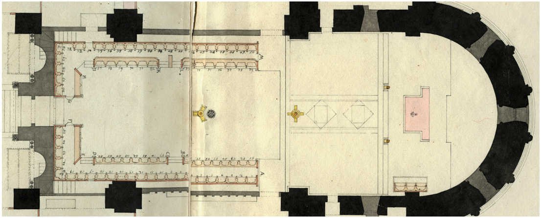
Figur 14. Högkorets planlösning 1833. Ritning av Axel Nyström. Källa: DM.
