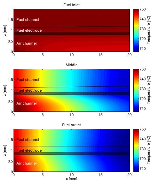
(d) T with thermal insulation
