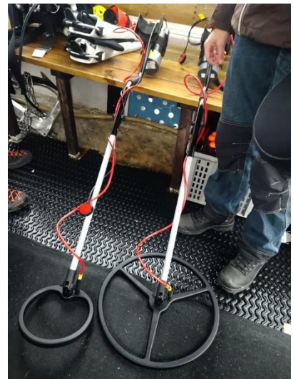
Figur 6 Aquascan AQ1B metalldetektorer. Foto: B. Foley.
