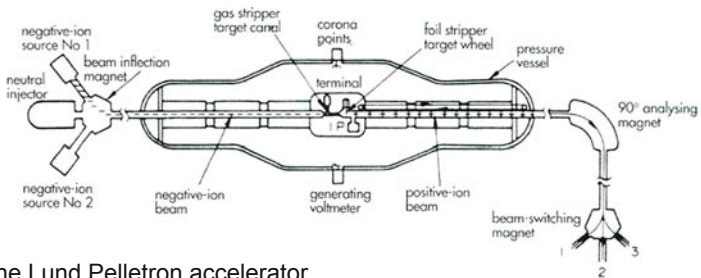
The Lund Pelletron accelerator.
