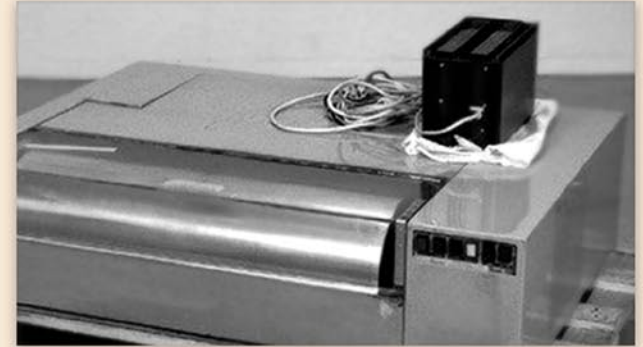
Hellmuth Hertz' inkjet printer. Prototyp. TM40522.
