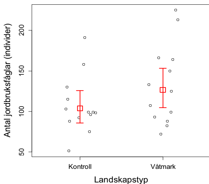
Figur 3. Effekten förekomsten av anlagd våtmark på antalet jordbruksfåglar i ett landskap med 1 km radie. Fyrkanterna visar modellresultatet och ringarna är data.
