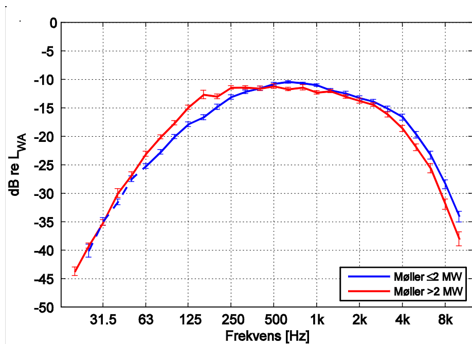
Figur 4. Normerede A-vægtede lydeffektniveauer i 1/3-oktavnånd. Middelvårdier for to grupper af mller: \leq 2 MW og > 2 MW. Lodrette streger angiver \pm 1 standard error of mean (s.e.m.).
