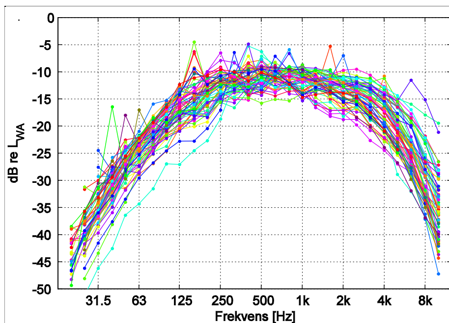
Figur 3. Normerede A-vægtede lydeffektniveauer i 1/3-oktavnband. 62 møller med nominel elektrisk effekt mellem 75 kW og 3,6 MW. (Normeret svarer til, at L_{WA} for den individuelle mølle er trukket fra alle niveauerne i 1/3-oktavnband).
