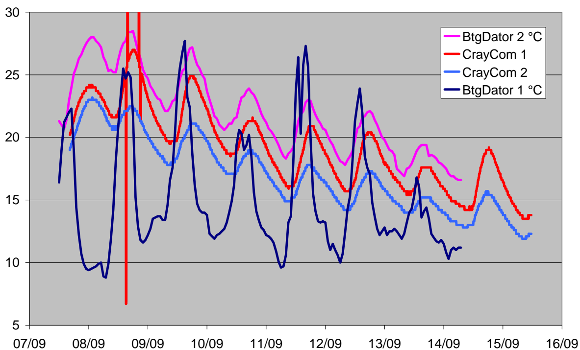
Figur 53. Jämförande mätvärden från BetongDatorn och CrayCom.
