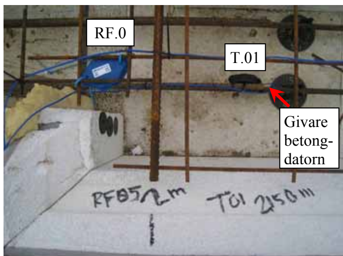
Figur 19. Placering av RF.05, T.01 samt betongdator
