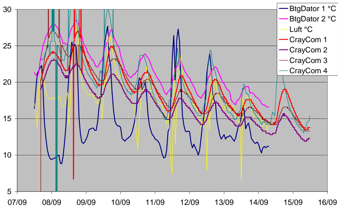
Figur 52. Samtliga mätvärden från BetongDatorn och CrayCom.
