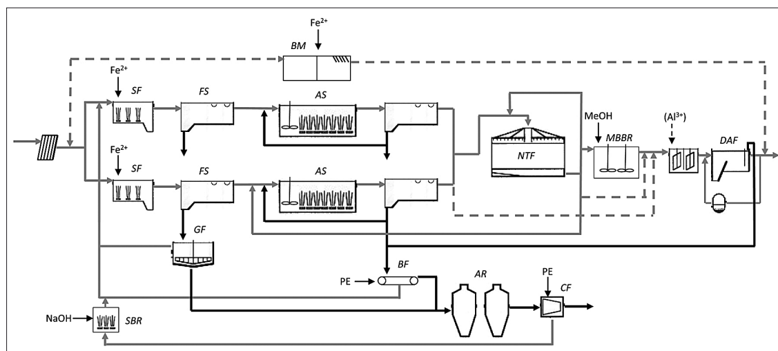
Figur 3. Dagens processkonfiguration på Sjölunda avloppsreningsverk. SF = sandfång, FS = försedimentering, AS = aktivt slamanläggning, NTF = nitritifierande biobädd, MBBR = Moving Bed Biofilm Reactor, DAF = flotation, GF = gravitationsförtjockare, BF = bandgravitationsförtjockare, AR = anaerob rötningsbassäng, CF = centrifuger, SBR = satsvis reaktor och BM = bräddvattenmagasin.
