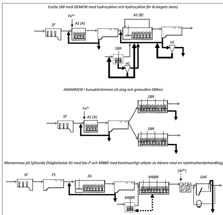
Figur 4. Tre olika processlösningar för implementering av anammox i huvudströmmen på kommunala avloppsreningsverk. SF = sandfång, FS = försedimentering, AS = aktivt slam, AS (A) = A-steg, AS (B) = B-steg, MBBR = Moving Bed Biofilm Reactor, DAF = flotation, SBR = satsvis reaktor och HC = hydrocyklon.
