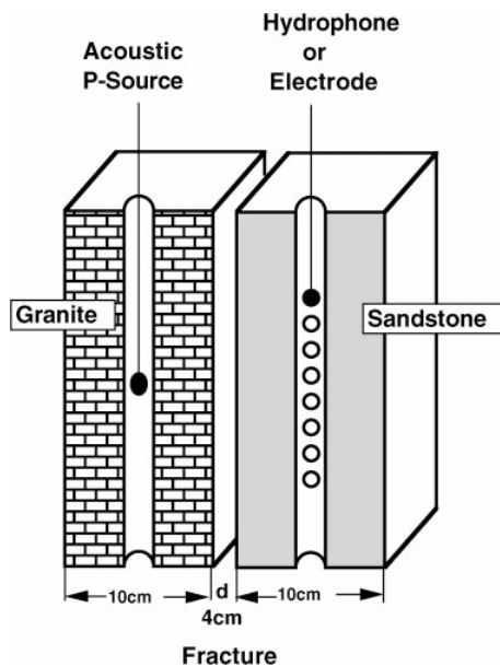
Figur 8.12. Försök med spricka mellan granit och sandstensytor (Zhu och Töksöz 2003) Test with a varying fracture width between granite and sandstone.
