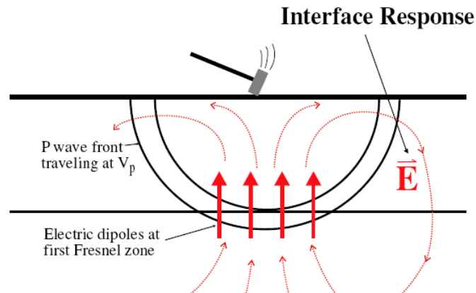
Figur 8.14. Det elektriska fältet (röda linjer) kring en vertikal dipol (röda pilar) The electric field (red lines) around a vertical dipole (red arrows)
