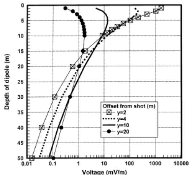
Figur 8.7. Det kring skottpunkten radiella elektriska fältets variation med djupet till en vertikal dipol med enhetsmoment 1 \text{ Am}^3 (produkten av ström och volym). Around the shotpoint radial field dependence of depth to a vertical dipole with unity moment 1 \text{ Am}^3 (product of current and volume)
