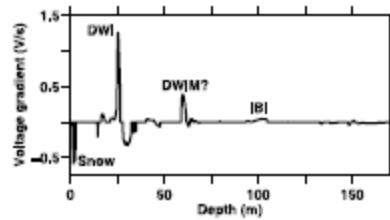
Figur 8.16. Seismoelektriska registreringar på glaciär med dubbelreflex vid 58 m.
