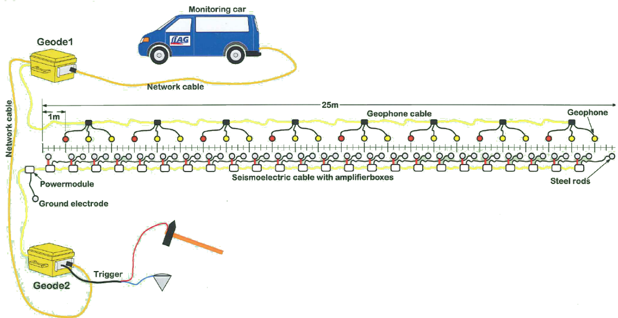
Figur 5.1. Principskiss för mätupställning för samtidig mätning av seismiska och seismo-elektriska signaler (Grüneberg 2011).
