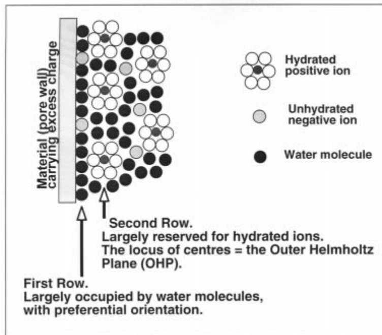
Figure 8.5. Principiell uppbyggnad av det elektriska dubbellagret nära en mineralyta. The structure of the electric double layer near a mineral surface.
